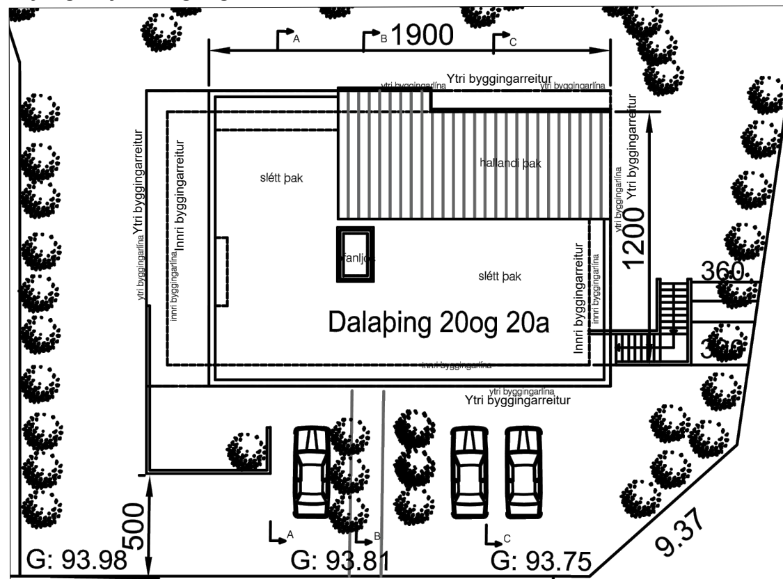
Skýringarmynd: afstöðumynd í mkv. 1:250
