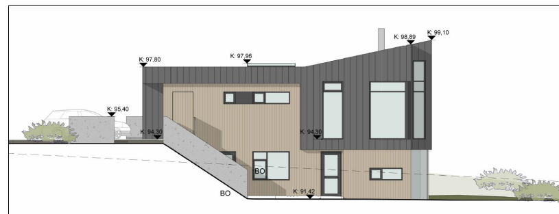
Skýringarmynd: mögulegt útlit vestur í mkv. 1:250
