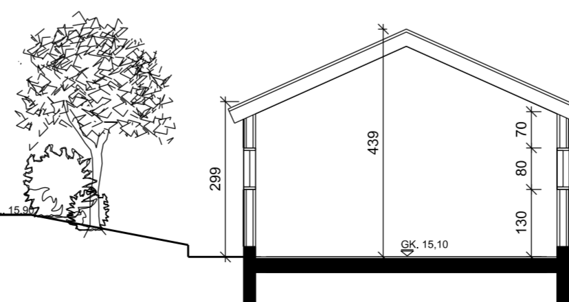
SNIDMYND
