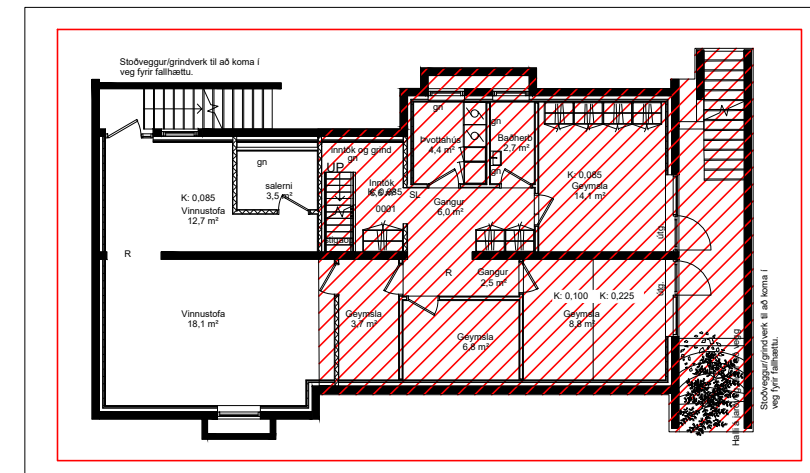
Skýringarmynd: Grunnmynd kjallara tillaga að breytingu mkv. 1:200
