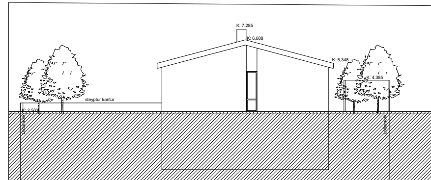
Skýringarmynd: Núverandi útliti kjallara suðurhlíð í mkv. 1:200
