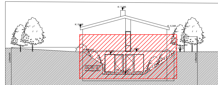
Skýringarmynd: Tillaga að breyting á útliti kjallara suðurhlíð í mkv. 1:200 Stoðveggur upp færður og útitróppur. Nýjir gluggar og hurðar.
