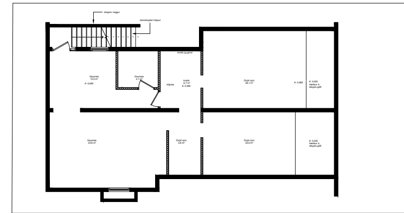
Skýringarmynd: Grunnmynd kjallara mkv. 1:200
