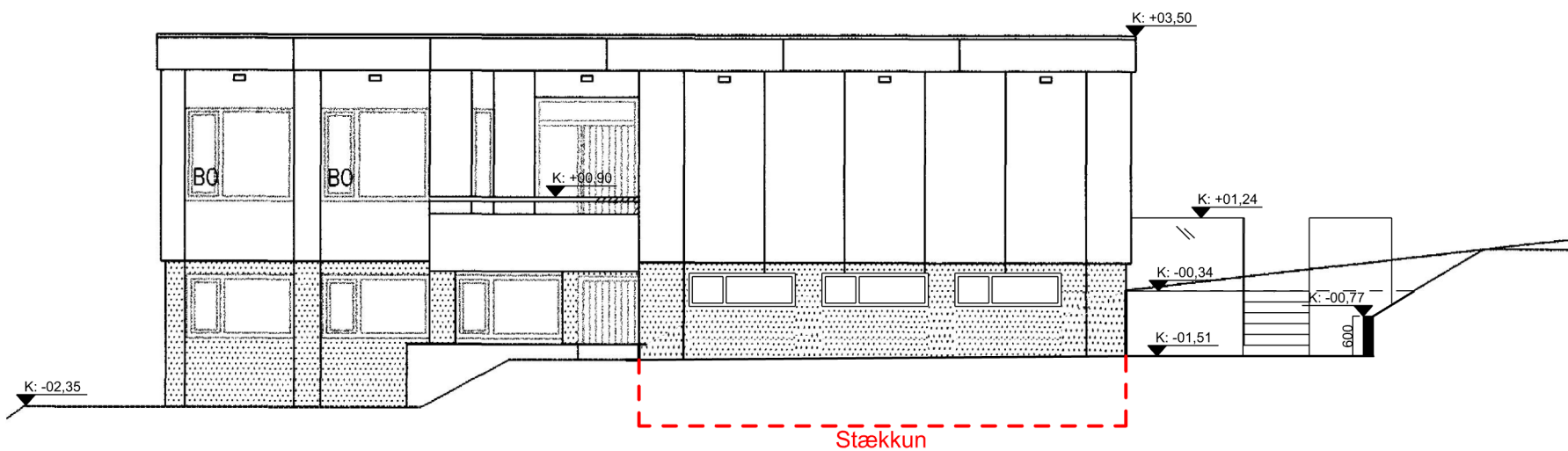
AUSTUR 1:100
