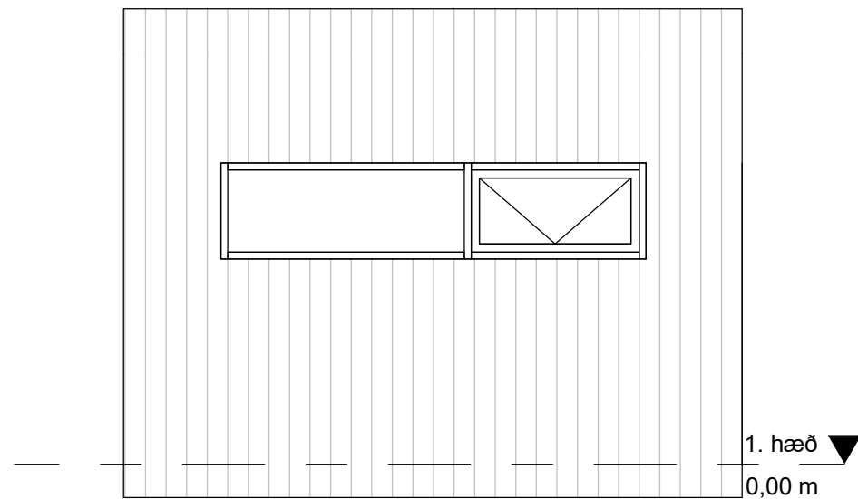
6 Vestur 1 : 50
