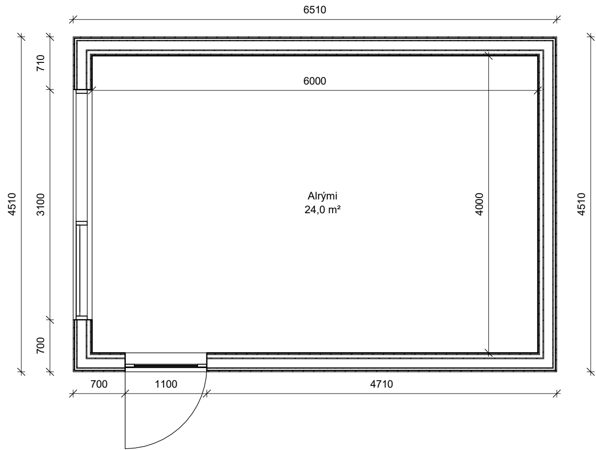
1 Grunnmynd 1 : 50
