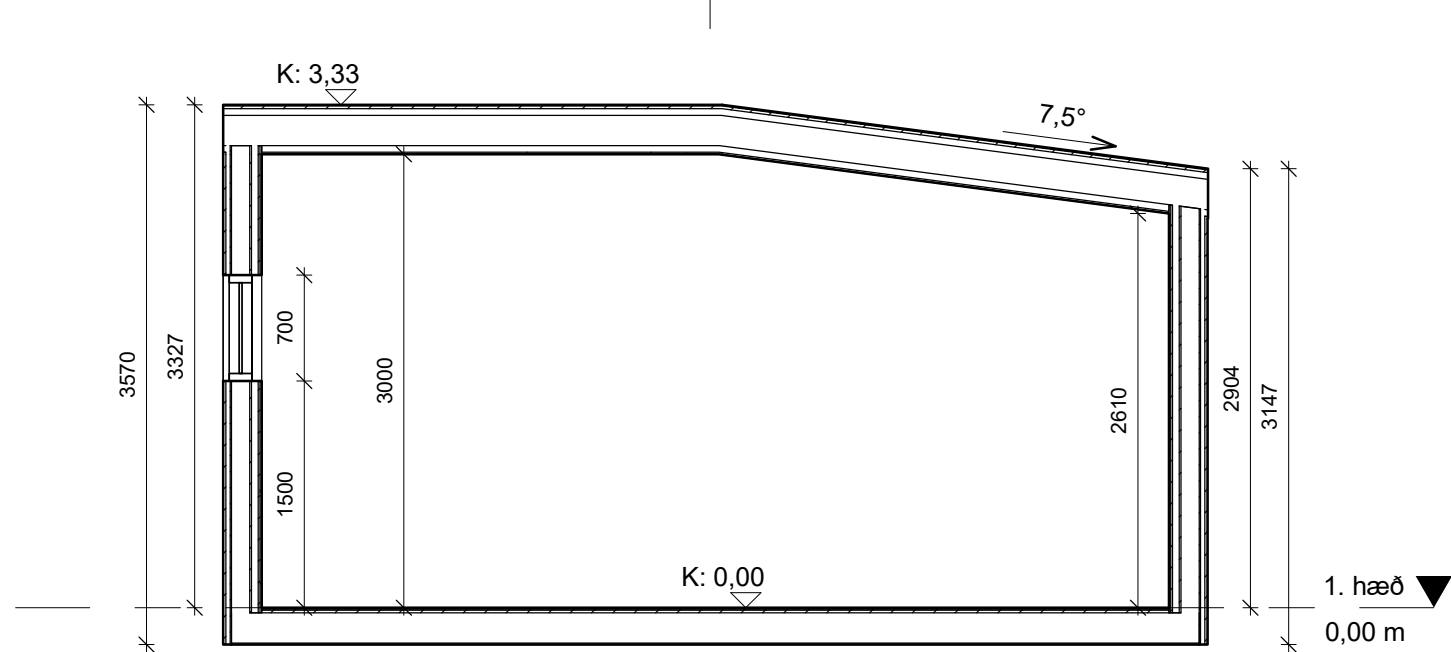
8 Snið. 1 : 50
