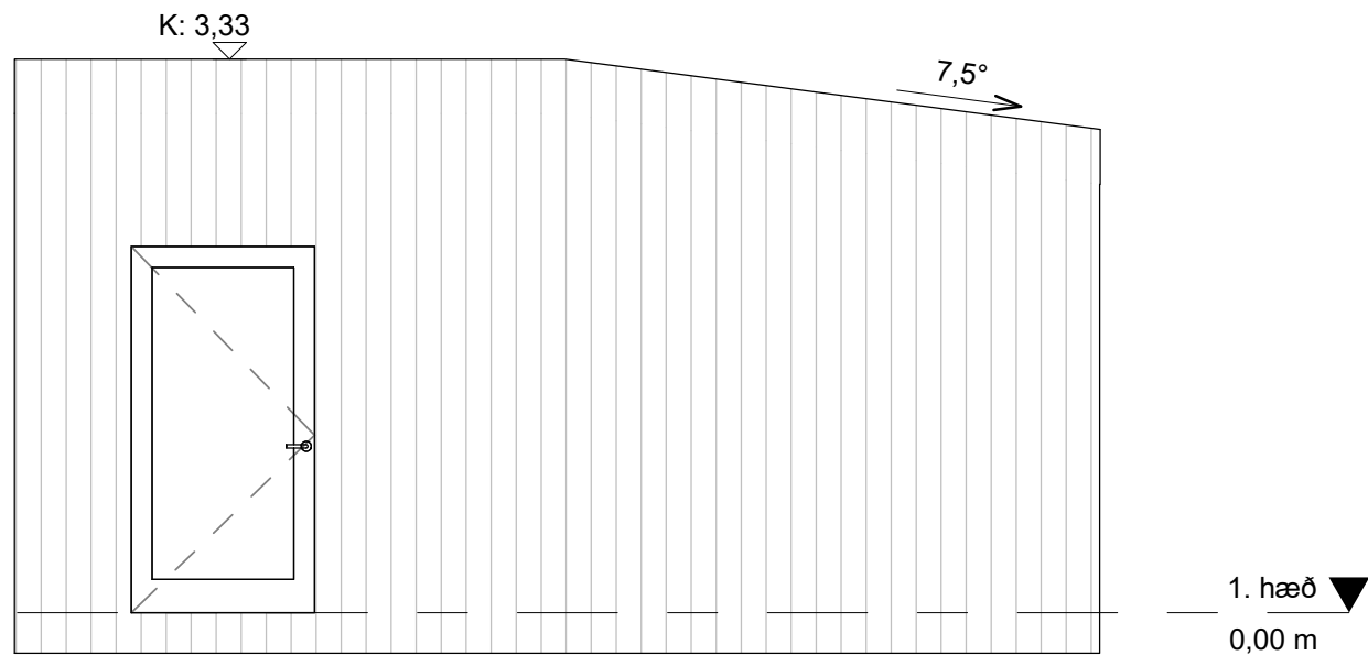
5 Suður 1 : 50
