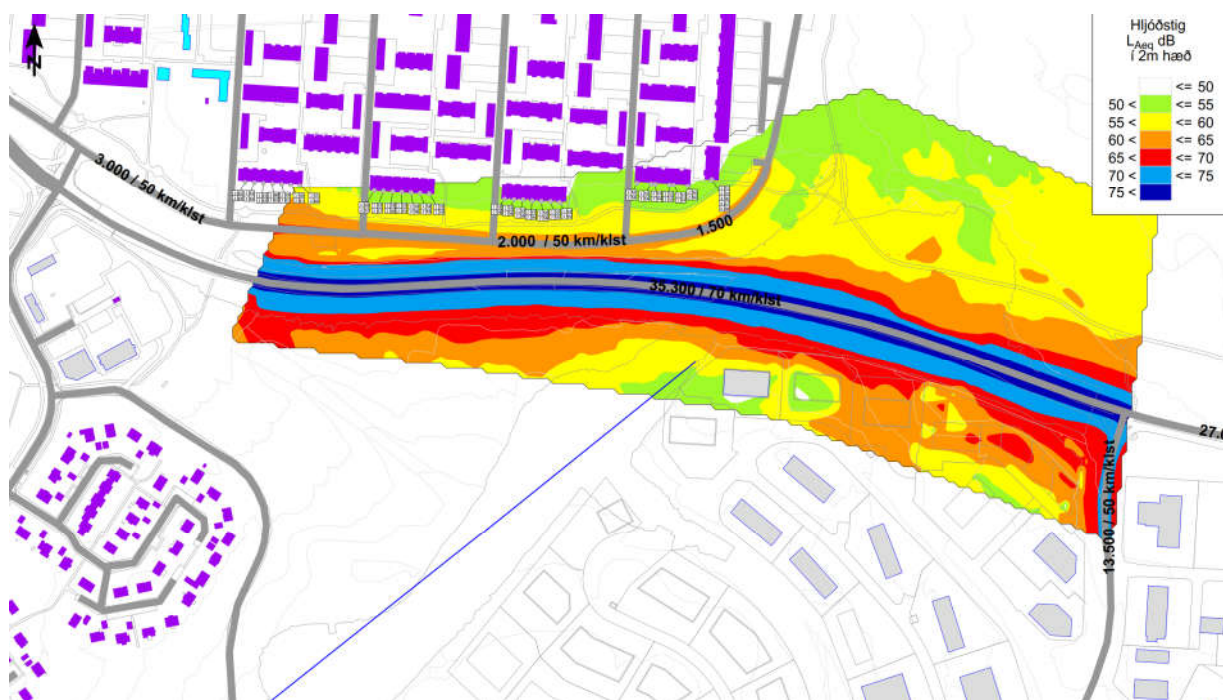
MYND 4 Yfirlitsmyndin sýnir núverandi gatnakerfi og hljóðstig í 2m hæð, miðan við umferðarspá fyrir árið 2030, alls 33.300 bíla á klst með hámarkshraða 70 km/klst á Breiðholtsbraut (EFLA, 2020).
