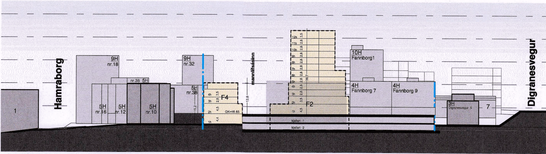
SKILMÁLASNEIÐING D-D FANNBORG
