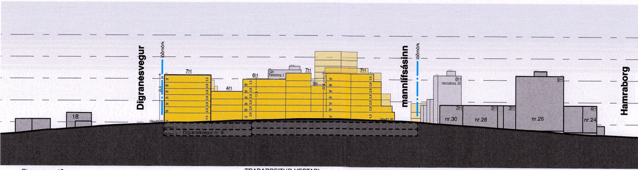
SKILMÁLASNEIÐING A-A VALLARTRÖÐ
