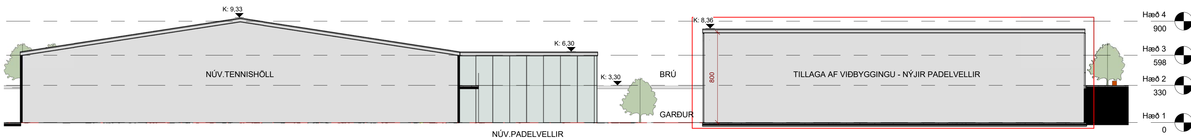
6 SNIÐ 1 - Í GEGNUM PADELVELLI OG GARÐ Á MILLI HÚSA 1 : 200
