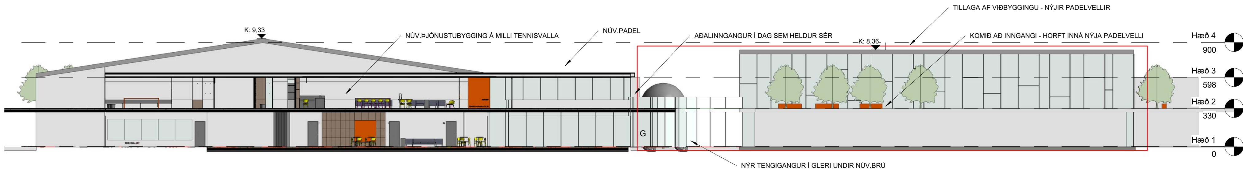
1 SNIÐ 2 - AÐKOMA - TENGIGANGUR 1 : 200
