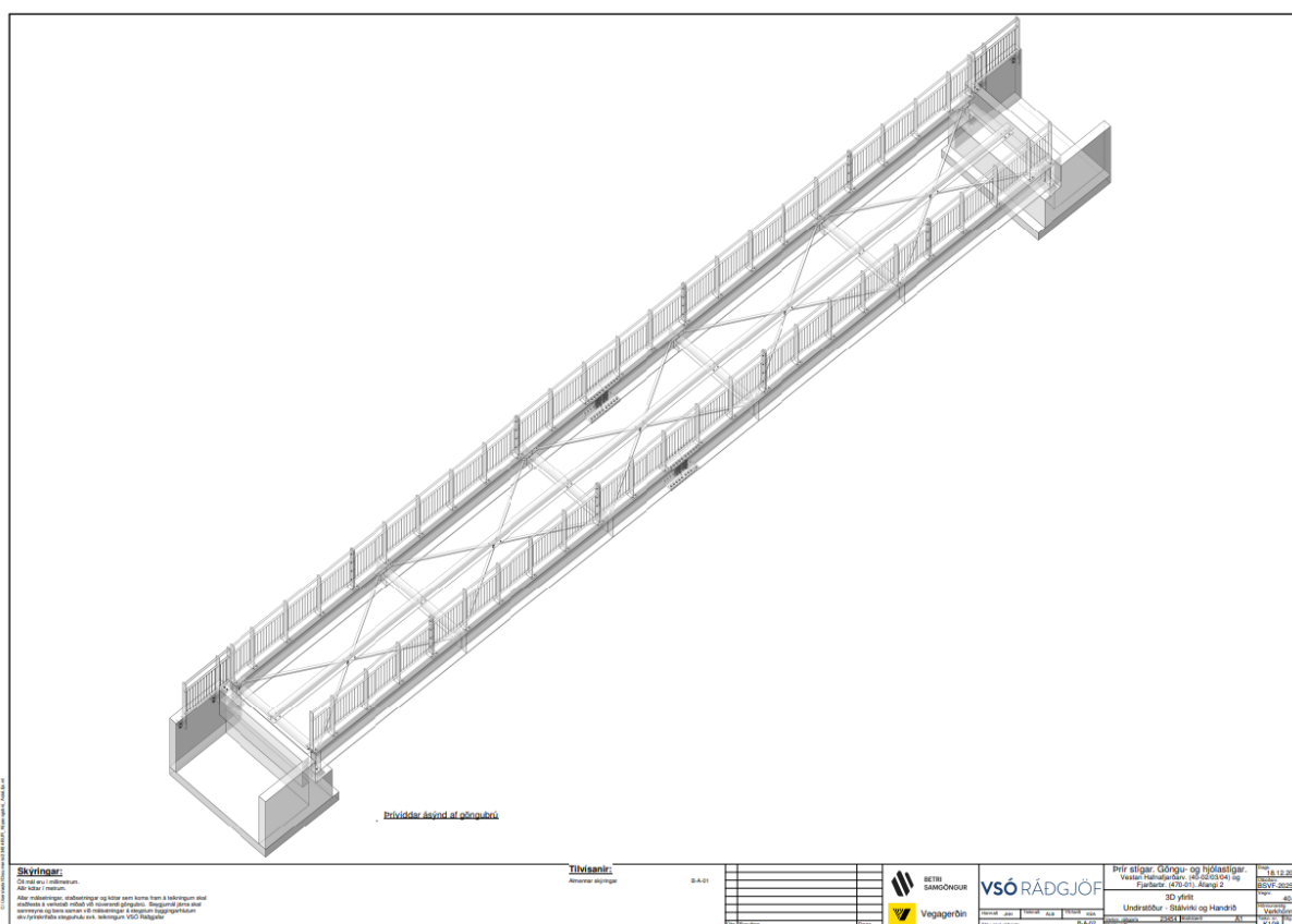
Mynd 8. Þrívíddar ásynd af göngubrú.
