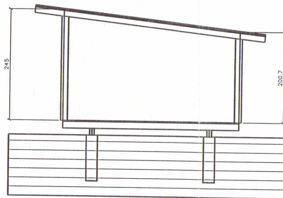
SNID GEGNUM HERBERGI
