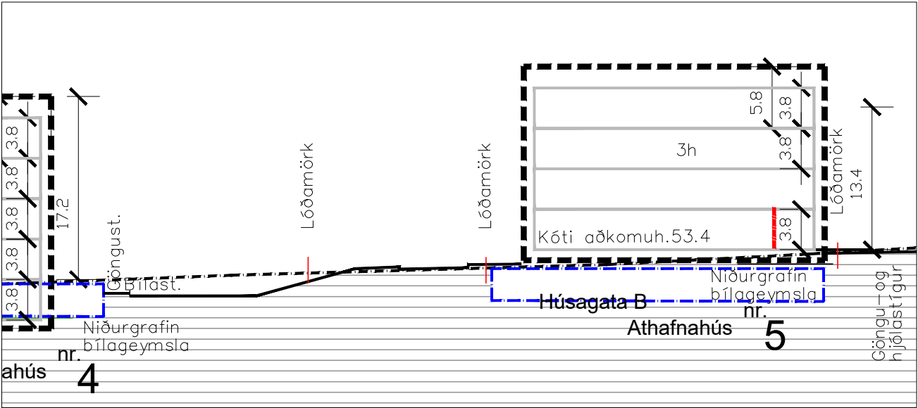
Sneiðing 1-0D í mkv. 1:500
