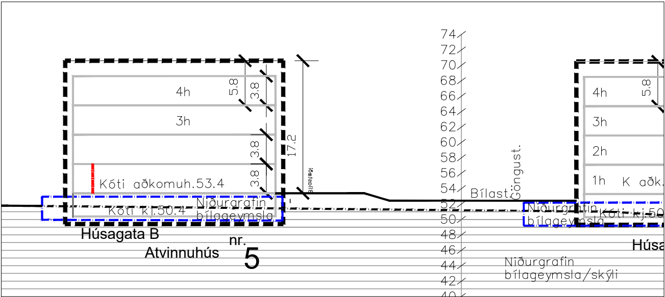
Sneiðing 1-0B í mkv. 1:500
