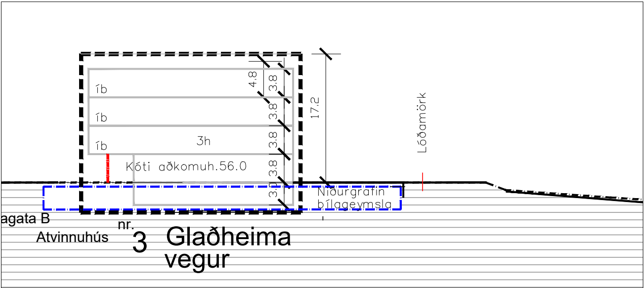
Sneiðing 1-0C í mkv. 1:500
