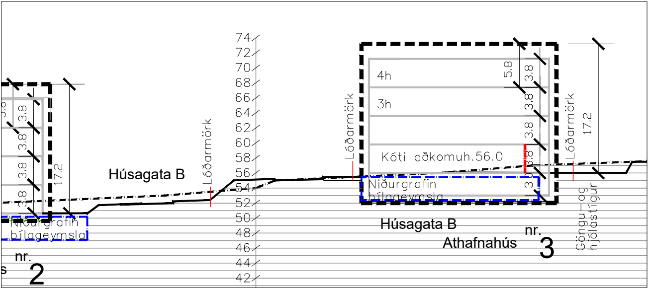
Sneiðing 1-0E í mkv. 1:500
