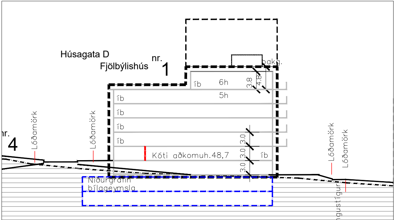
Sneiðing 2-0F í mkv. 1:500
