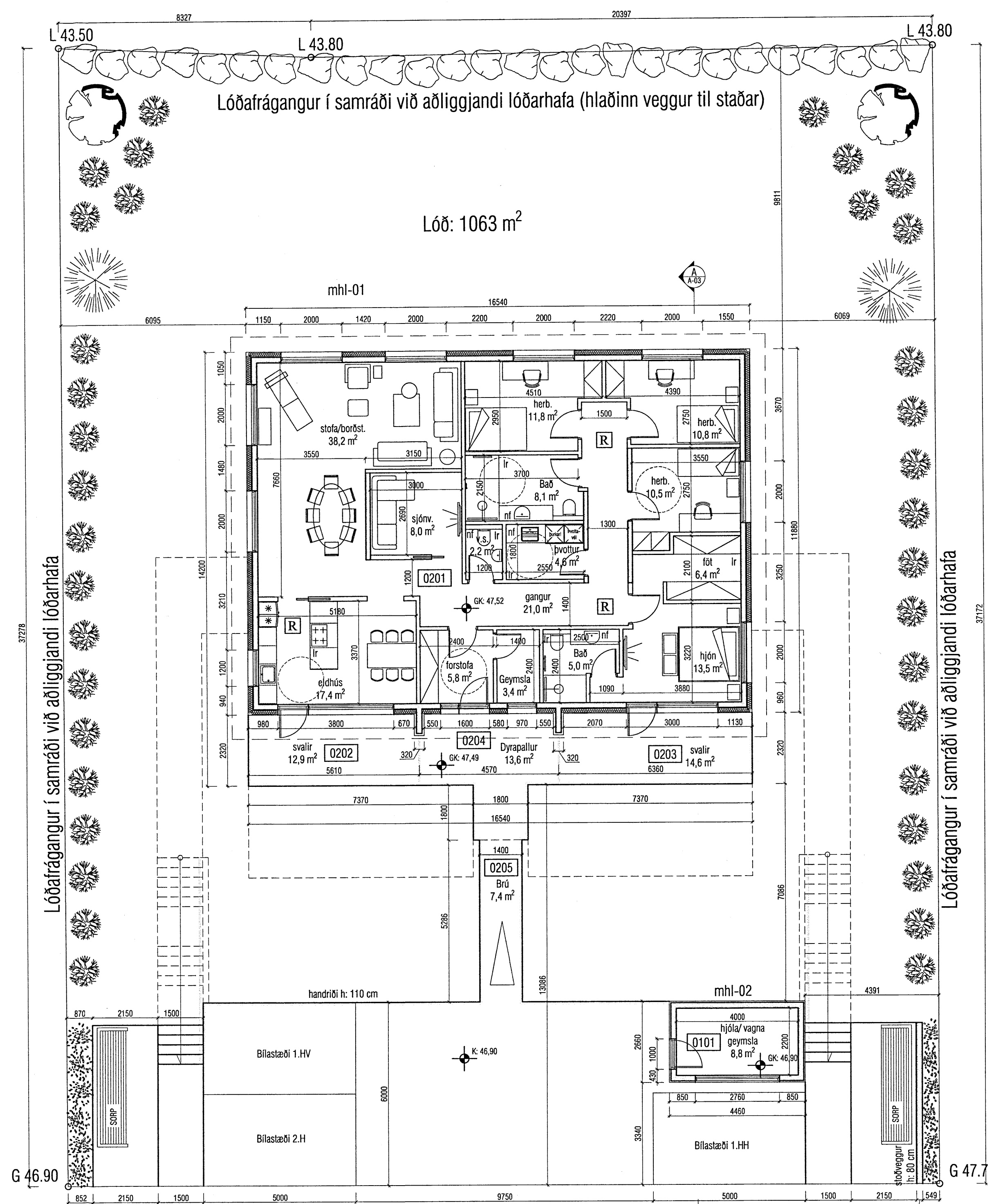
Grunnmynd 2.hæð
