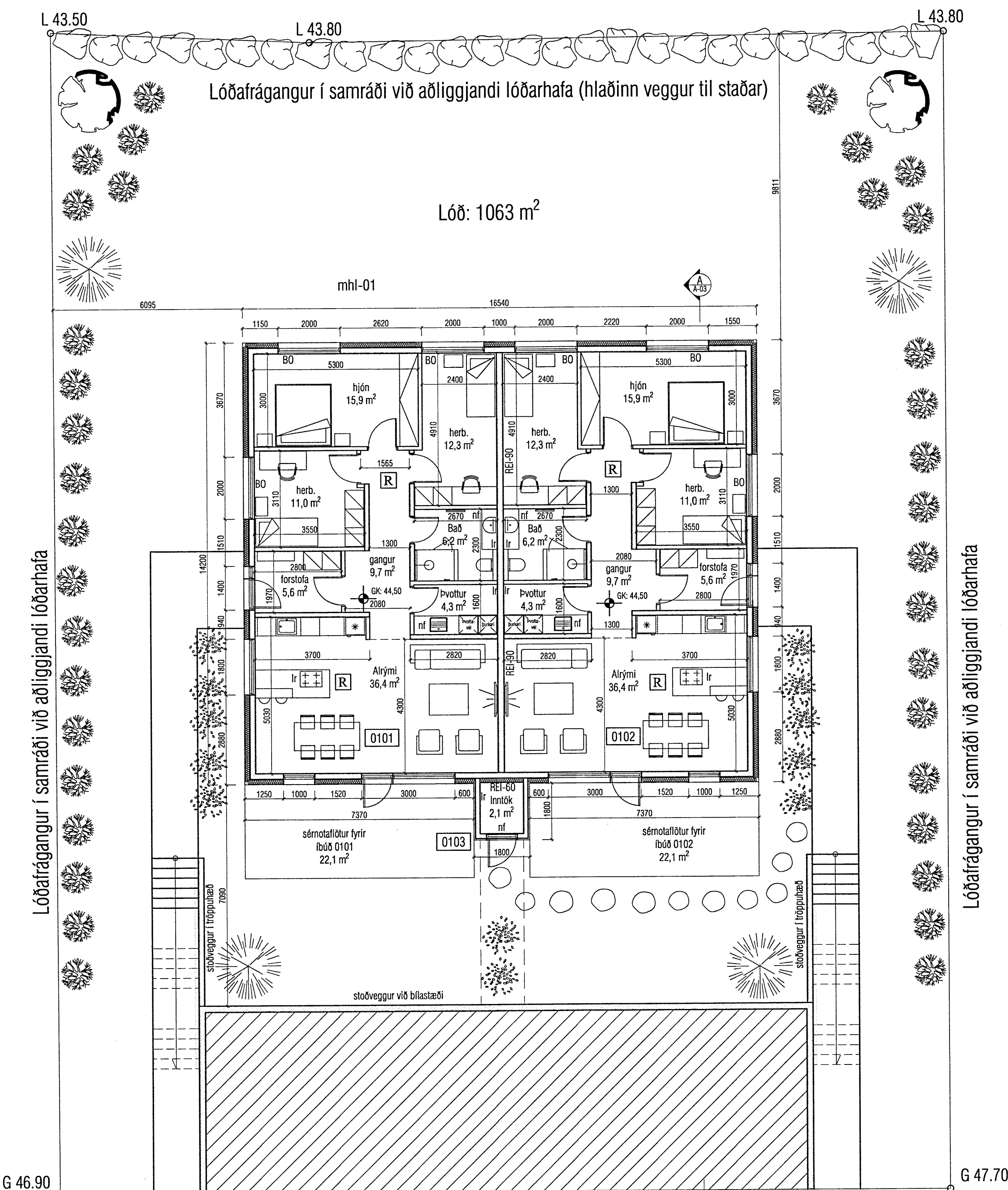
Grunnmynd 1.hæð
