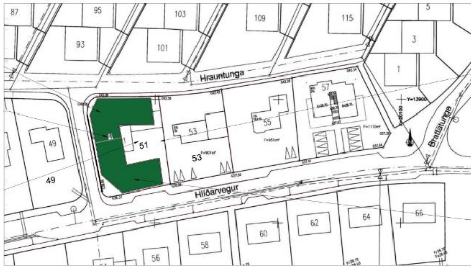
AFSTÖÐUMYND 1:500
