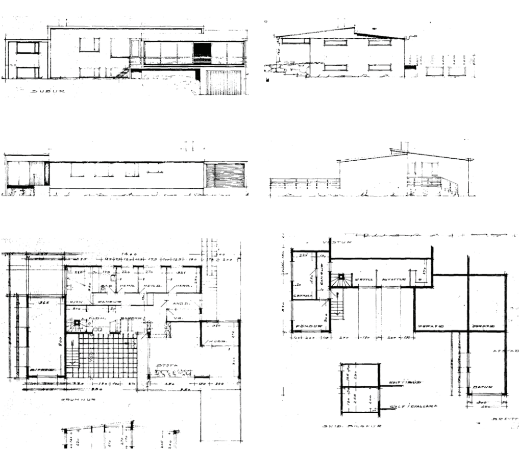
Mynd 114: Grunnmyndir og ásyndir.
