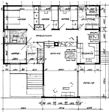
Mynd 101: Kastalagerði 11. Grunnmyndir og ásýndir
