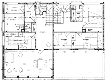
Mynd 90: Skólagerði 19-21. Grunnmynd og ásýndir
