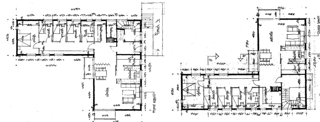
Mynd 91: Kársnesbraut 47. Grunnmynd og ásýndir
