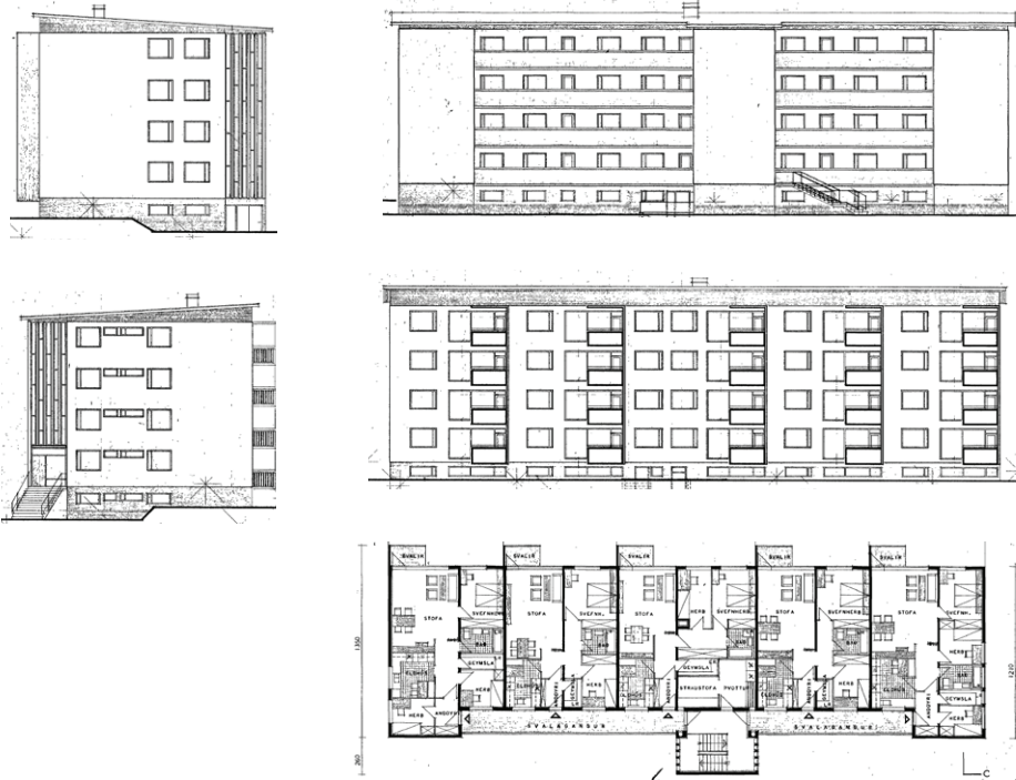
Mynd 89: Ásbraut 15-17. Grunnmynd og ásyndir
