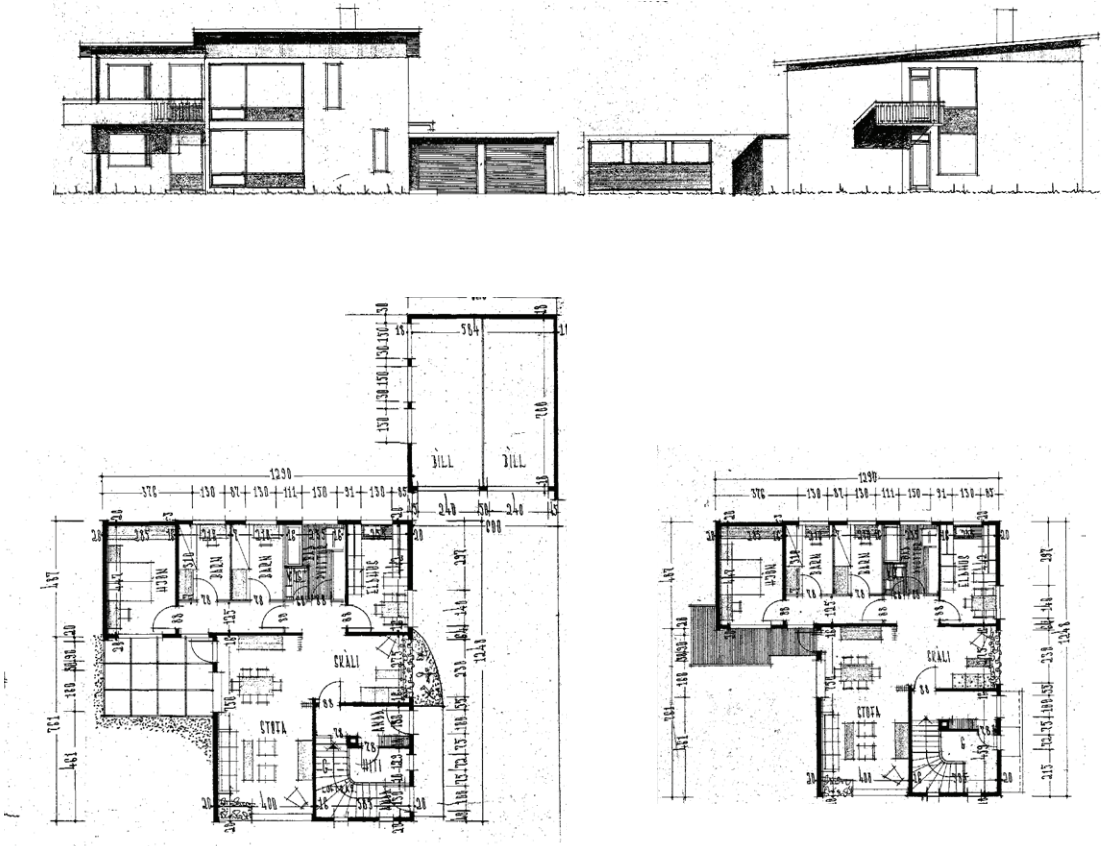
Mynd 93: Holtagerði 50. Grunnmyndir og ásýndir.
