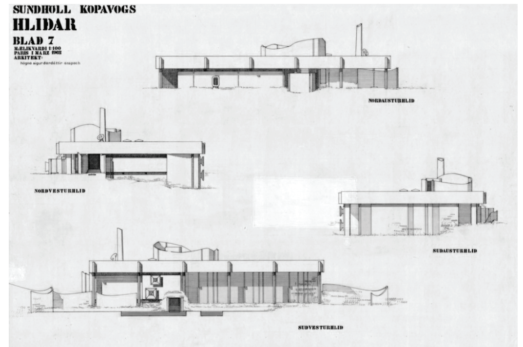
Mynd 78: Tillaga að útliti sundlaugarinnar, 1962.
