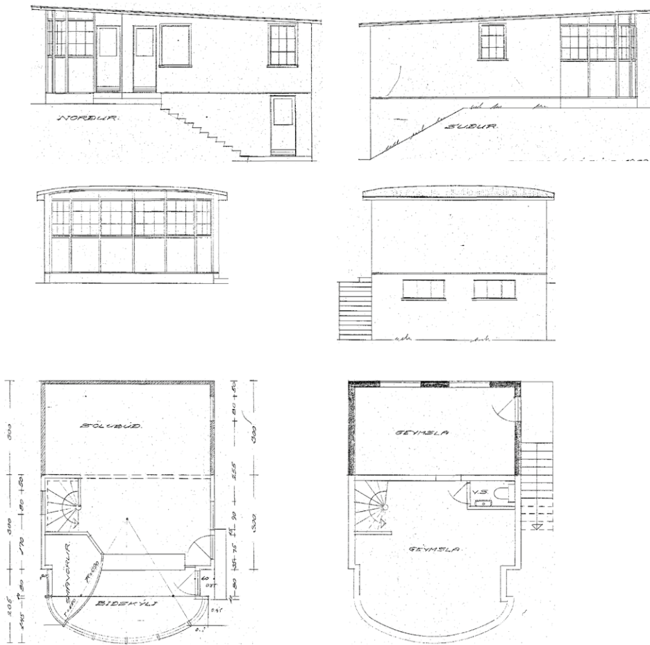
Mynd 65: Ásýndir. Aðaluppdráttur fyrir Kópavogsbraut 115, 1955.
