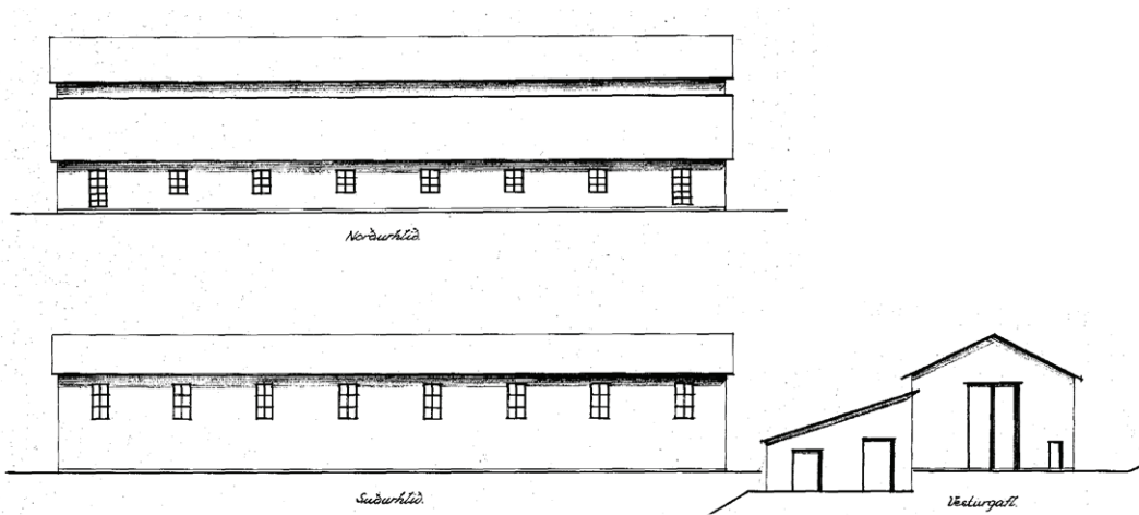
Mynd 64: Ásýndir. Aðaluppdráttur fyrir Kársnesbraut 58a, 1949.
