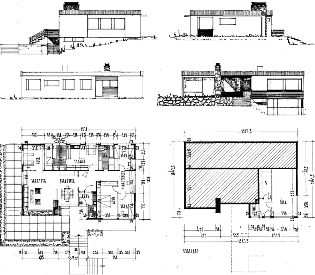
Mynd 108: Sunnubraut 34. Grunnmyndir og áskýndir.
