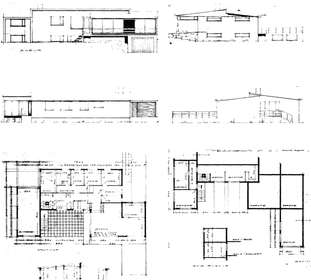
Mynd 113: Grunnmyndir og ásyndir.
