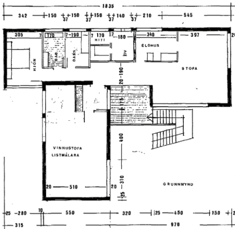
Mynd 100: Kastalagerði 13. Grunnmyndir og ásýndir
