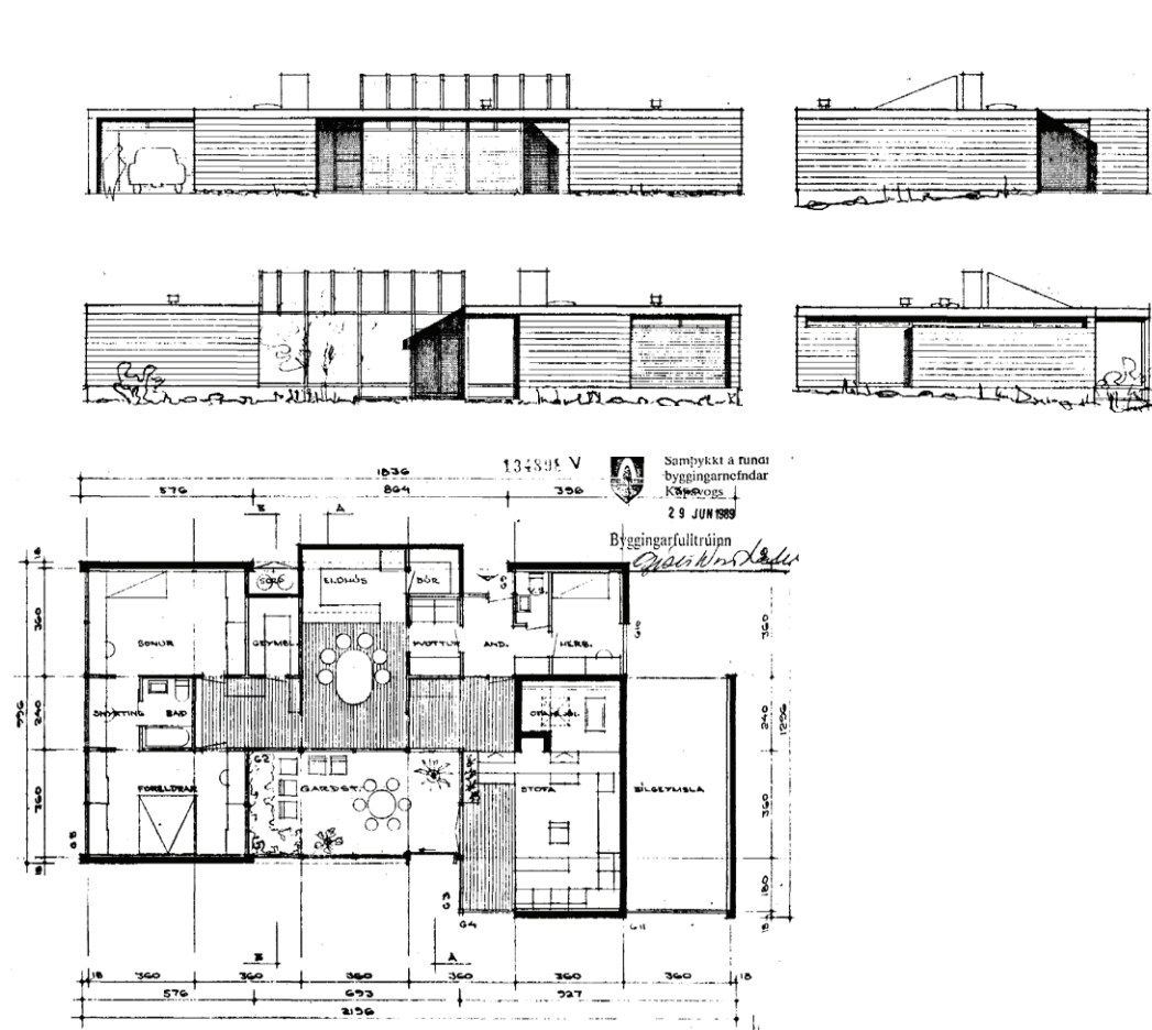
Mynd 112: Grunnmyndir og ásyndir.
