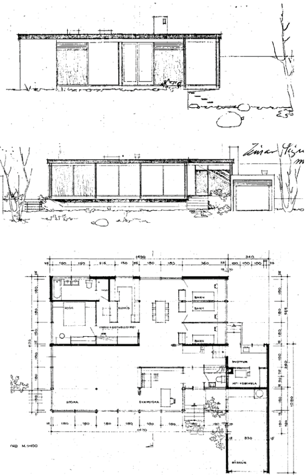
Mynd 110: Sunnubraut 6-10. Grunnmynd og ásýndir.
