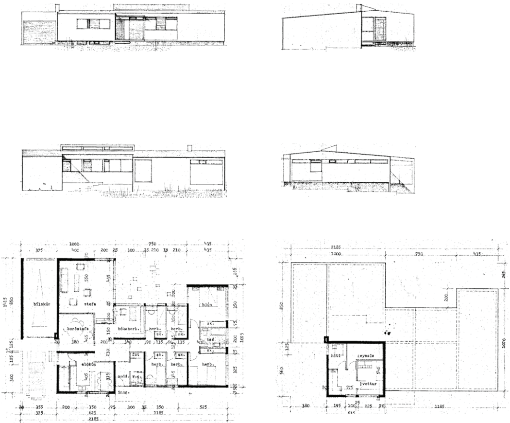
Mynd 111: Grunnmyndir og ásýndir.
