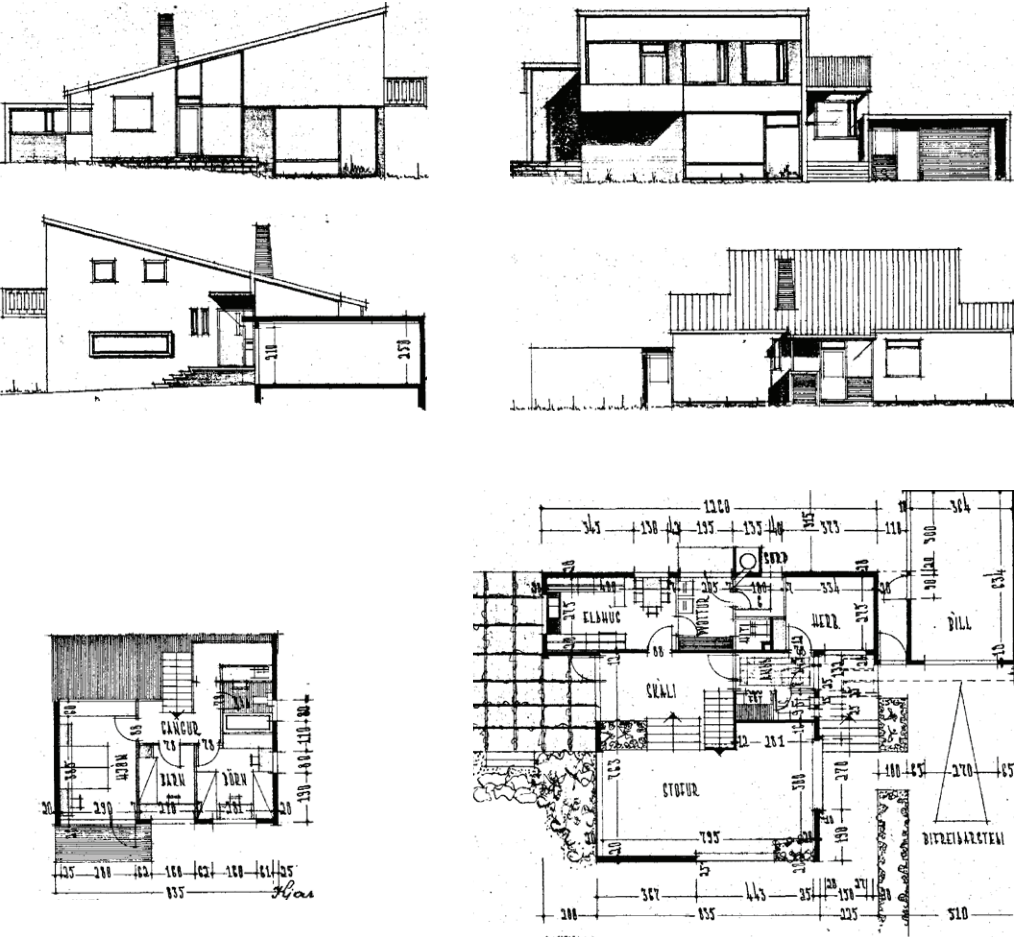
Mynd 109: Sunnubraut 40. Grunnmyndir og áskýndir.
