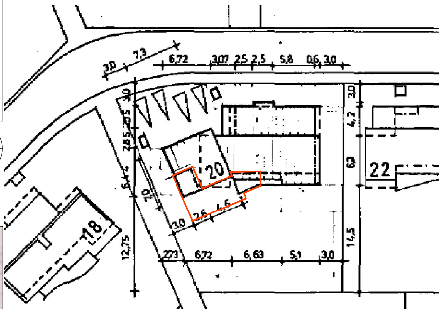
Núv. afstöðumynd mkv.1:500 og mörk kjallara eru sýnd með rauðri línu FAGRIHJALLI
