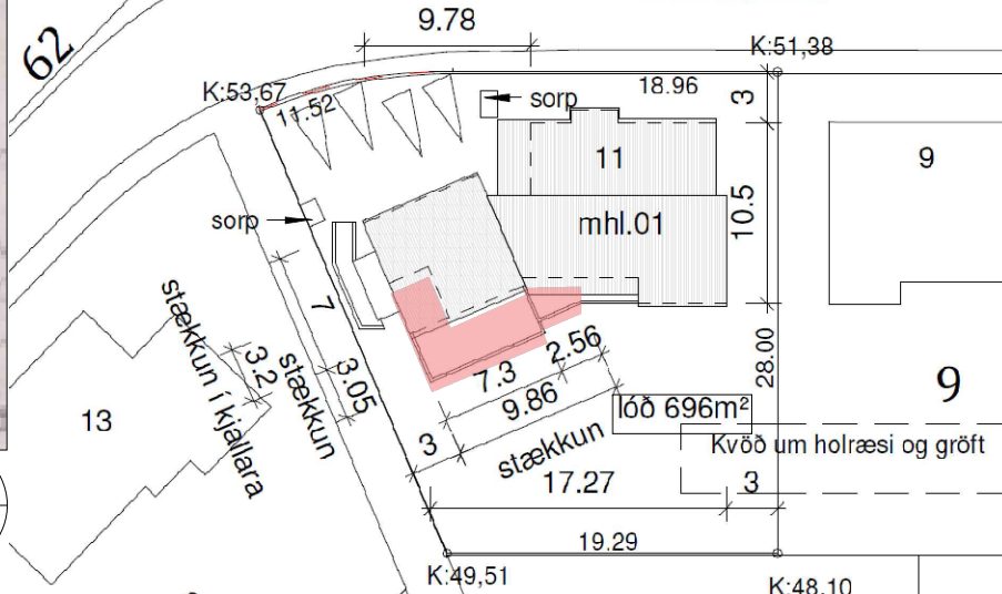
Breytt afstöðumynd mkv.1:500. Breyting. Stækkun byggingarreits kjallara.
