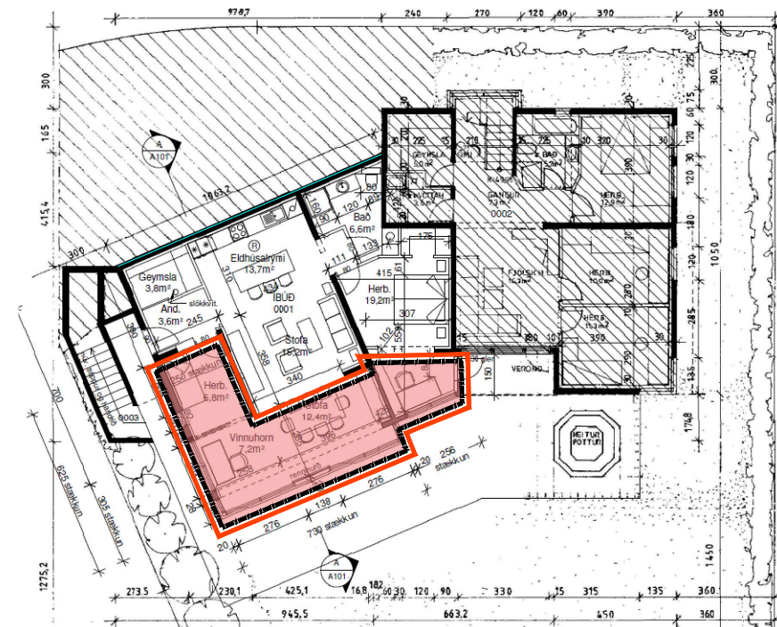
Breytt grunnmynd kjallara mkv.1:250. Neðri hæð íbúðar 0101 er skástrikuð helst óbreytt.
