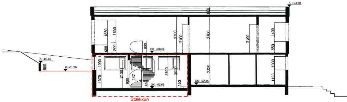
SNID B-B 1:100
