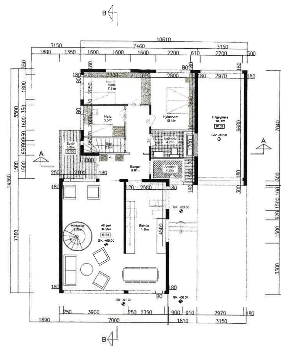
GRUNNMYND 1.HÆÐ 1:100
