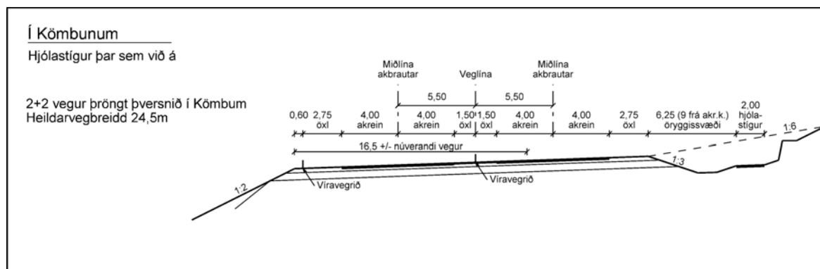
Mynd 3-10 Kennisnið Suðurlandsvegar í Kömbunum. Hjólastígur verður utan öryggissvæðis. Vegrið verður á milli akbrauta og á ytri vegöxl.
