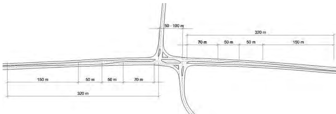
Mynd 3-13 Fyrirkomulag vegamóta þar sem tvenn T-vegamót mynda saman ein X-vegamót. Af öryggisástæðum er aðeins ein akrein í hvora átt í gegnum vegamótin.
