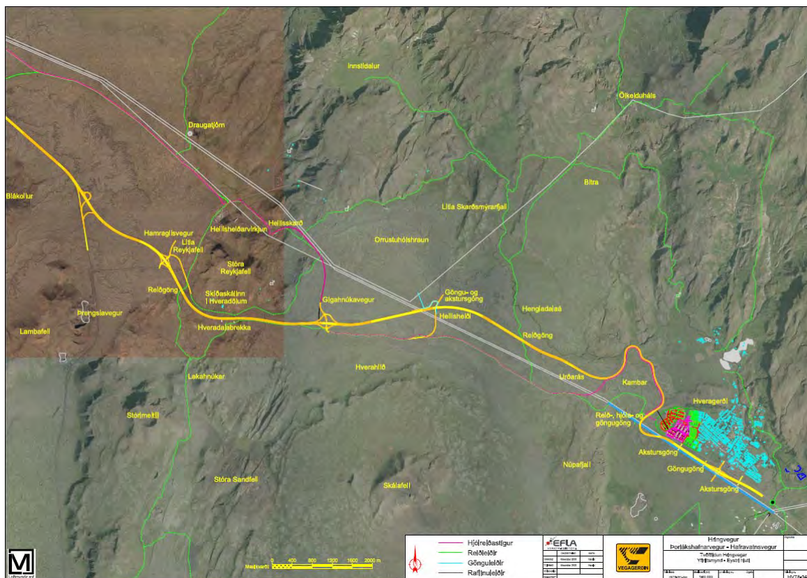
Mynd 3-19 Hjólréiðaleiðin mun liggja um Gígahnúkaveg og sunnan Suðurlandsvegur um þjónustuvegi Hverahlíðarvirkjunar, gamla þjóðveginn og með vegi í Kömbum (sjá stærra kort í viðauka 1).
