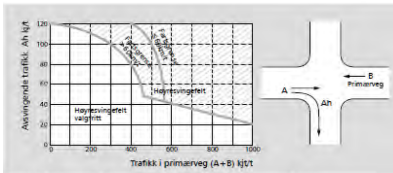
Figur 4.13: Høyresvingefelt i primærvæg basert på trafikk i dimensionerende time
