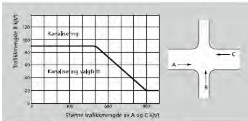
Figur 4.6: Trafíkkay í sekundærvæg basert på trafikken i dimensionerende time
