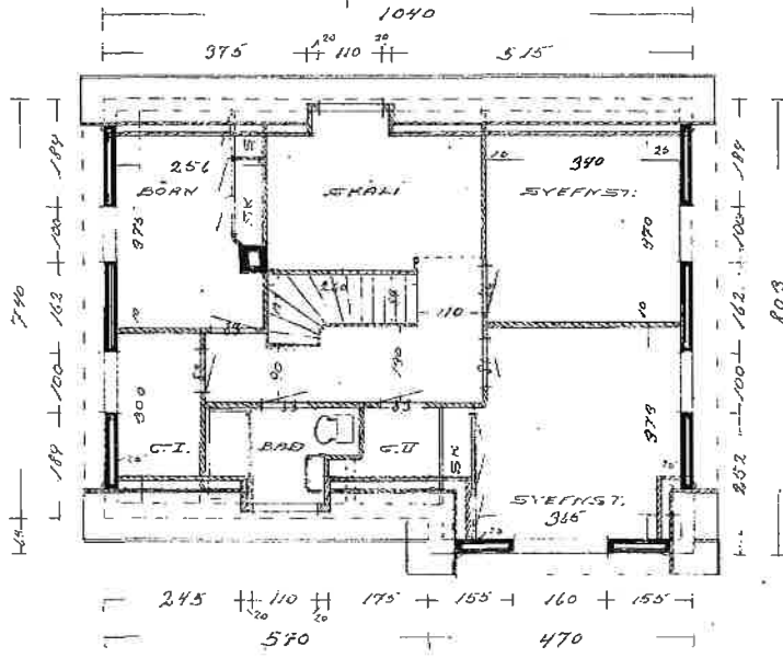
ÞAKHÆÐ
