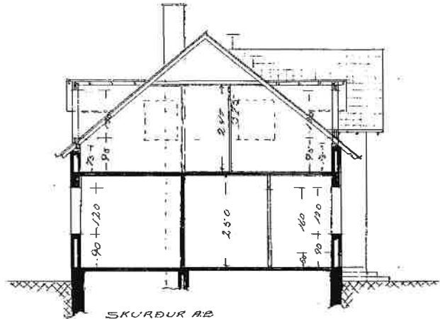
SKURÐUR A2
