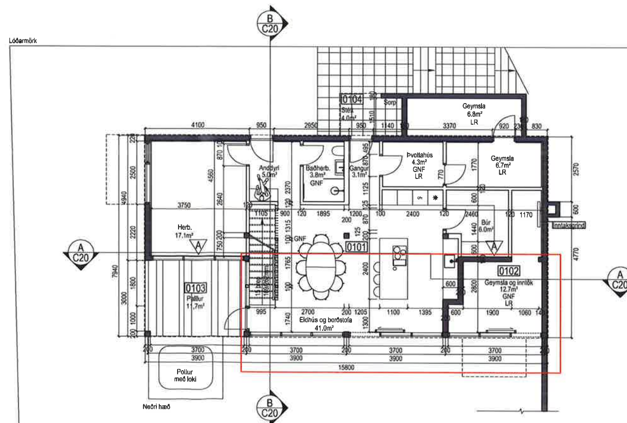
2. HÆÐ 1:100
