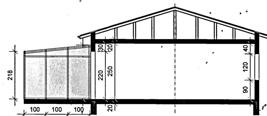
Snið D-D
