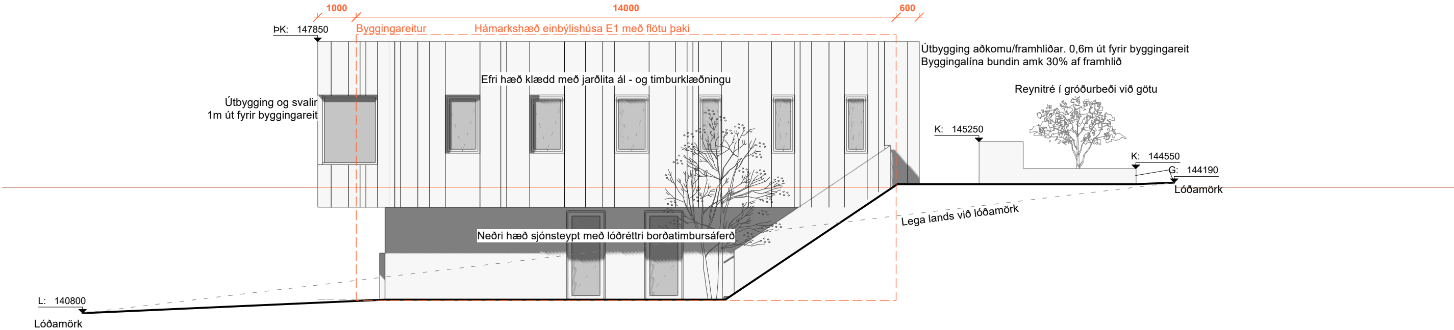
austurhlíð 1:100
