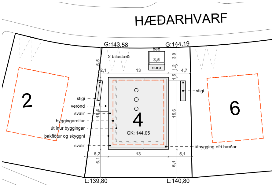
afstöðumynd 1:500
