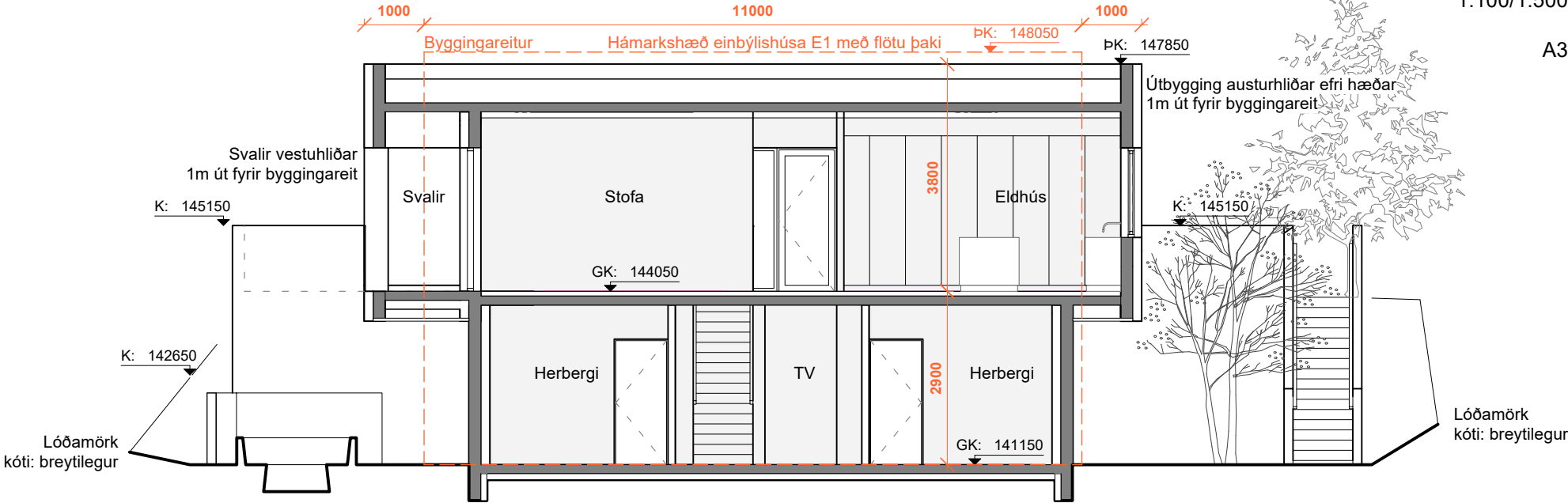
þversnið 1:100
