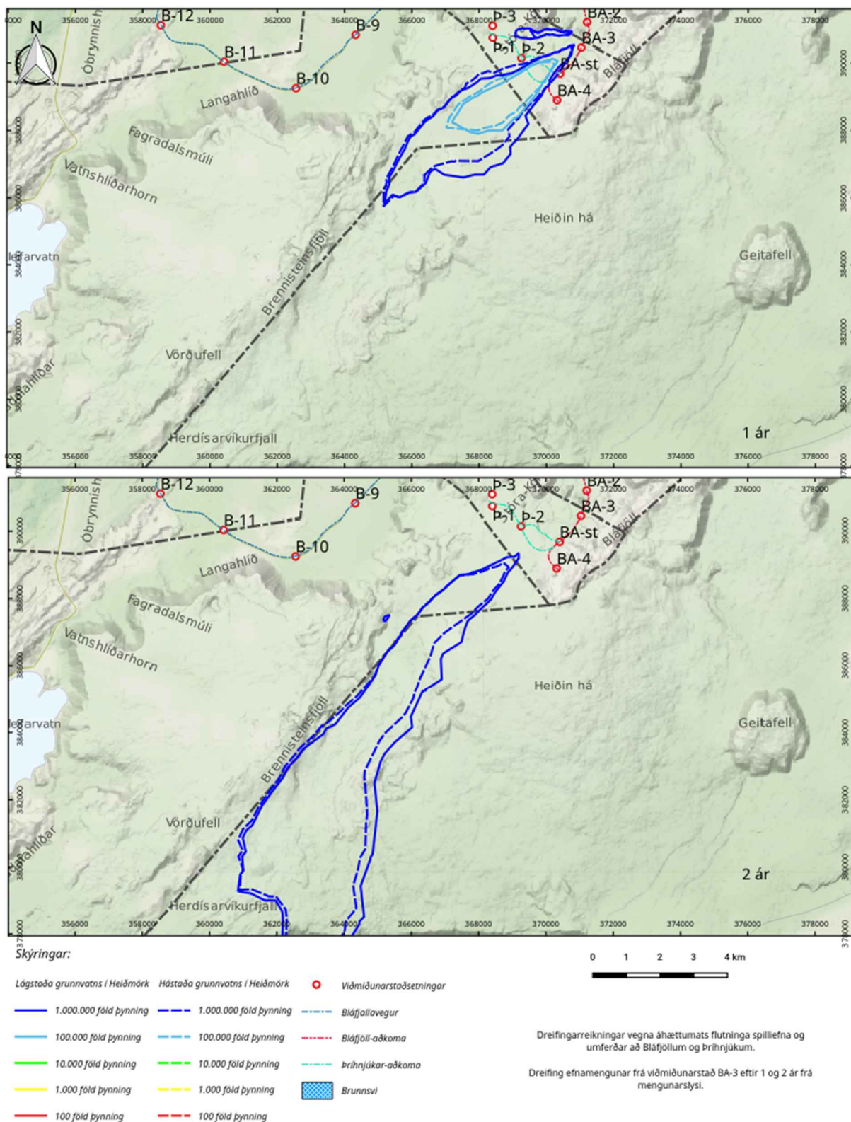
Mynd 68. Dreifing efnamengunar frá viðmiðunarstað BA-3 eftir 1 og 2 ár frá mengunarslysi.
