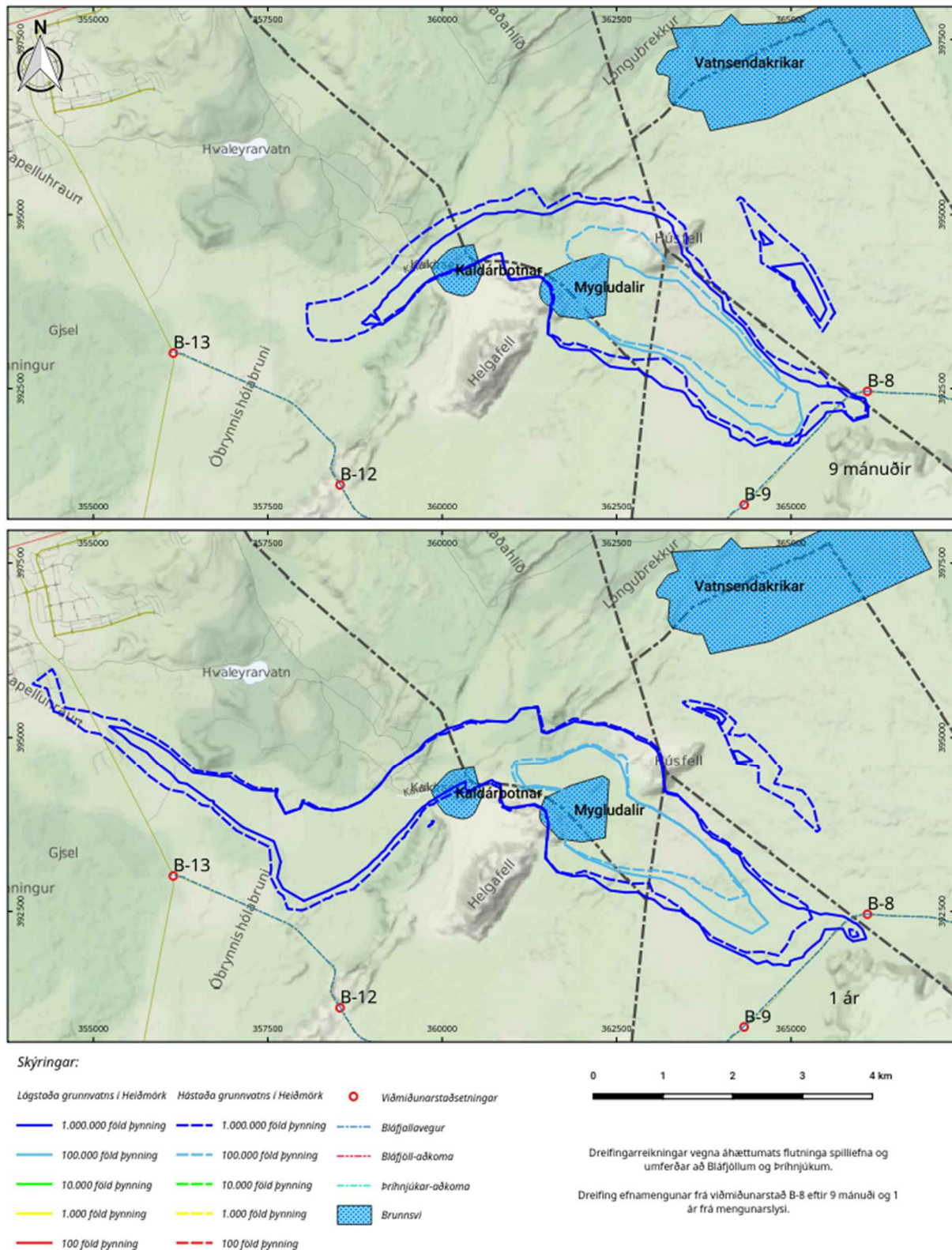
Mynd 37. Dreifing efnamengunar frá viðmiðunarstað B-8 eftir 9 mánuði og 1 ár frá mengunarslysi.
