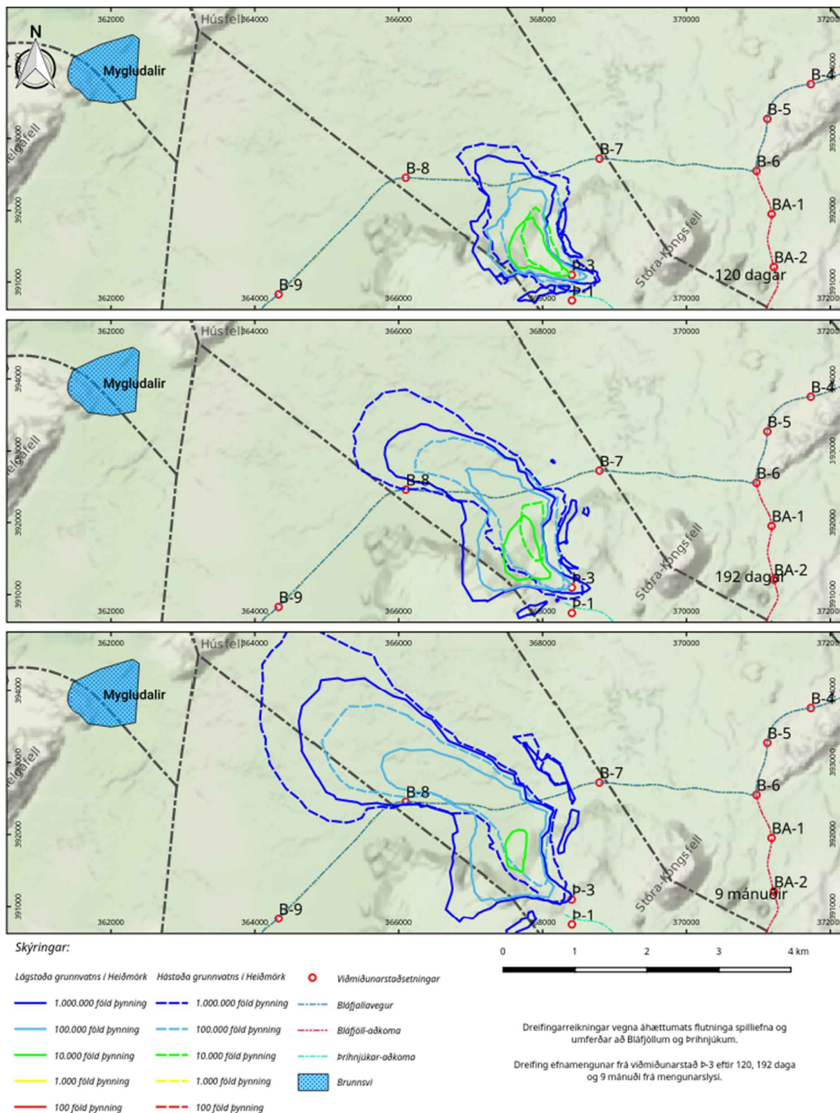
Mynd 90. Dreifing efnamengunar frá viðmiðunarstað P-3 eftir 120, 192 daga og 9 mánuði frá mengunarslysi.
