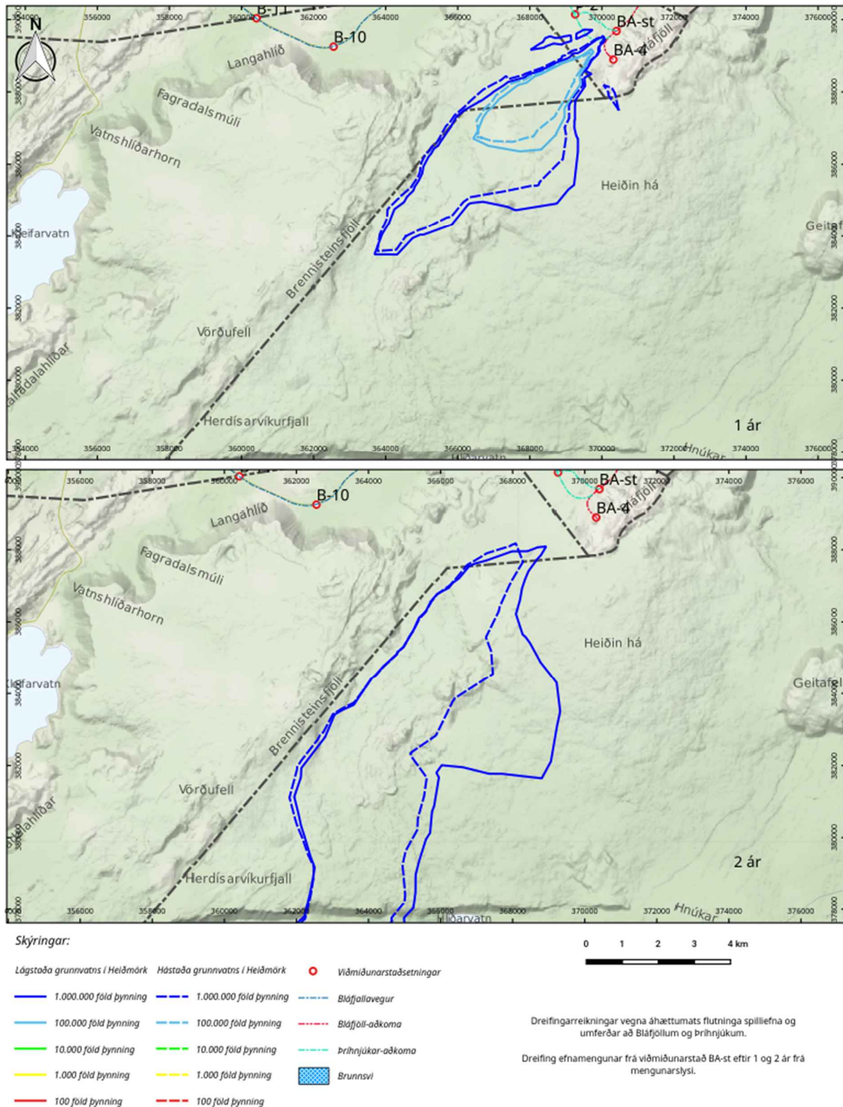
Mynd 73. Dreifing efnamengunar frá viðmiðunarstað BA-st eftir 1 og 2 ár frá mengunarslysi.
