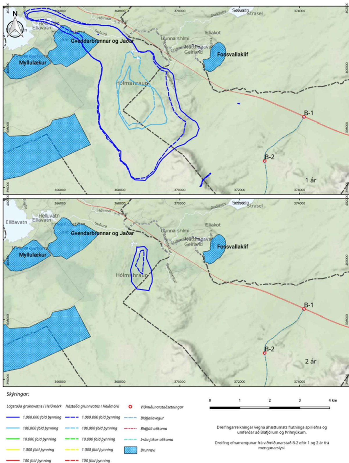
Mynd 8. Dreifing efnamengunar frá viðmiðunarstað B-2 eftir hálft, 1 og 2 ár frá mengunarslysi.
