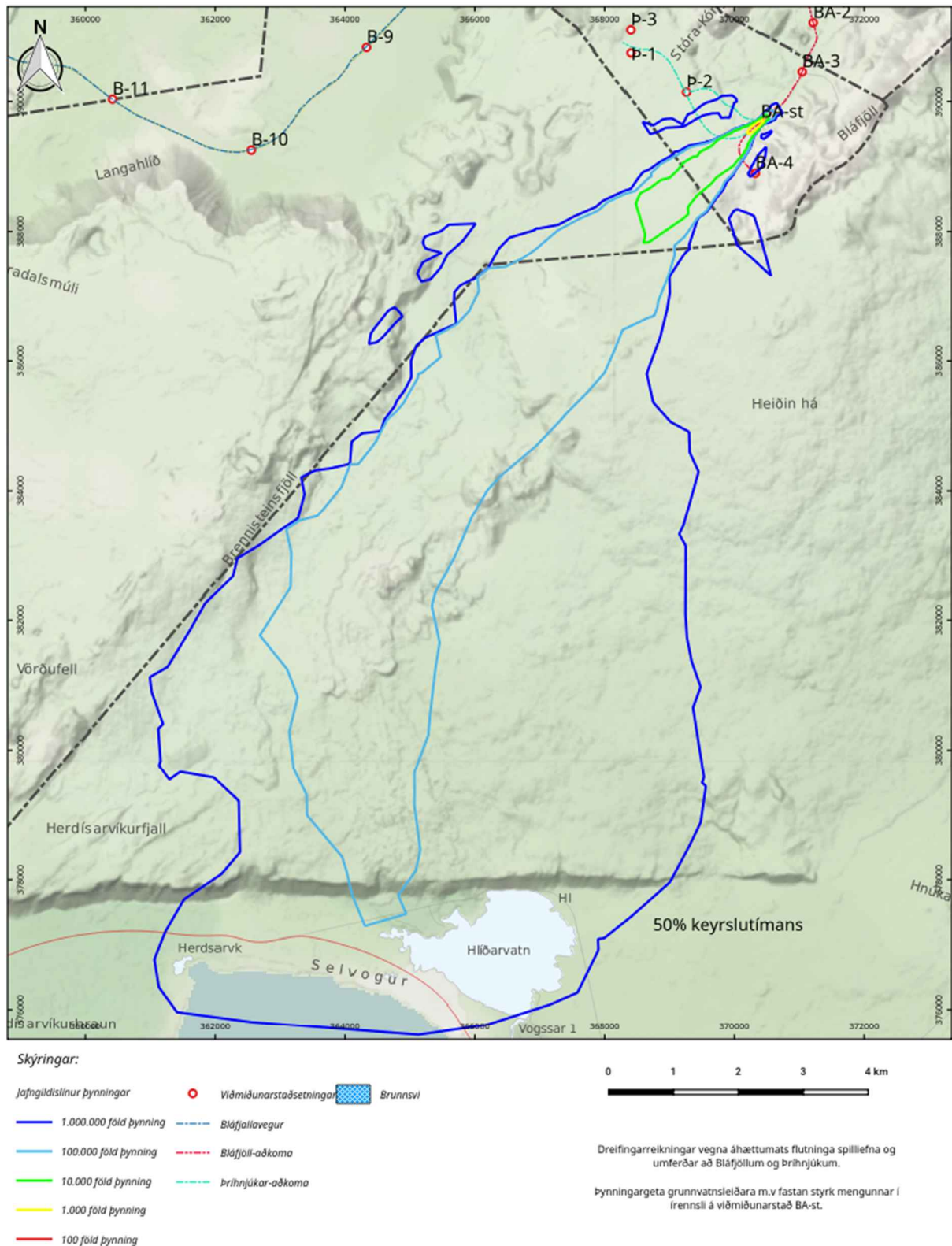
Mynd 75. Þynningargeta grunnvatnsleiðara miðað við fastan styrk mengunar í írennsli á viðmiðunarstað BA-st. Breytileiki yfir 50% keyrslutímans.
