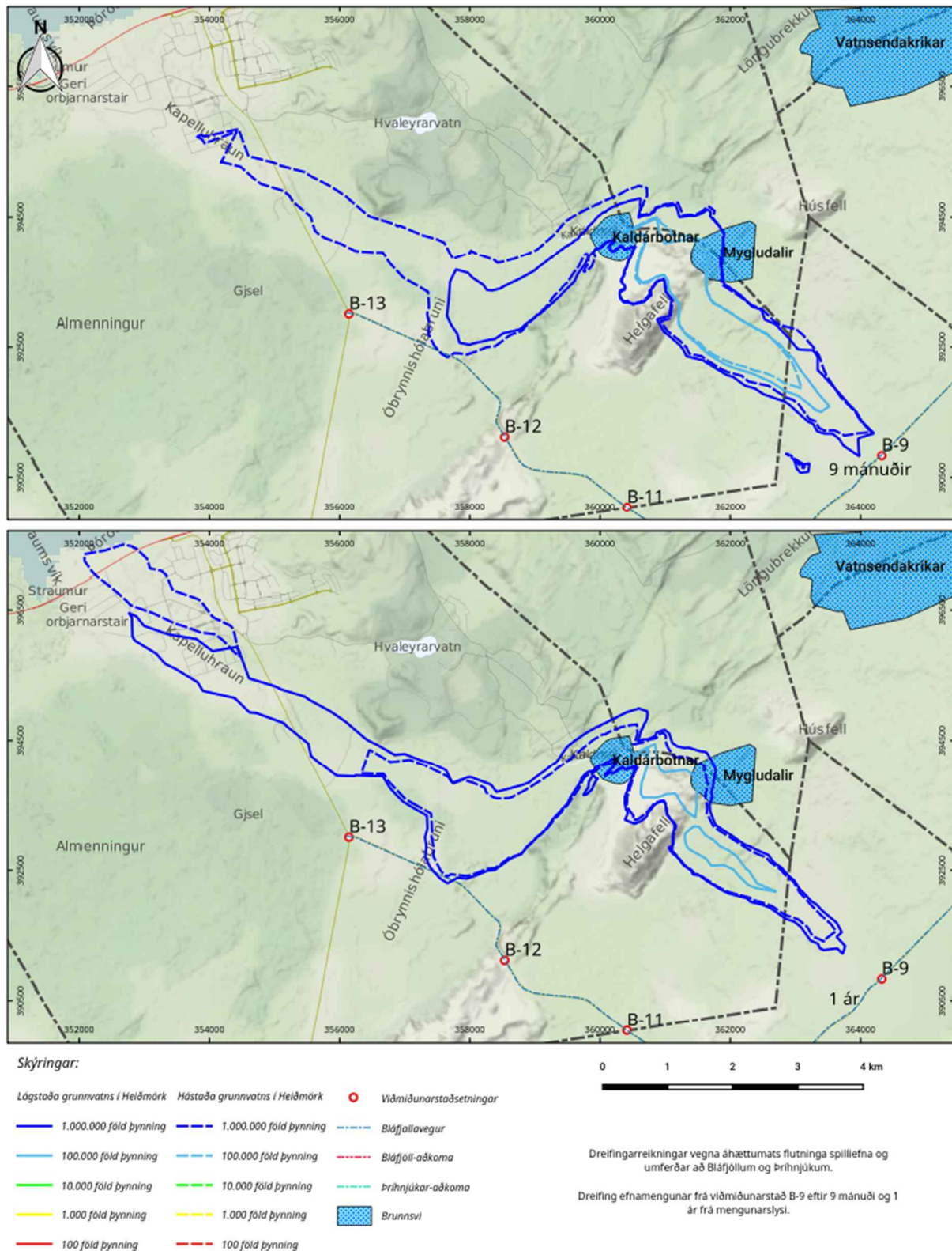
Mynd 42. Dreifing efnamengunar frá viðmiðunarstað B-9 eftir 9 mánuði og 1 ár frá mengunarslysi.
