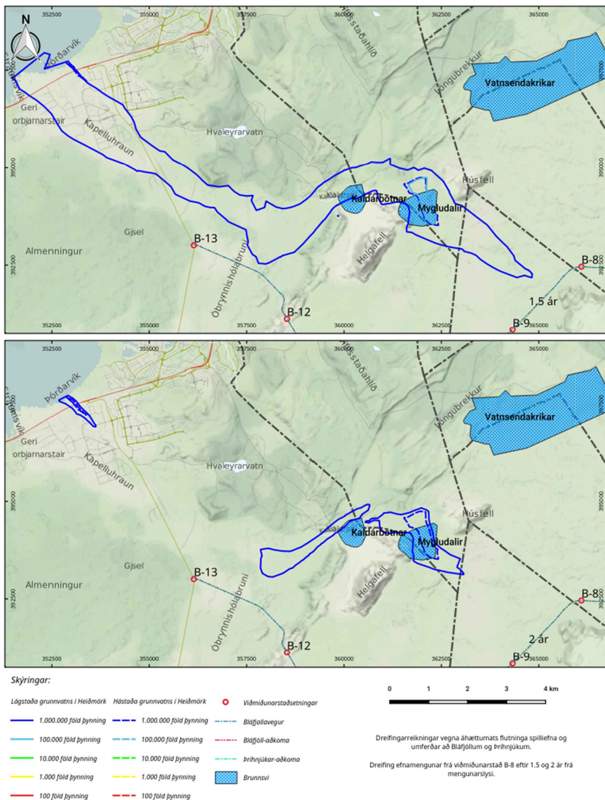
Mynd 38. Dreifing efnamengunar frá viðmiðunarstað B-8 eftir 1.5 og 2 ár frá mengunarslysi.
