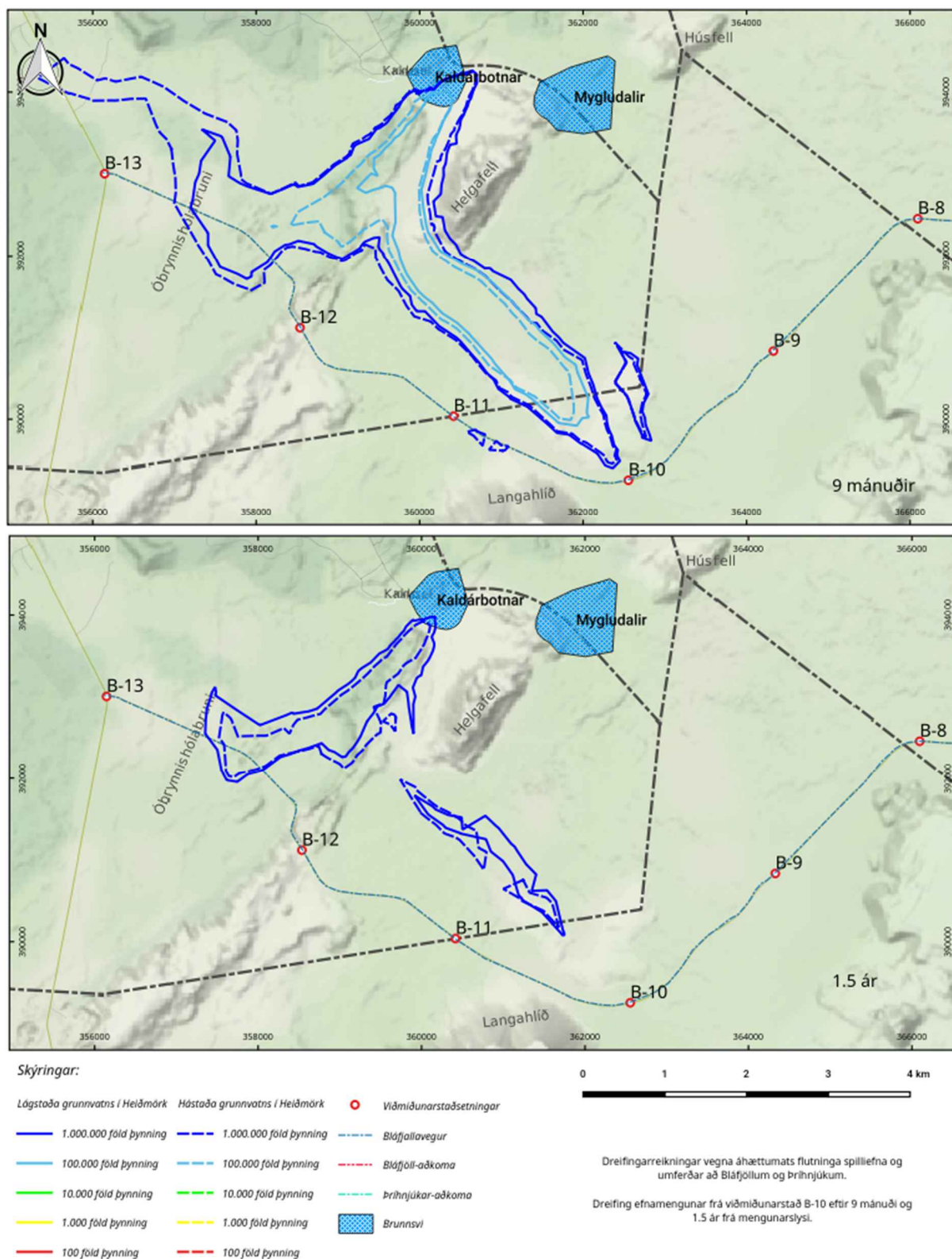
Mynd 46. Dreifing efnamengunar frá viðmiðunarstað B-10 eftir 9 mánuði og 1.5 ár frá mengunarslysi.
