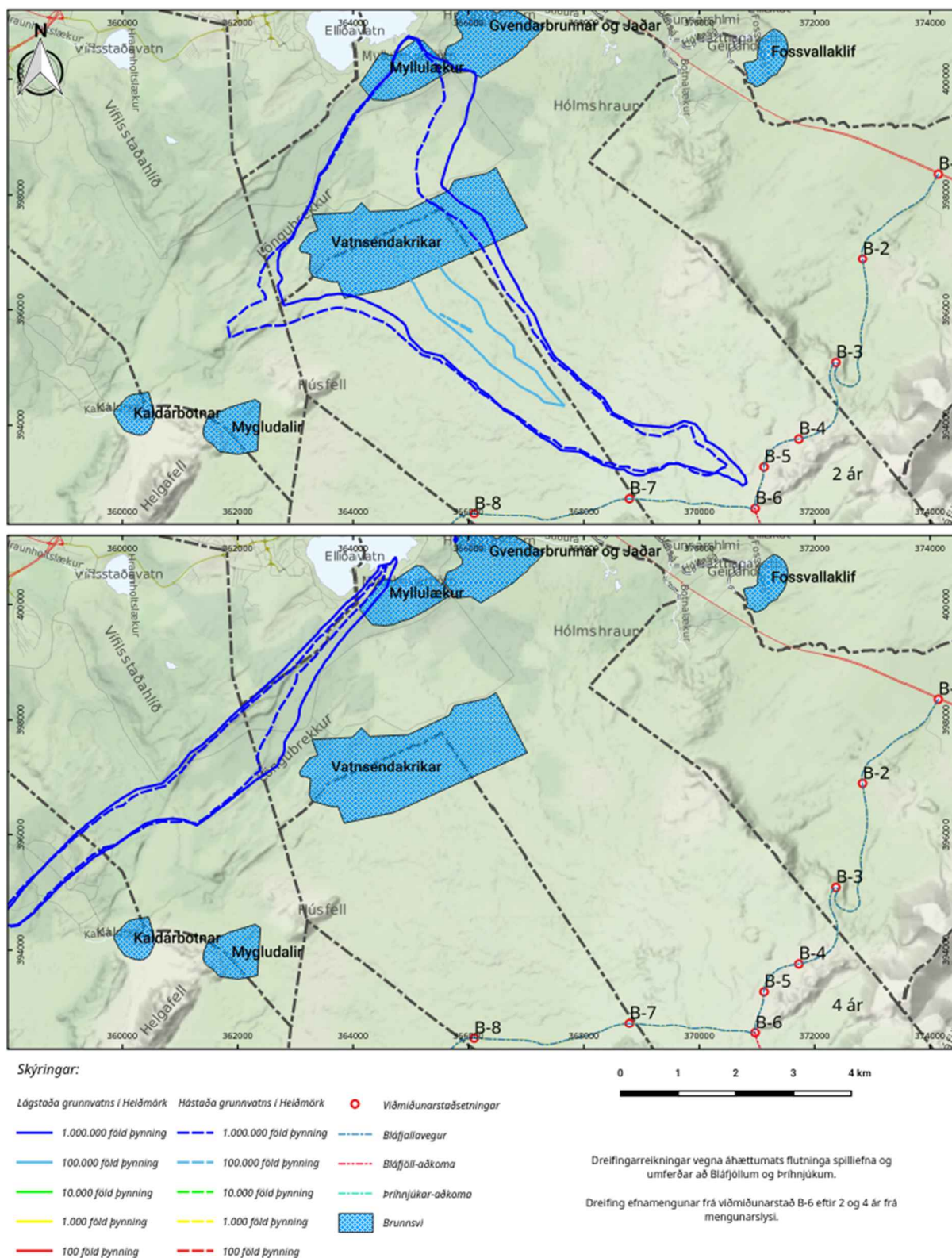
Mynd 28. Dreifing efnamengunar frá viðmiðunarstað B-6 eftir 2 og 4 ár frá mengunarslysi.
