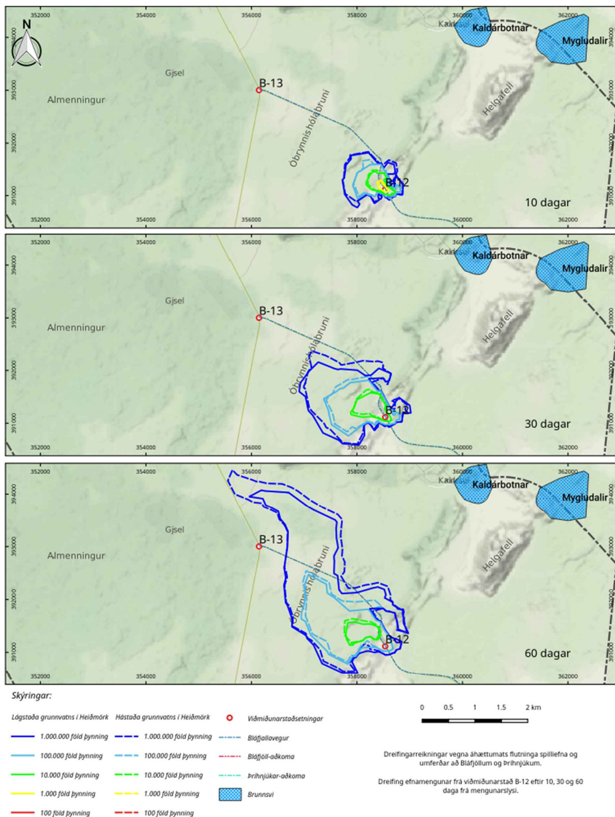
Mynd 52. Dreifing efnamengunar frá viðmiðunarstað B-12 eftir 10, 30 og 60 daga frá mengunarslysi.
