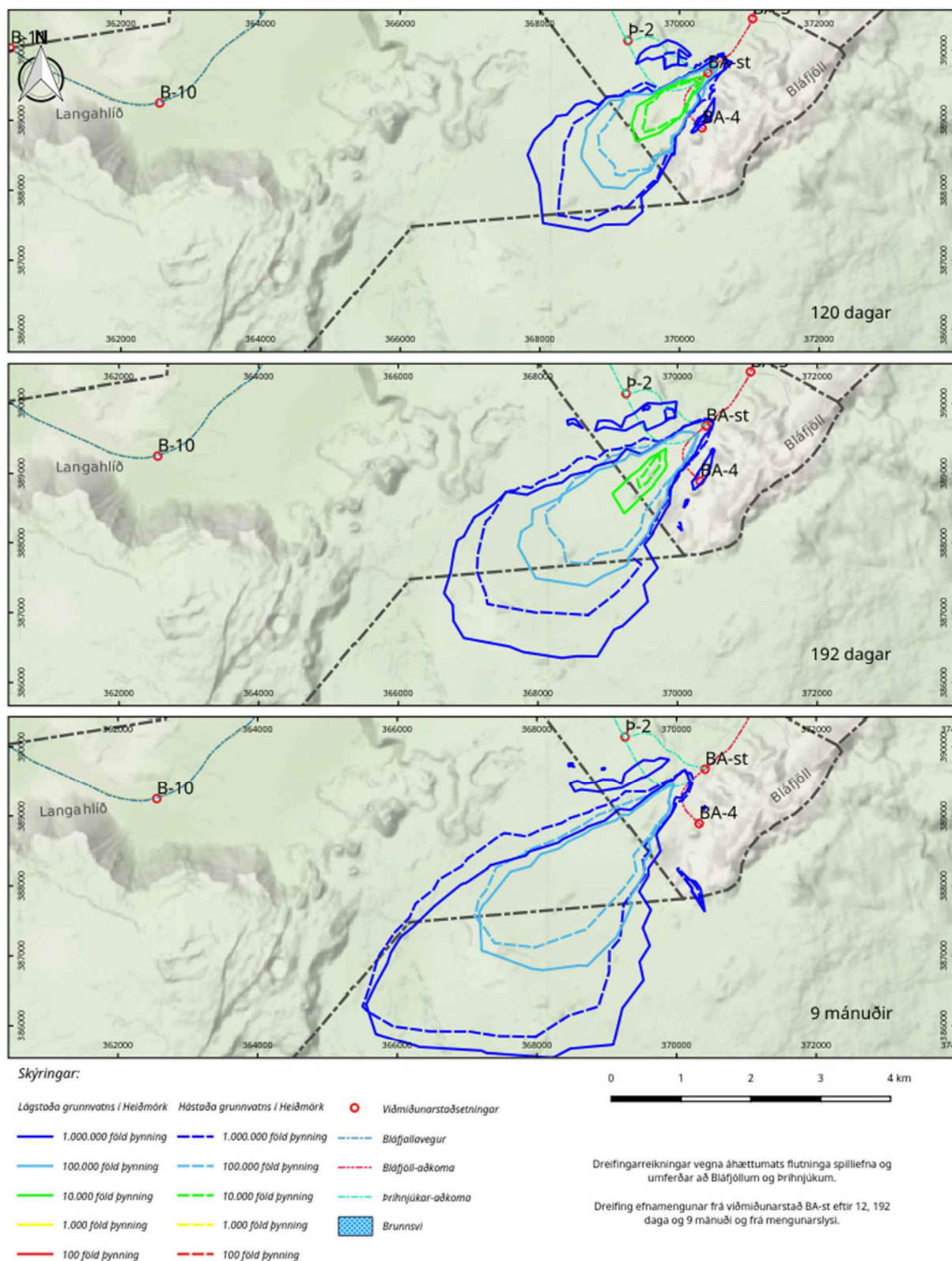
Mynd 72. Dreifing efnamengunar frá viðmiðunarstað BA-st eftir 120, 192 daga og 9 mánuði frá mengunarslysi.
