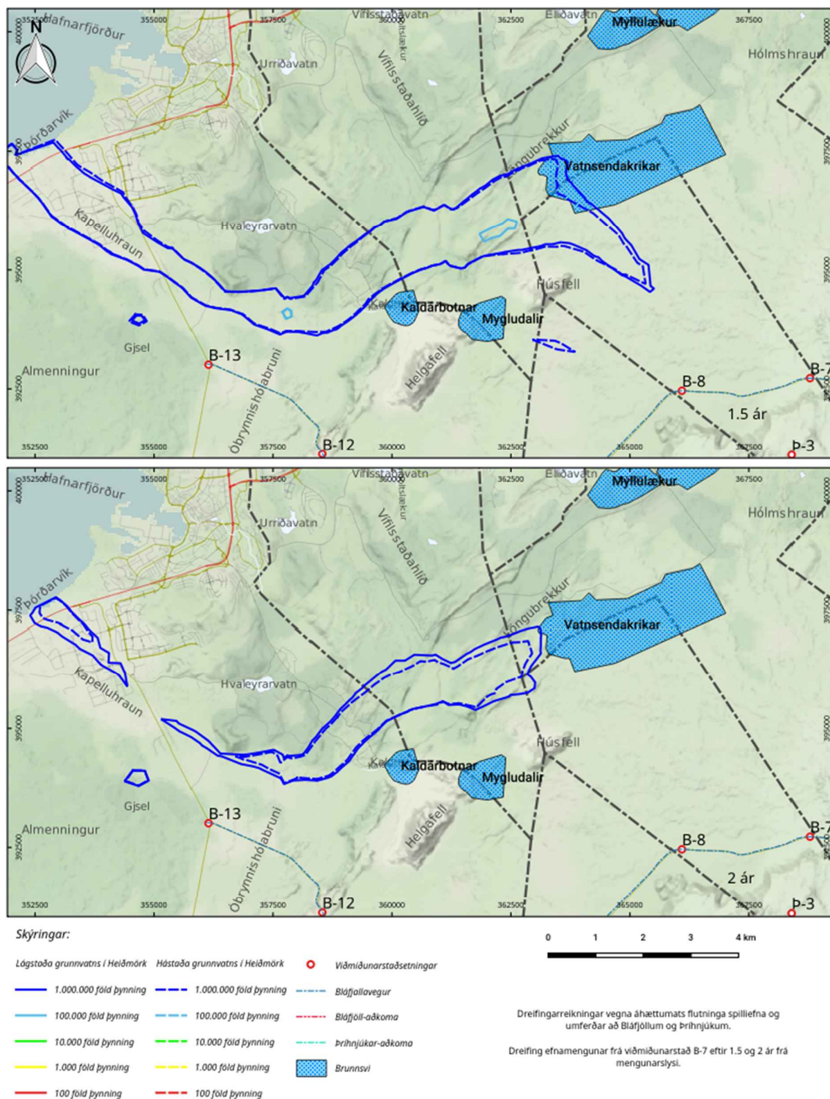
Mynd 33. Dreifing efnamengunar frá viðmiðunarstað B-7 eftir 1.5 og 2 ár frá mengunarslysi.
