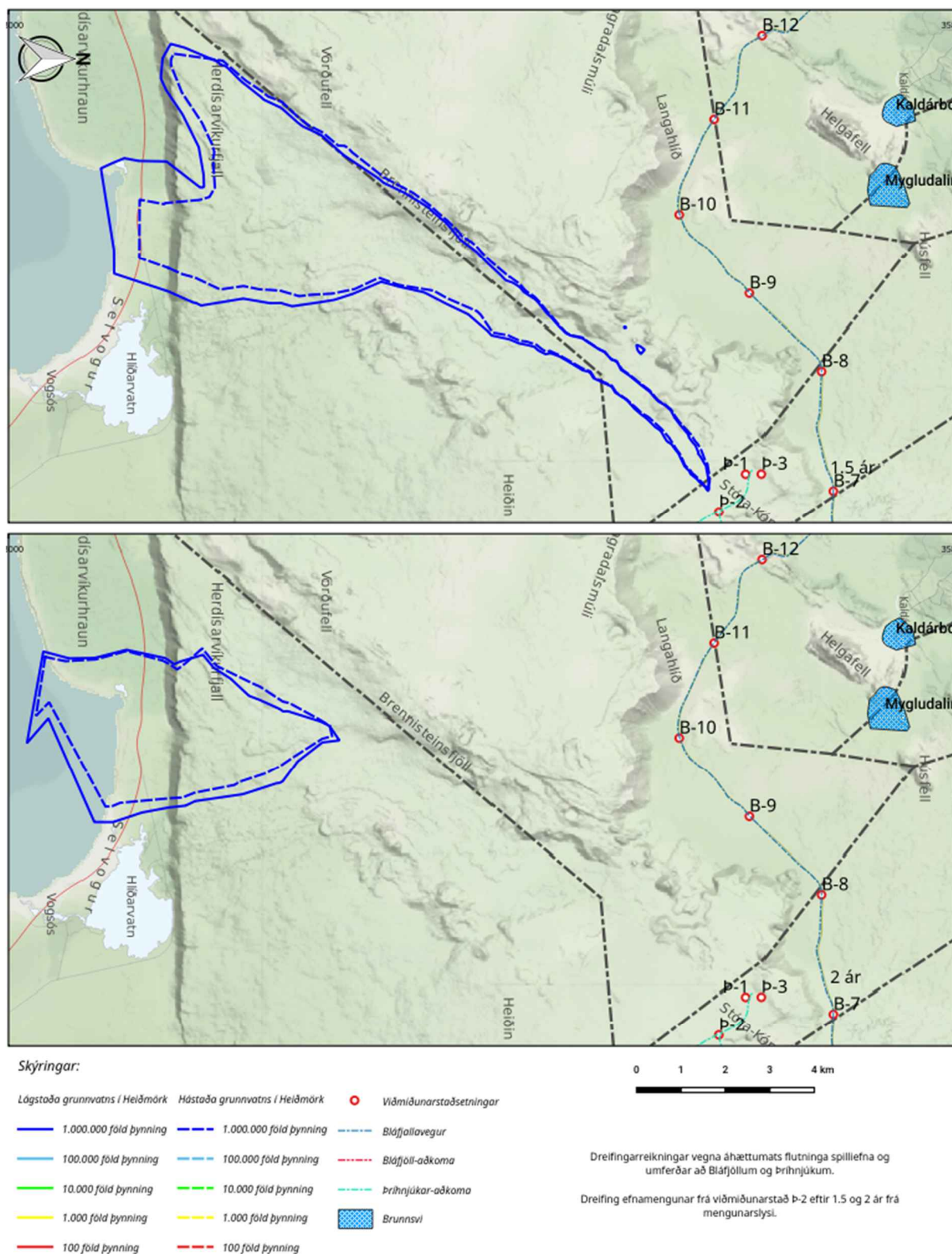
Mynd 86. Dreifing efnamengunar frá viðmiðunarstað P-2 eftir 1.5 og 2 ár frá mengunarslysi.
