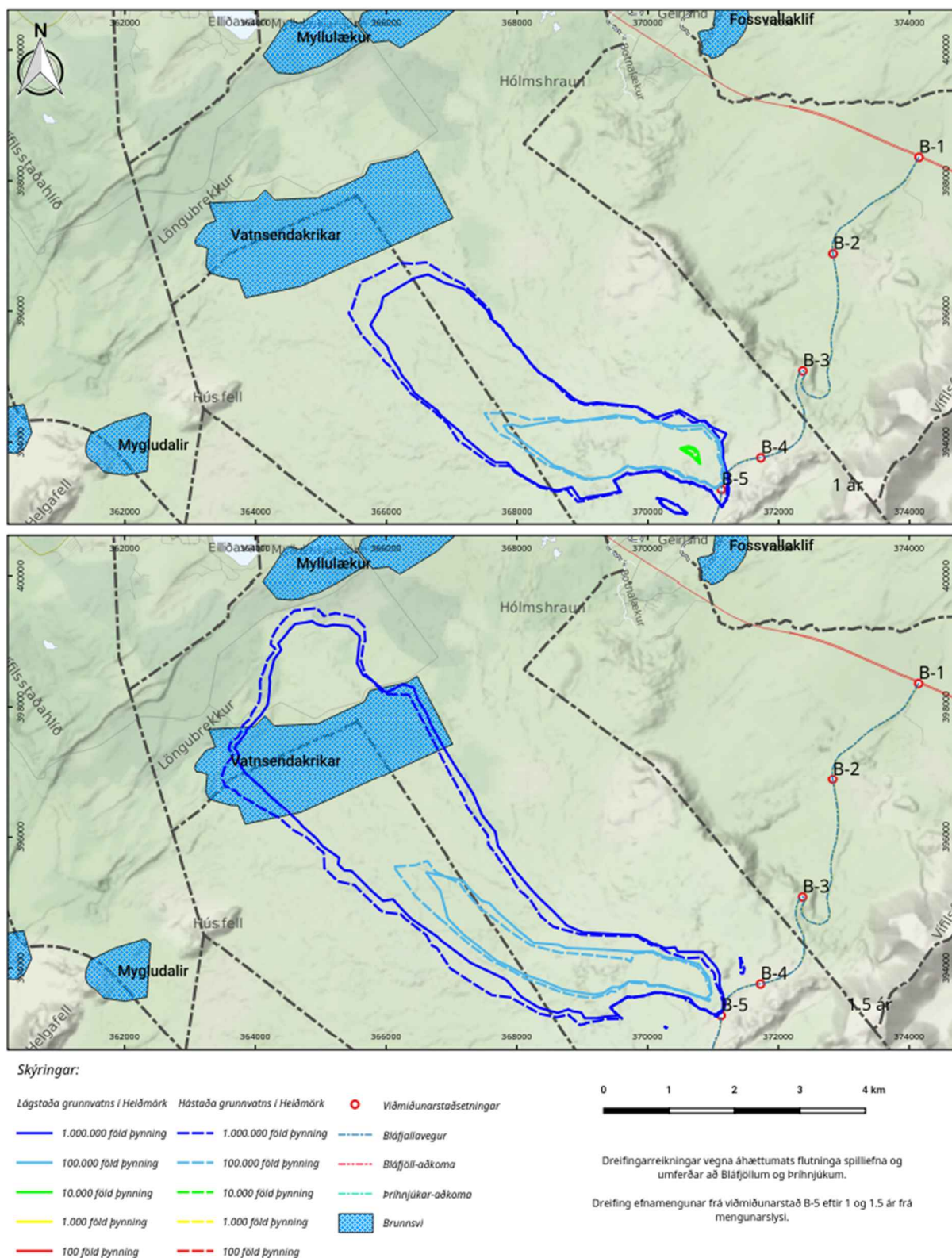
Mynd 22. Dreifing efnamengunar frá viðmiðunarstað B-5 eftir 1 og 1.5 ár frá mengunarslysi.
