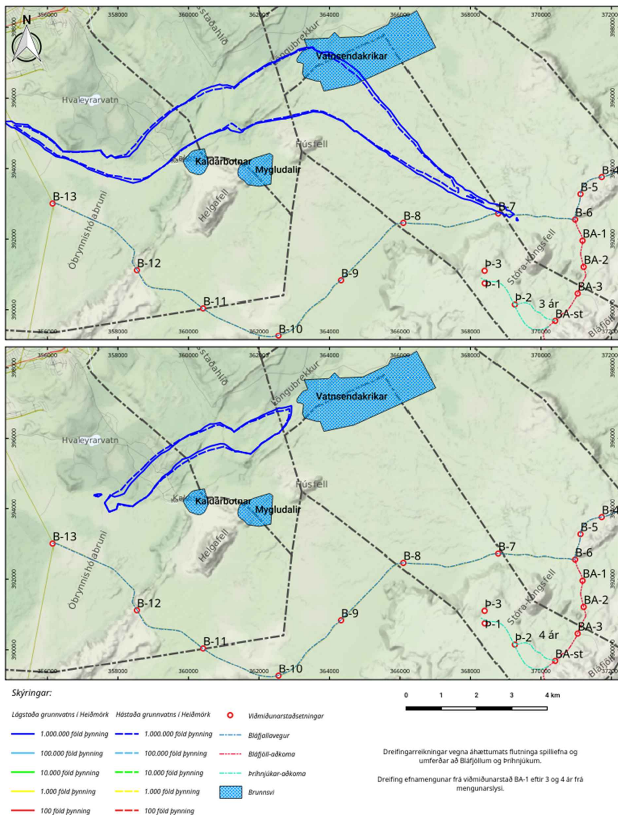
Mynd 58. Dreifing efnamengunar frá viðmiðunarstað BA-1 eftir 3 og 4 ár frá mengunarslysi.
