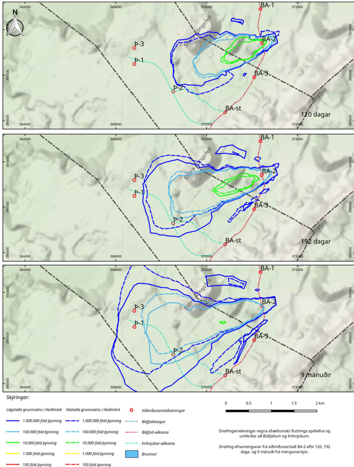
Mynd 61. Dreifing efnamengunar frá viðmiðunarstað BA-2 eftir 120, 192 daga og 9 mánuði frá mengunarslysi.
