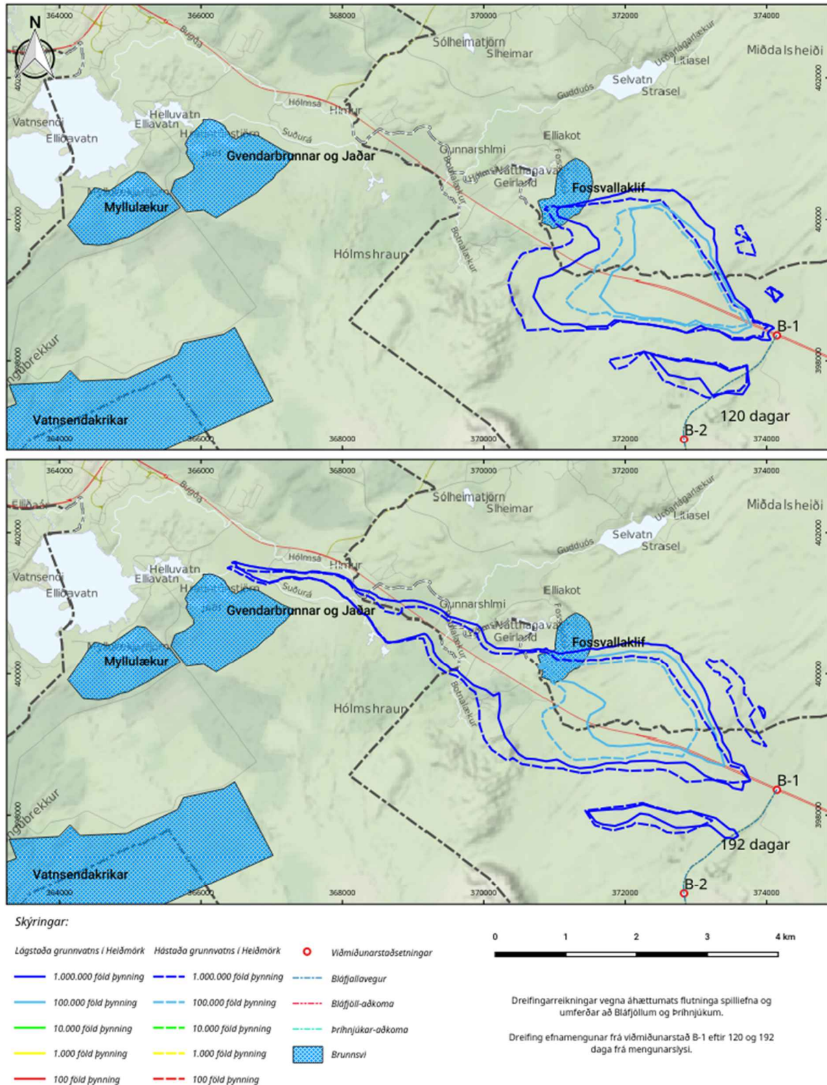
Mynd 3. Dreifing efnamengunar frá viðmiðunarstað B-1 eftir 120 daga og 192 daga.
