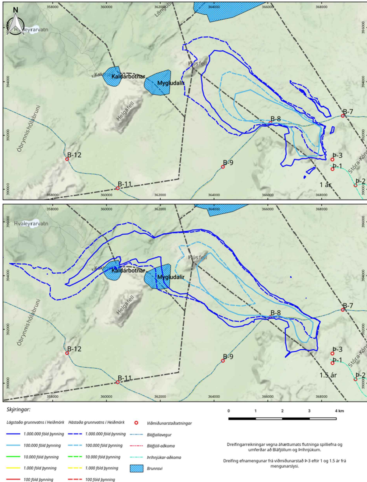
Mynd 91. Dreifing efnamengunar frá viðmiðunarstað P-3 eftir 1 og 1.5 ár frá mengunarslysi.
