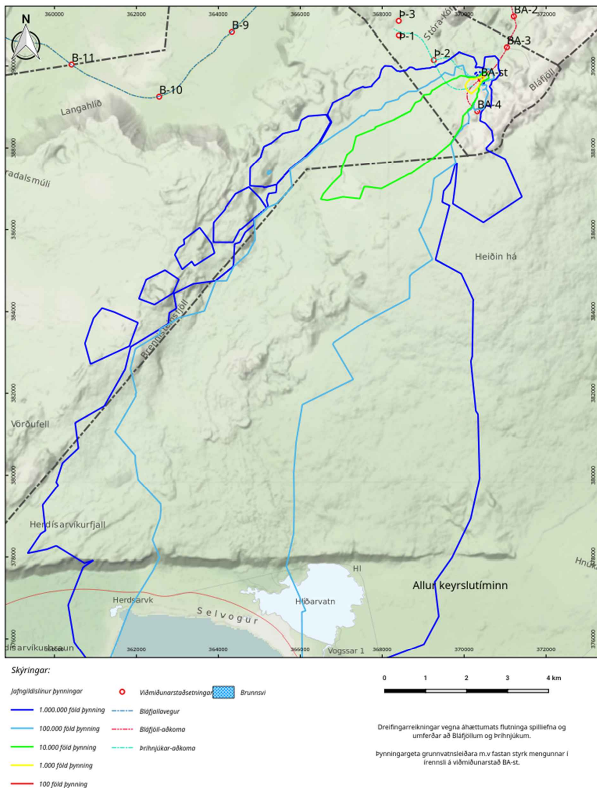
Mynd 74. Þynningargeta grunnvatnsleiðara miðað við fastan styrk mengunar í írennsli á viðmiðunarstað BA-st. Breytileiki yfir allan keyrslutímann.
