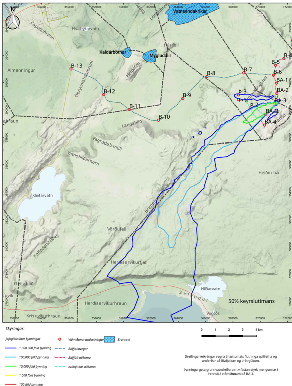
Mynd 70. Þýnningargeta grunnvatnsleiðara miðað við fastan styrk mengunar í írennsli á viðmiðunarstað BA-3. Breytileiki yfir 50% keyrslutímans.
