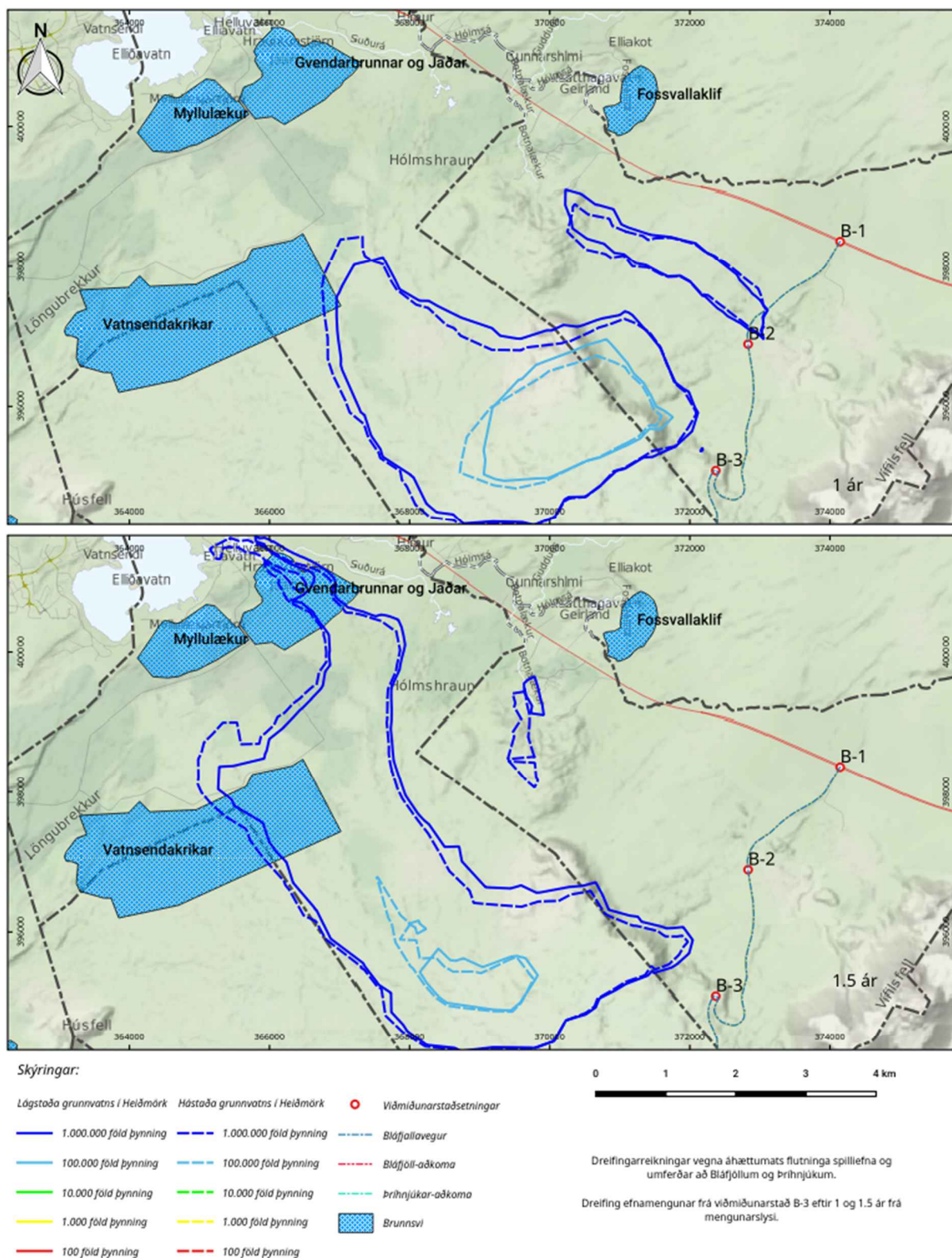
Mynd 12. Dreifing efnamengunar frá viðmiðunarstað B-3 eftir 1 og 1.5 ár frá mengunarslysi.
