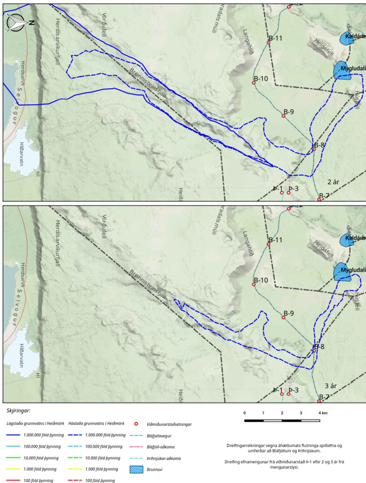
Mynd 80. Dreifing efnamengunar frá viðmiðunarstað B-1 eftir 2 og 3 ár frá mengunarslysi.
