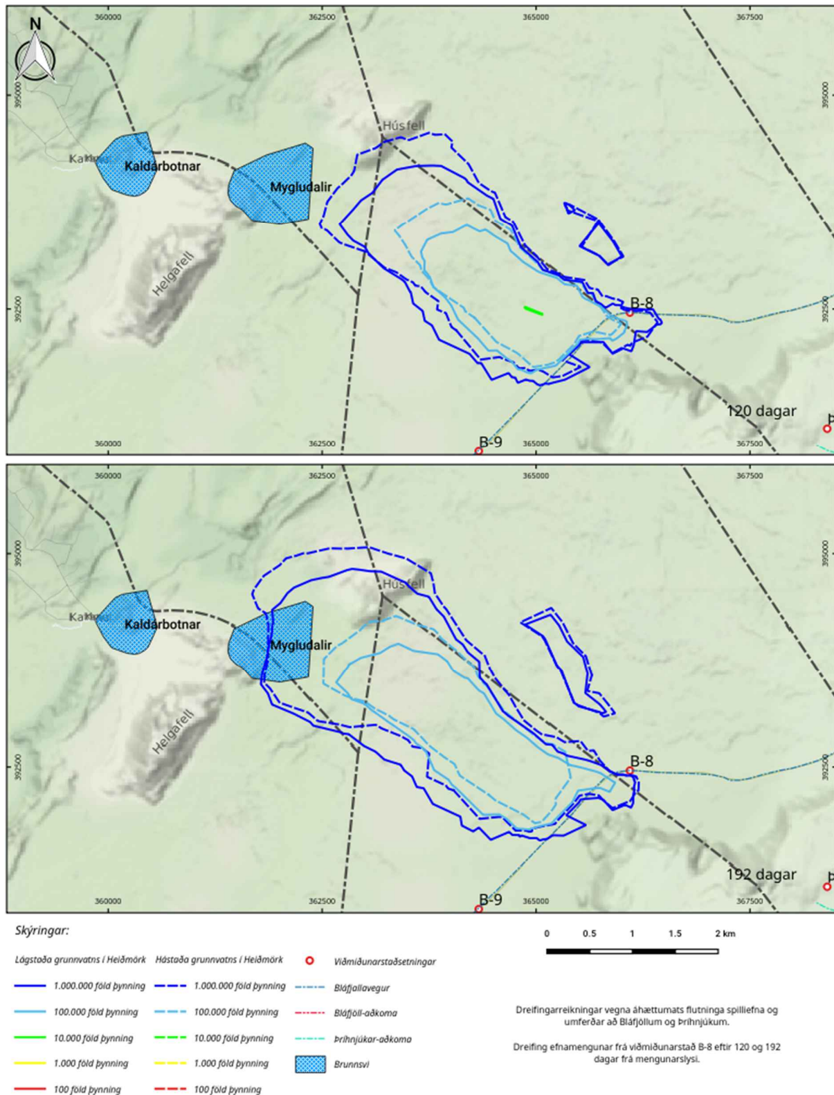
Mynd 36. Dreifing efnamengunar frá viðmiðunarstað B-8 eftir 120 og 192 dagar frá mengunarslysi.
