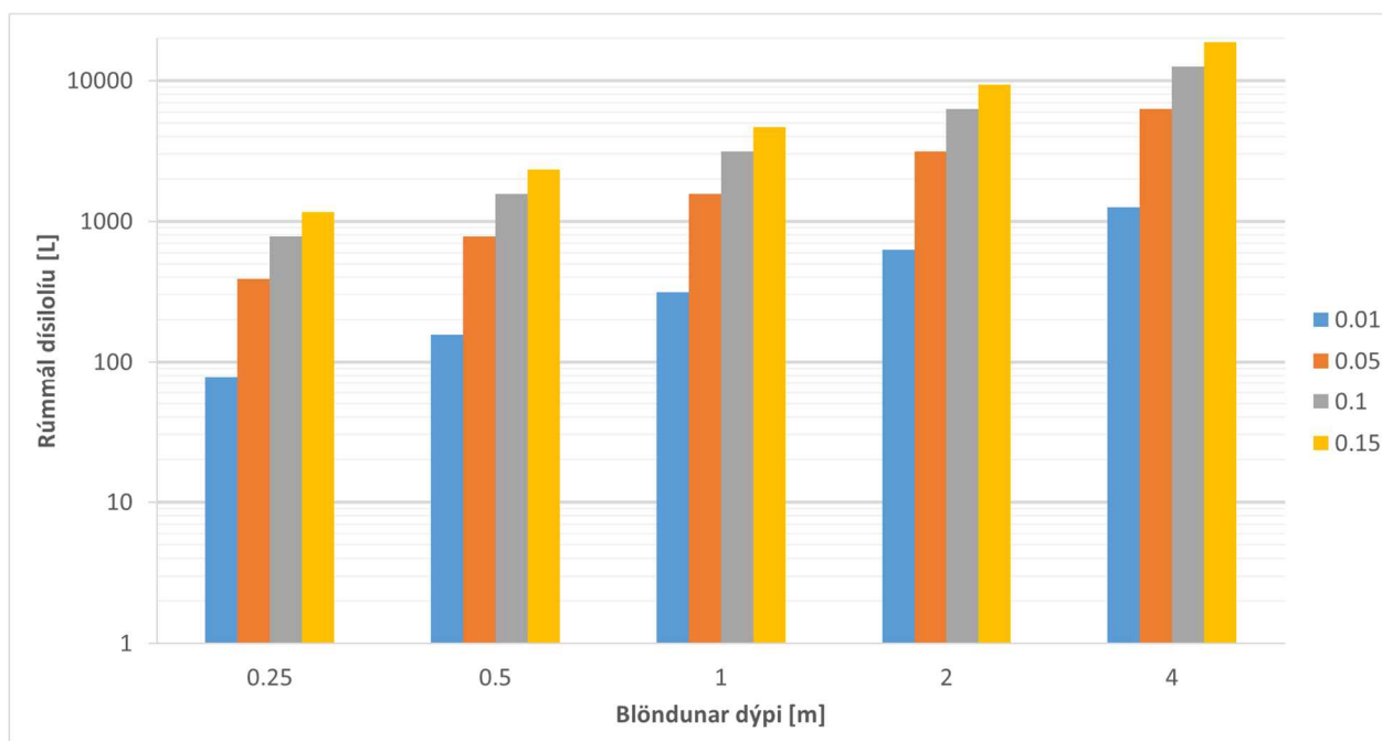
Mynd 96. Rúmmál díselolíu m.v. 1 ppm þynningu, fyrir viðmiðunarmengunarstyrk 0.01 (blár), 0.5 (appelsínugulur), 0.1 (grár) og 0.15 (gulur) mg/L.
