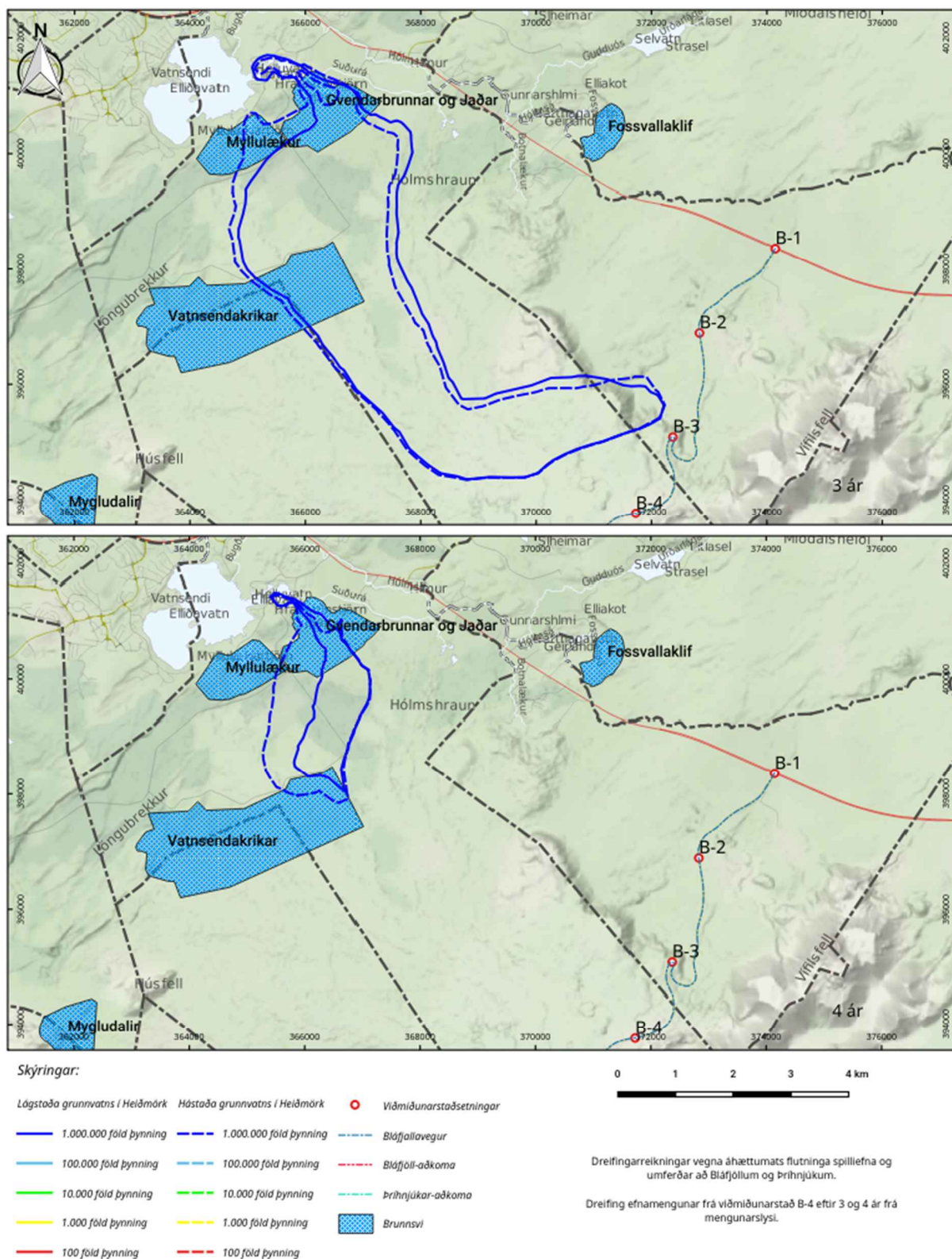
Mynd 18. Dreifing efnamengunar frá viðmiðunarstað B-4 eftir 3 og 4 ár frá mengunarslysi.
