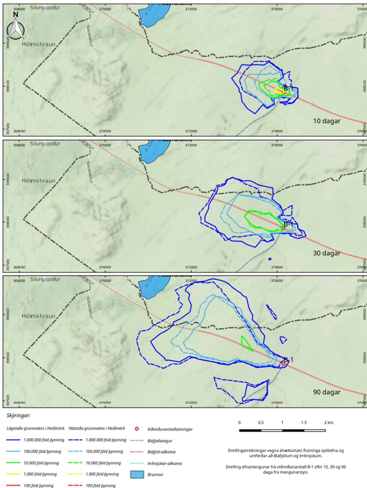
Mynd 2. Dreifing efnamengunar frá viðmiðunarstað B-1 eftir 10, 30 og 90 daga frá mengunarslysi.
