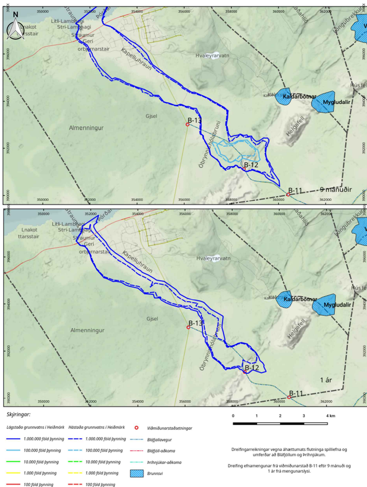
Mynd 50. Dreifing efnamengunar frá viðmiðunarstað B-11 eftir 9 mánuði og 1 ár frá mengunarslysi.
