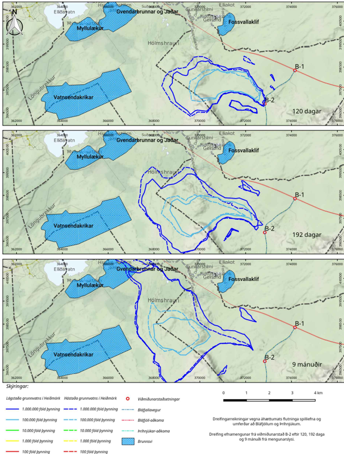
Mynd 7. Dreifing efnamengunar frá viðmiðunarstað B-2 eftir 120, 192 daga og 9 mánuði frá mengunarslysi.
