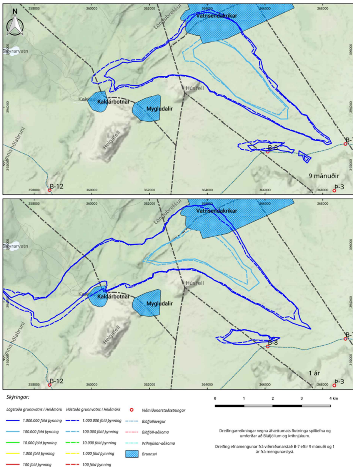
Mynd 32. Dreifing efnamengunar frá viðmiðunarstað B-7 eftir 9 mánuði og 1 ár frá mengunarslysi.
