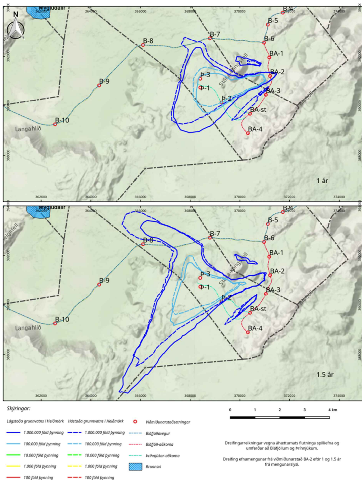
Mynd 62. Dreifing efnamengunar frá viðmiðunarstað BA-2 eftir 1 og 1.5 ár frá mengunarslysi.
