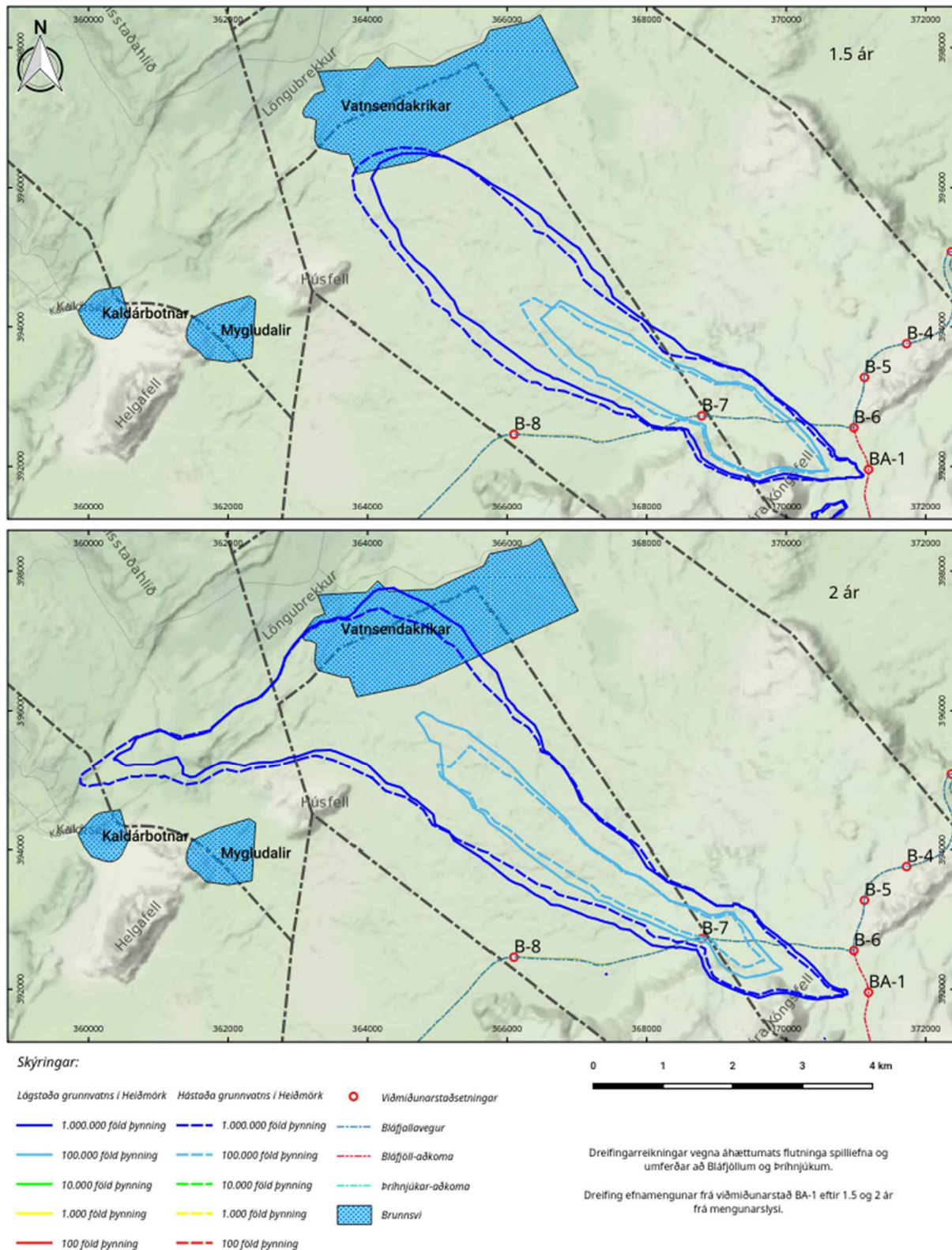
Mynd 57. Dreifing efnamengunar frá viðmiðunarstað BA-1 eftir 1.5 og 2 ár frá mengunarslysi.
