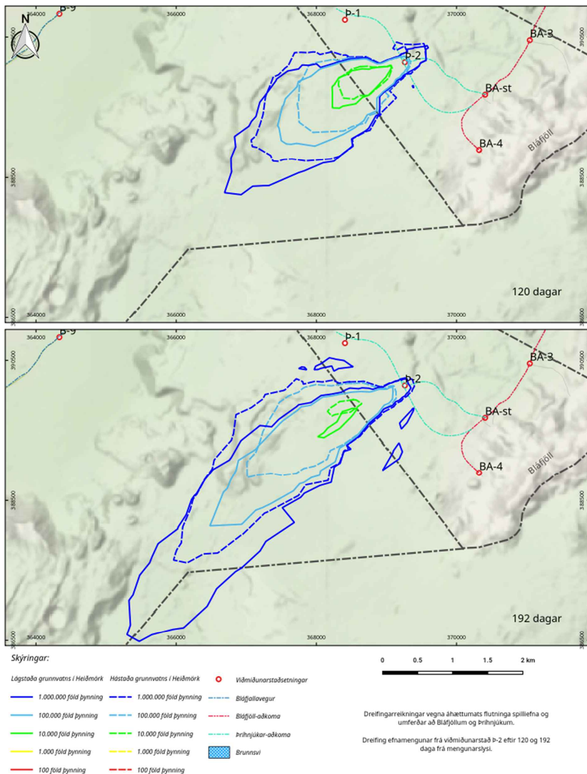
Mynd 84. Dreifing efnamengunar frá viðmiðunarstað P-2 eftir 120 og 192 daga frá mengunarslysi.
