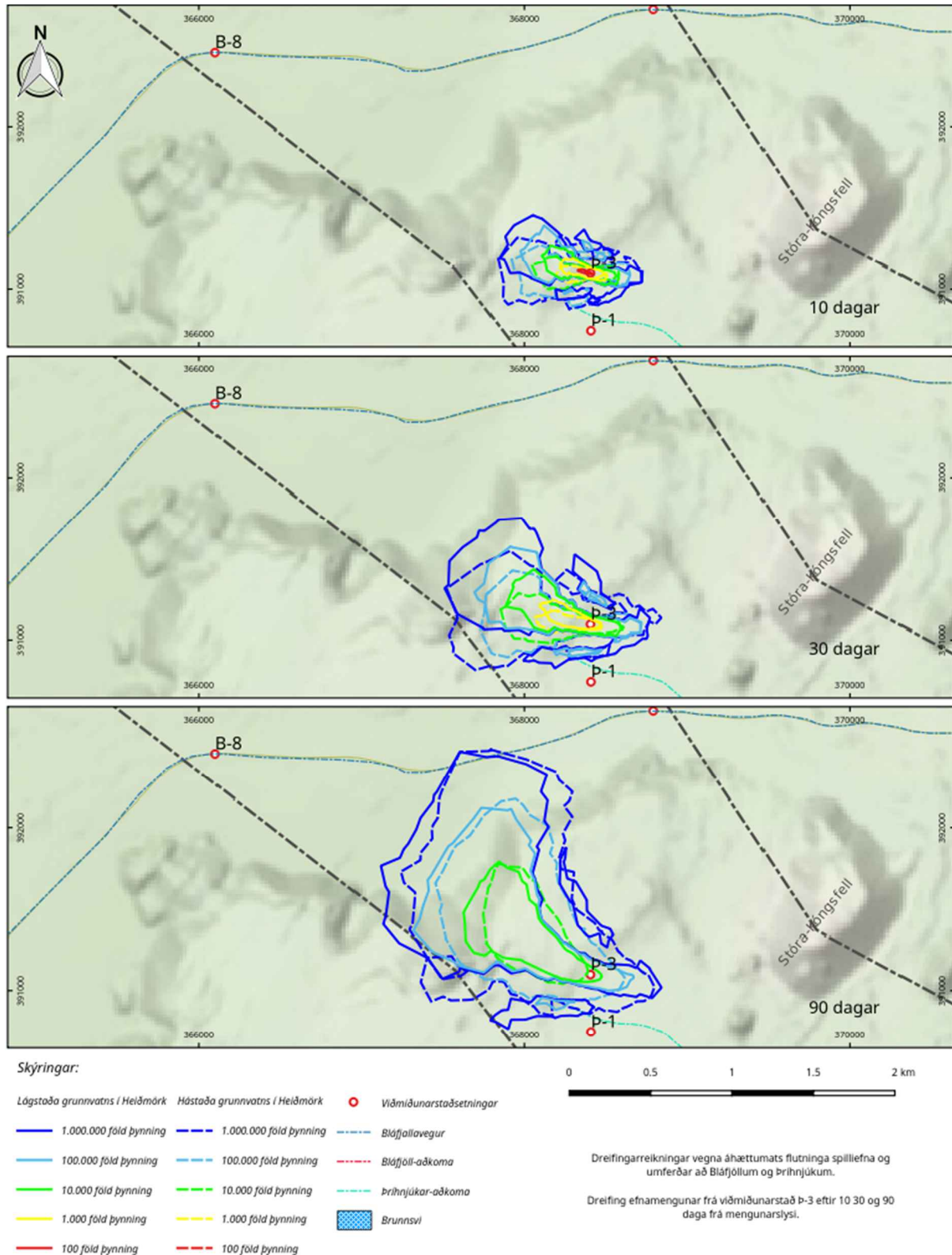
Mynd 89. Dreifing efnamengunar frá viðmiðunarstað P-3 eftir 10, 30 og 90 daga frá mengunarslysi.
