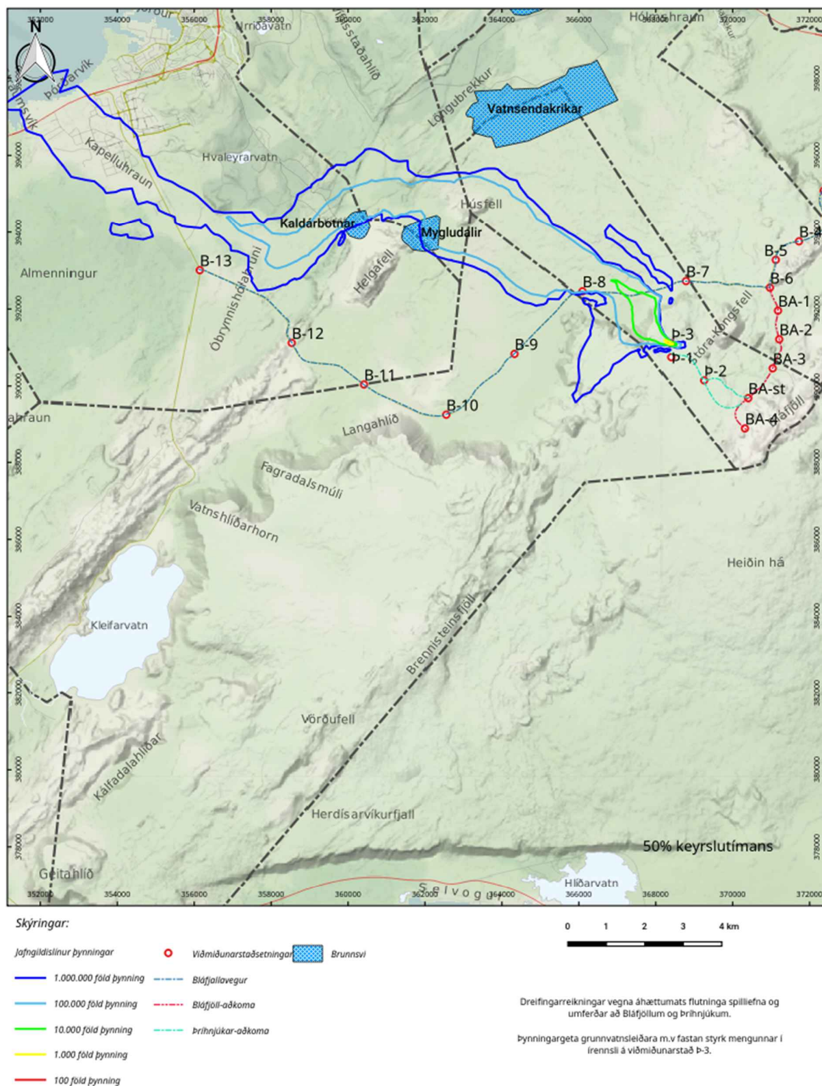
Mynd 94. Þynningargeta grunnvatnsleiðara miðað við fastan styrk mengunar í írennsli á viðmiðunarstað Þ-3. Breytileiki yfir 50% keýrslutímans.
