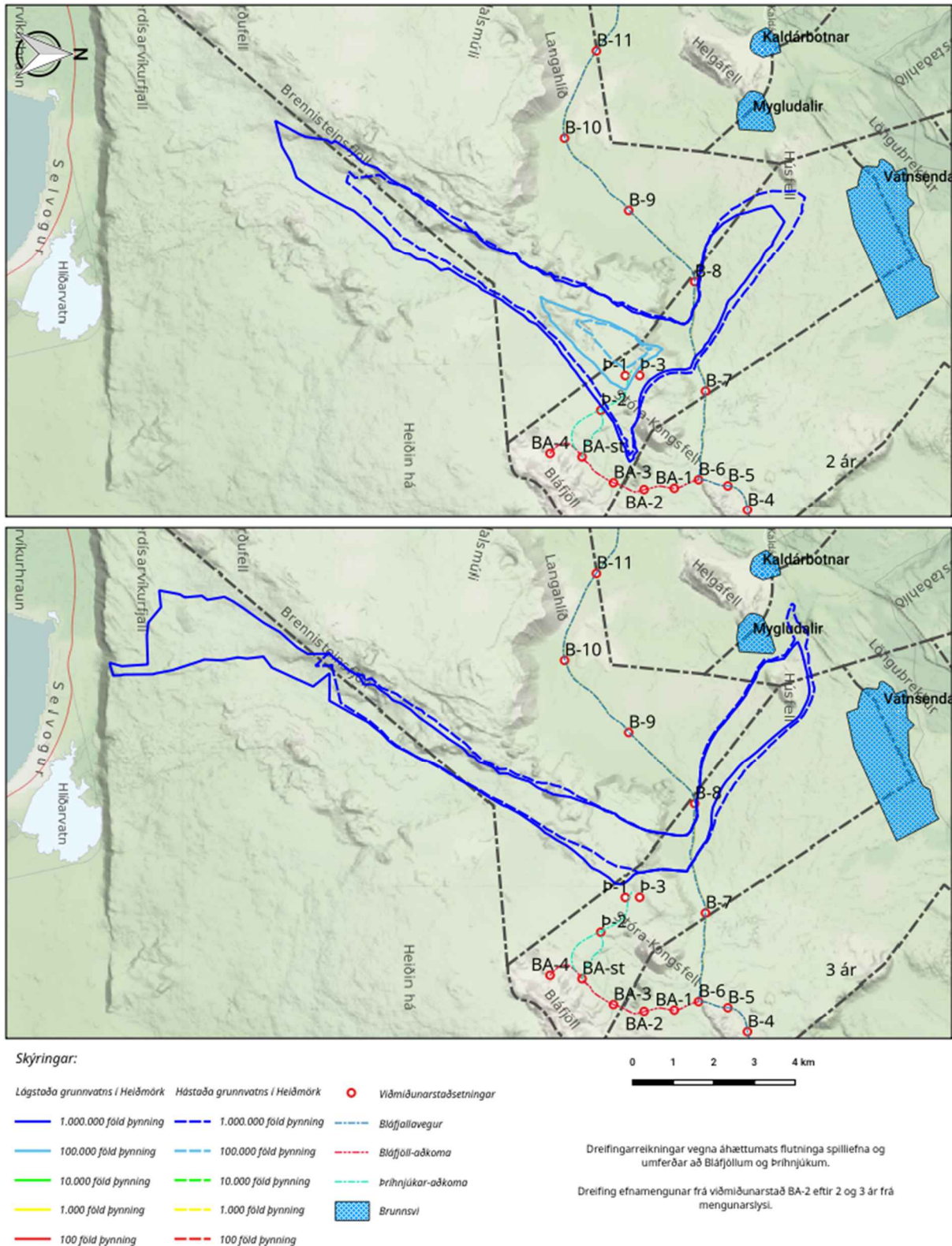
Mynd 63. Dreifing efnamengunar frá viðmiðunarstað BA-2 eftir 2 og 3 ár frá mengunarslysi.
