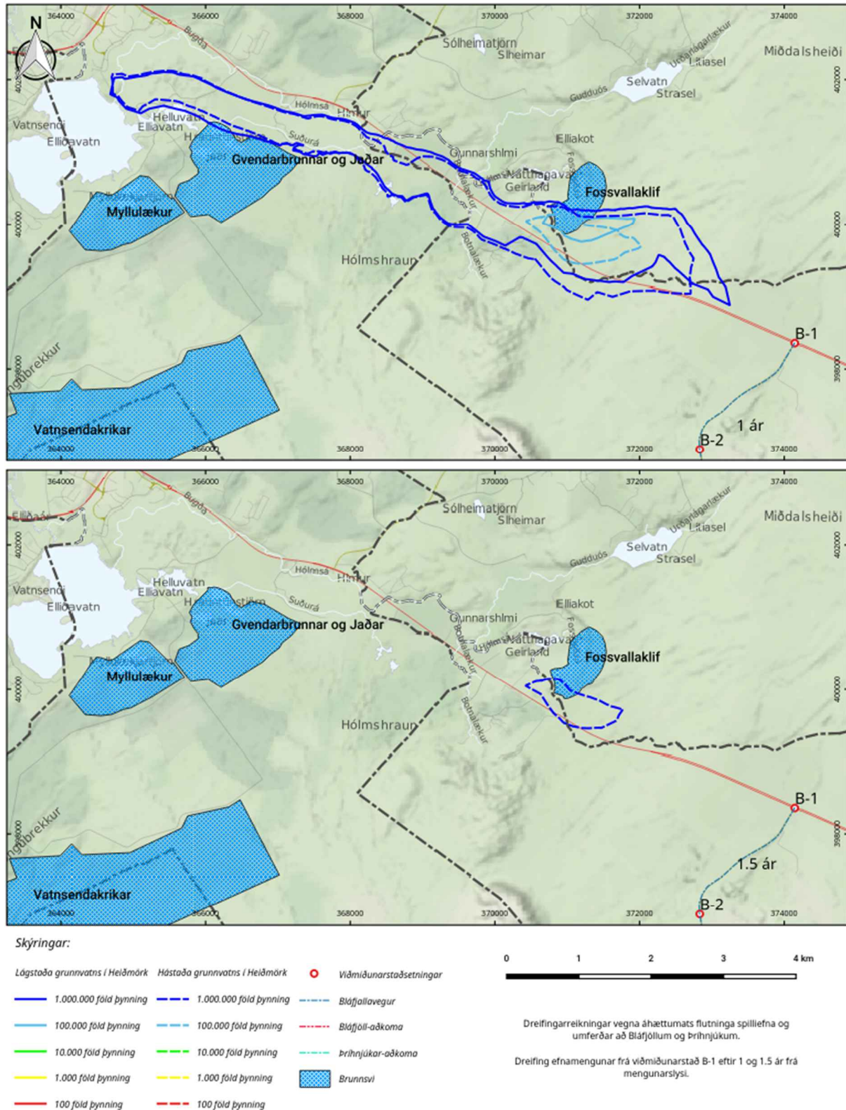
Mynd 4. Dreifing efnamengunar frá viðmiðunarstað B-1 eftir 1 og 1.5 ár frá mengunarslysi.
