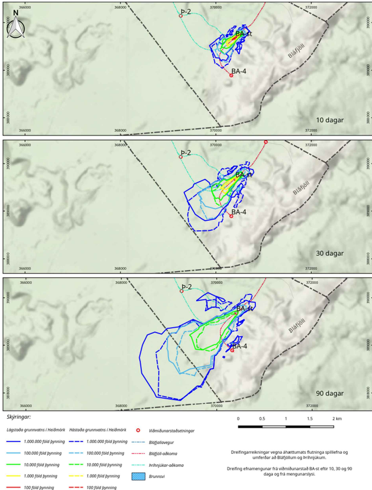
Mynd 71. Dreifing efnamengunar frá viðmiðunarstað BA-st eftir 10, 30 og 90 daga frá mengunarslysi.
