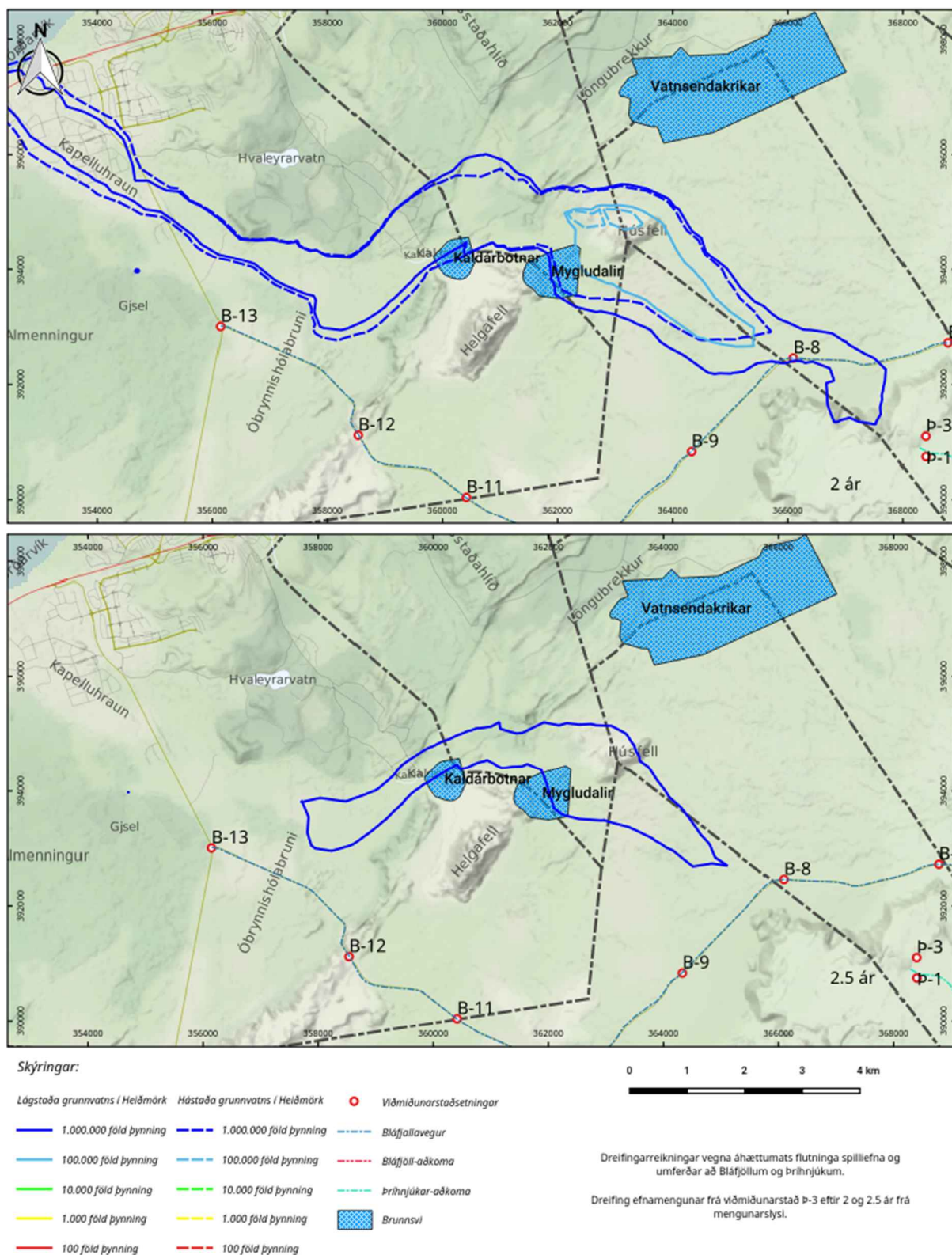
Mynd 92. Dreifing efnamengunar frá viðmiðunarstað P-3 eftir 2 og 2.5 ár frá mengunarslysi.
