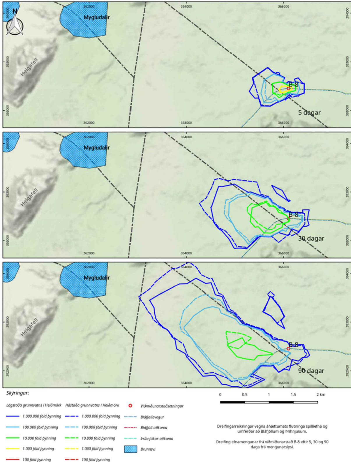
Mynd 35. Dreifing efnamengunar frá viðmiðunarstað B-8 eftir 5, 30 og 90 daga frá mengunarslysi.
