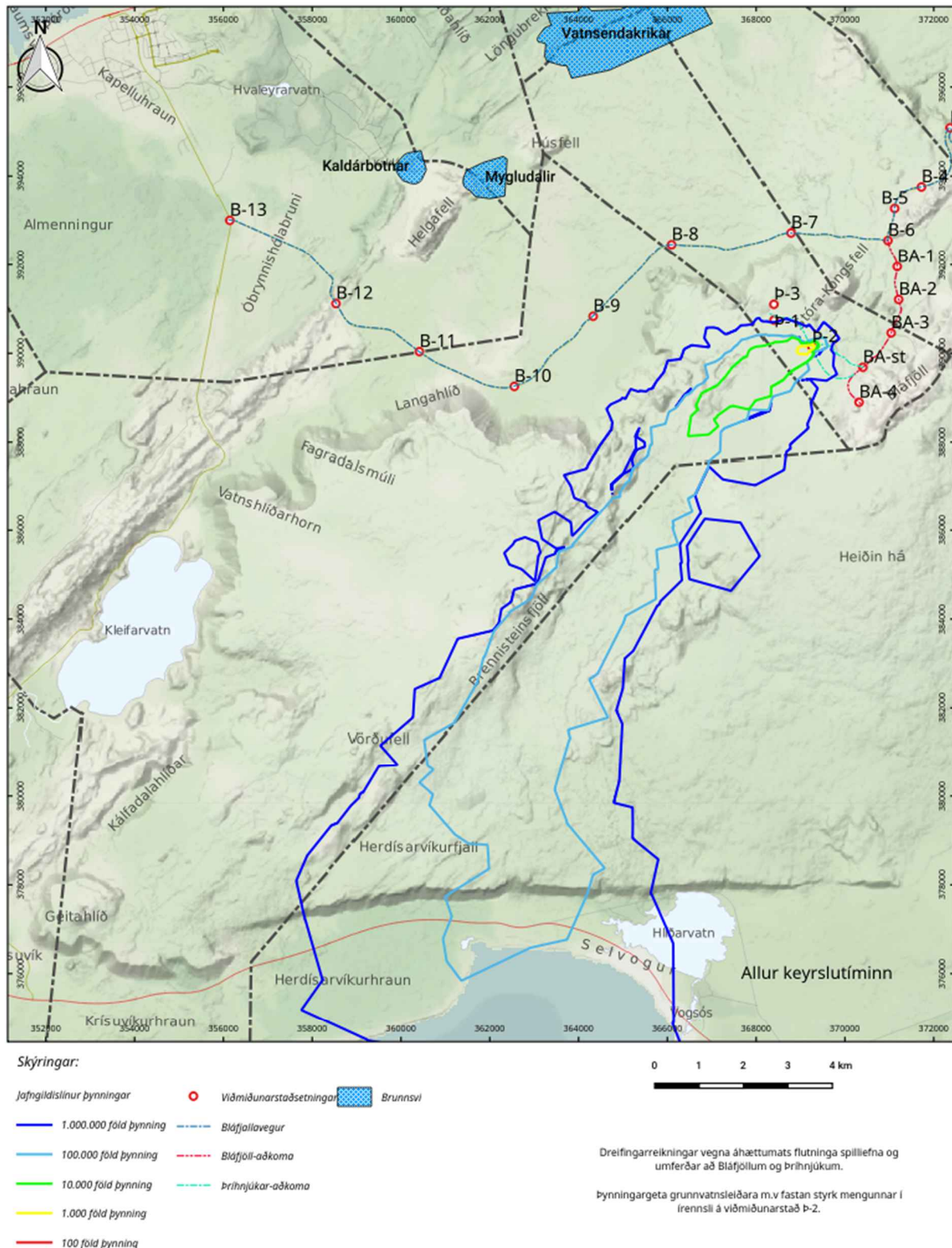
Mynd 87. Þýnningargeta grunnvatnsleiðara miðað við fastan styrk mengunar í írennsli á viðmiðunarstað Þ-2. Breytileiki yfir allan keyrslutímann.
