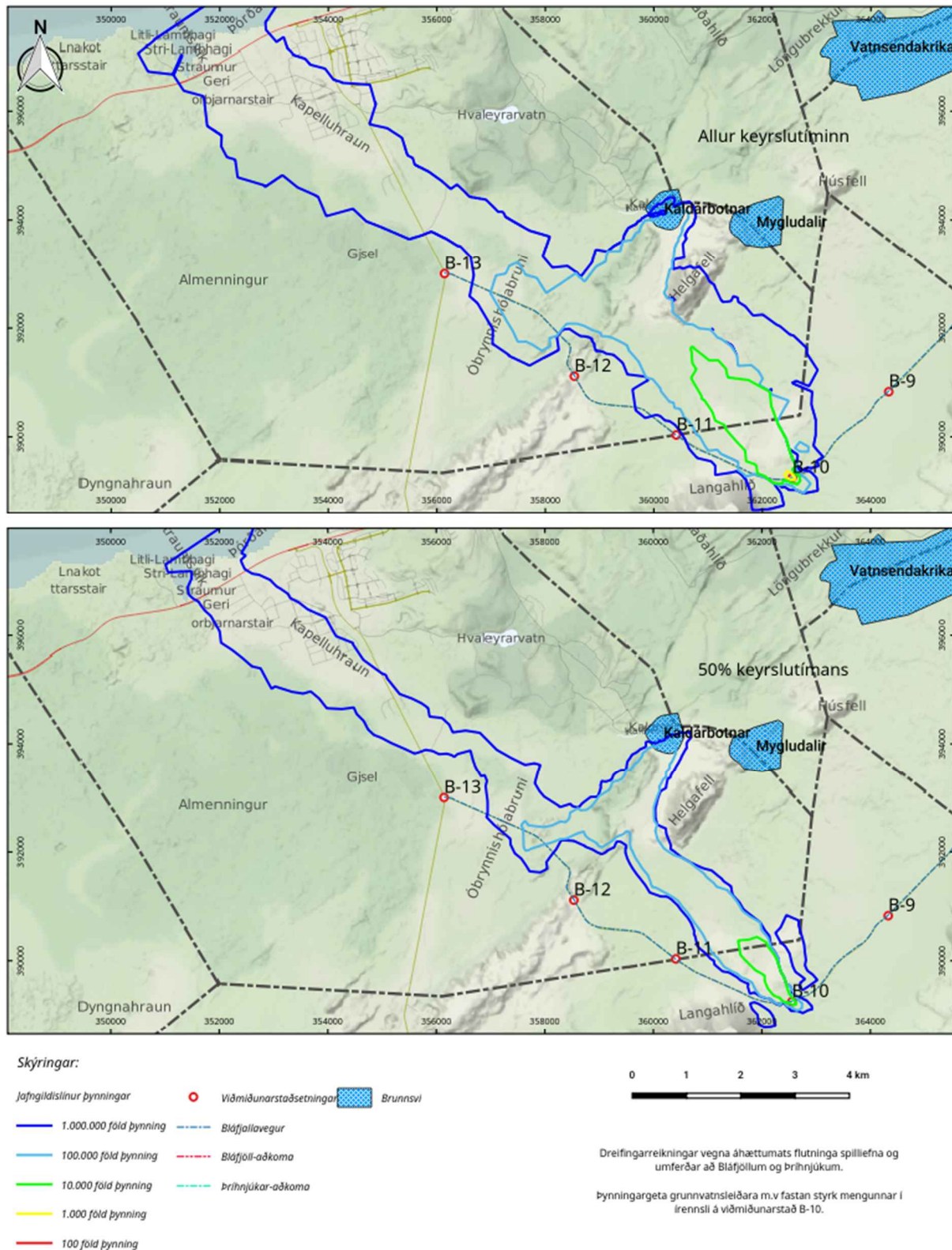
Mynd 47. Þýnningargeta grunnvatnsleiðara miðað við fastan styrk mengunar í írennsli á viðmiðunarstað B-10. Breytileiki yfir allan keyrslutímamann (efri mynd) og helming hans (neðri mynd).
