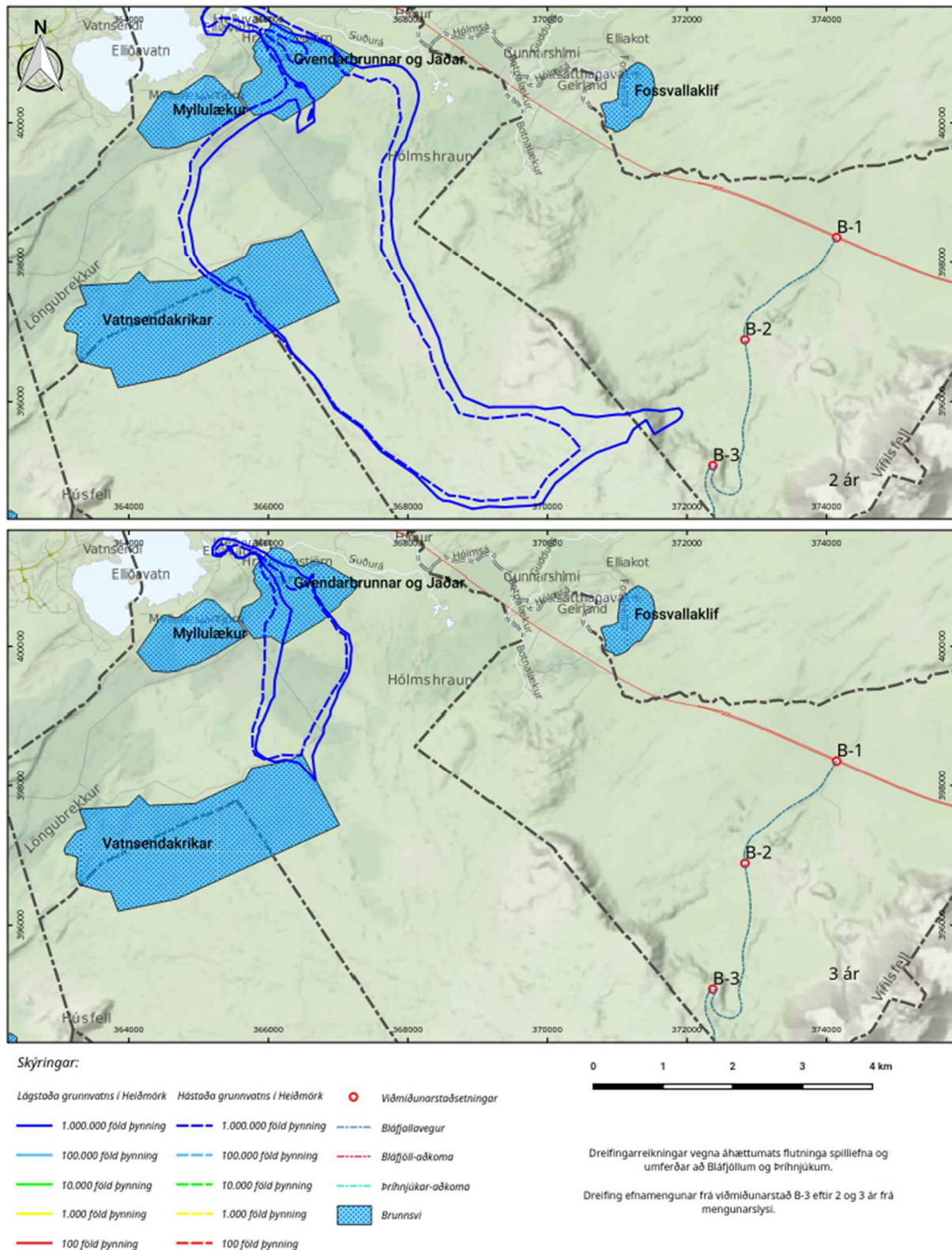
Mynd 13. Dreifing efnamengunar frá viðmiðunarstað B-3 eftir 2 og 3 ár frá mengunarslysi.
