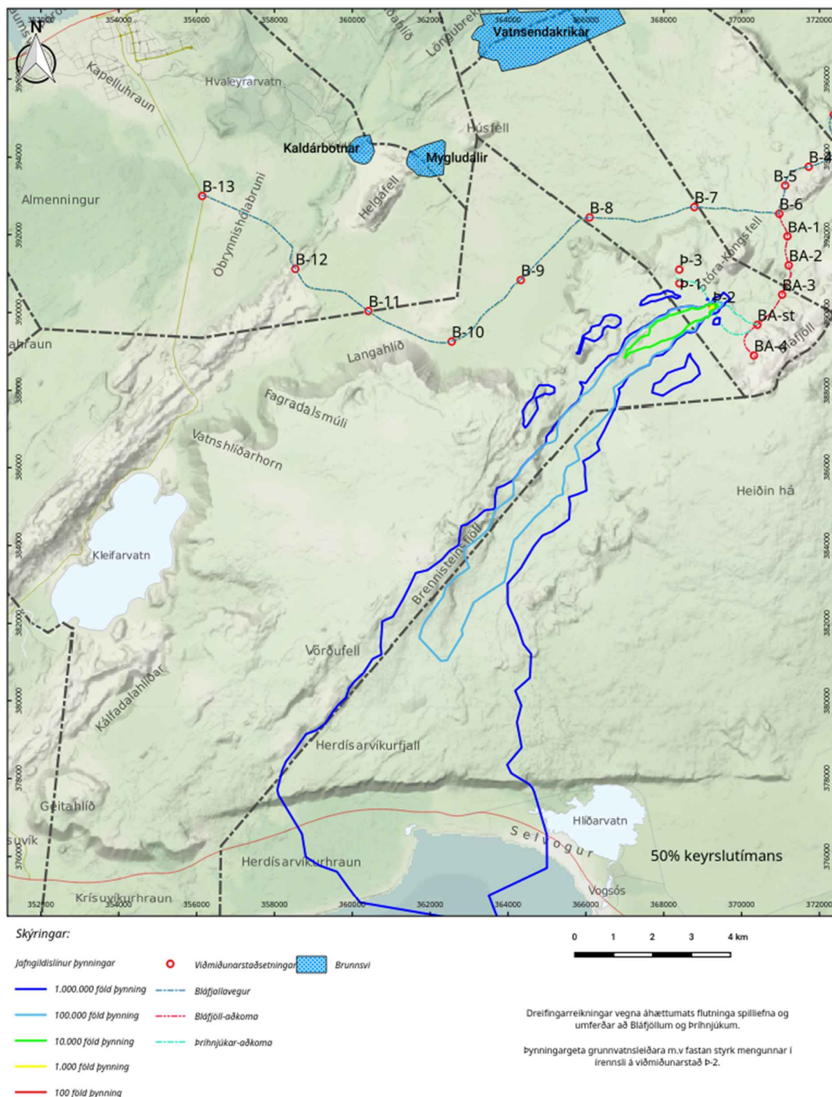
Mynd 88. Þynningargeta grunnvatnsleiðara miðað við fastan styrk mengunar í írennsli á viðmiðunarstað Þ-2. Breytileiki yfir 50% keyrslutímans.
