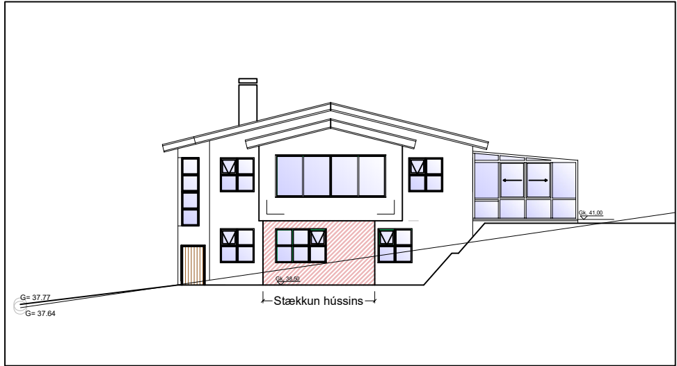
Skýringarmynd: Vesturhlið í mkv. 1:200
