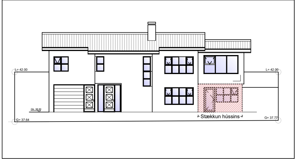
Skýringarmynd: Norðurhlið í mkv. 1:200
