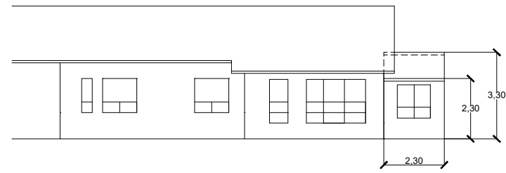
Útlit - Norðvestur Mælikvarði 1:100
