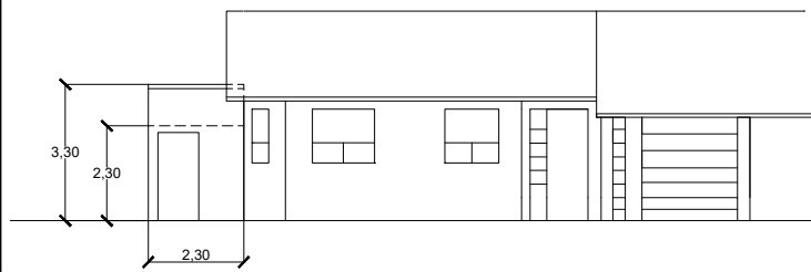
Útlit - Suðaustur Mælikvarði 1:100
