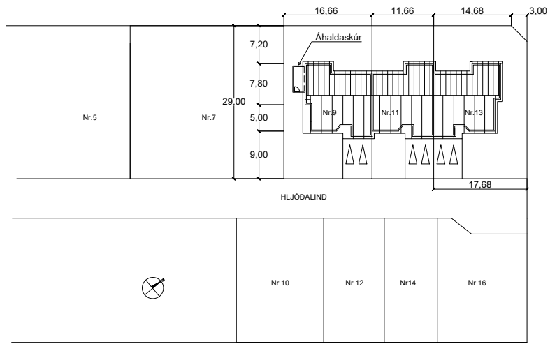
Afstöðumynd Mælikvarði 1 : 500
