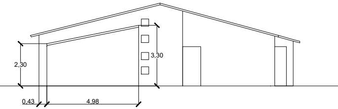
Útlit - Suðvestur Mælikvarði 1:100
