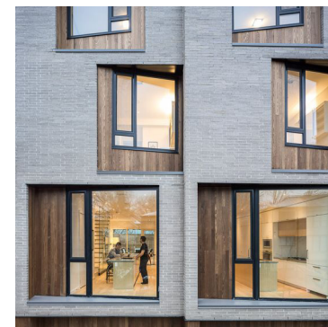
Dæmi uppbrót og stöllum á húshliðum og byggingarmassa til að draga úr umfangi bygginga og auka mannlegan skala. Hægt er að nota ólík byggingarefni til að auka fjölbreytileikann.
