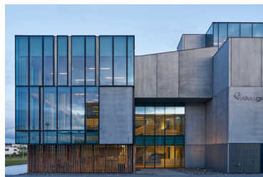
Dæmi um uppbrót á byggingarmassa og húshliðum með ólíkum hæðum, efnisvali og gluggasetningu
