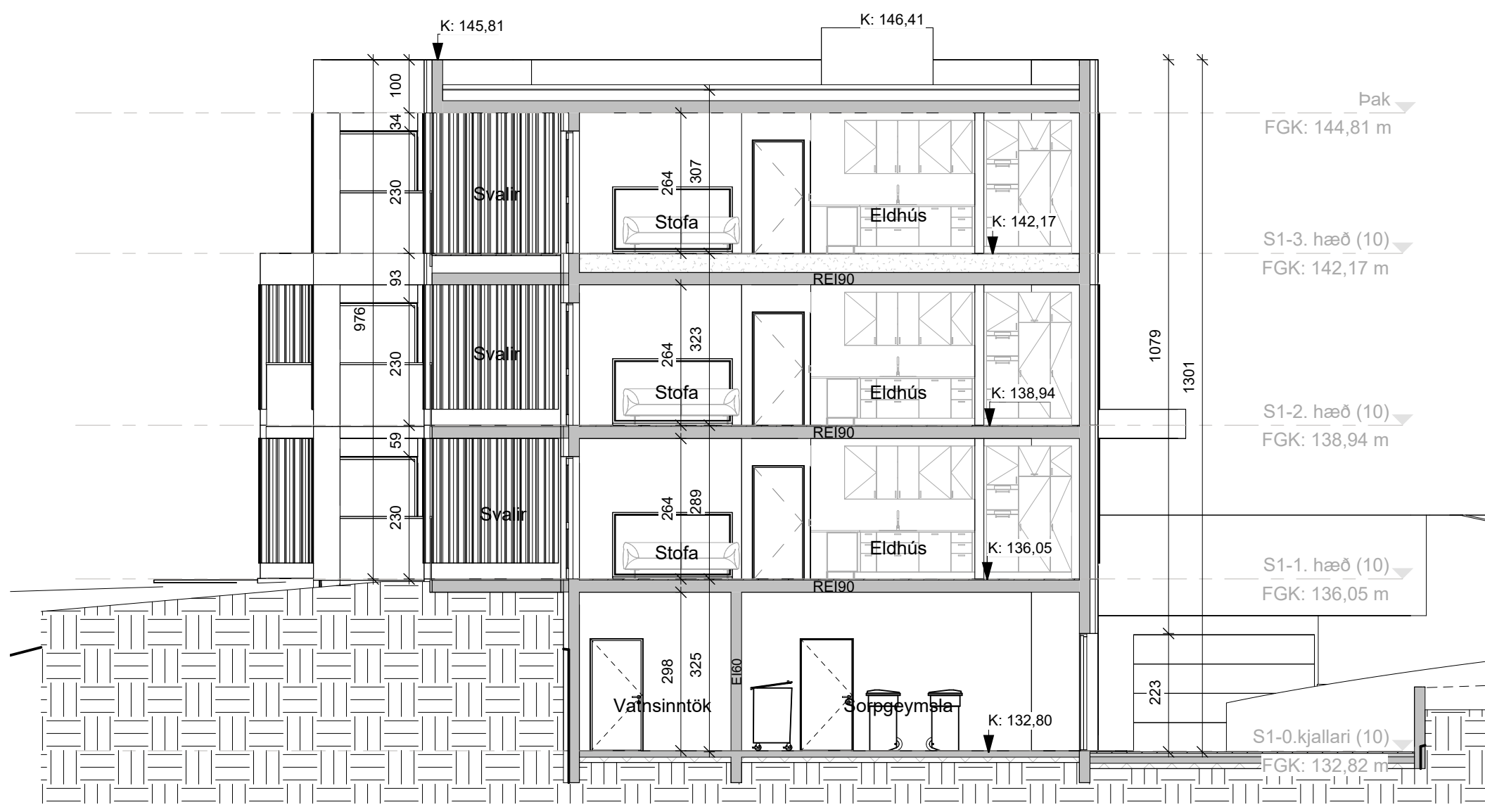
E-1 Sneiðingar E (S1) 1 : 100
