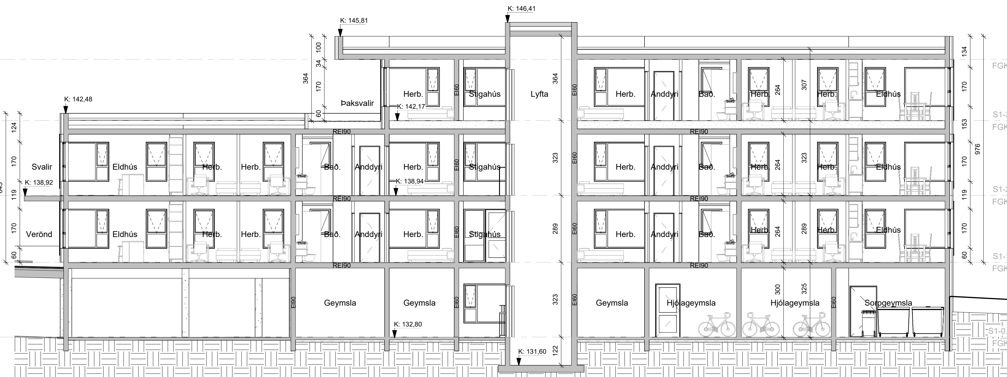
A-1 Sneiðing A (S1) 1 : 100
