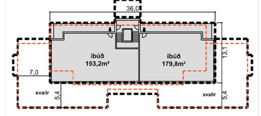
Fyrir breytingu: 4. hæð í mkv. 1:500
