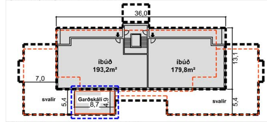
Eftir breytingu: 4. hæð í mkv. 1:500
