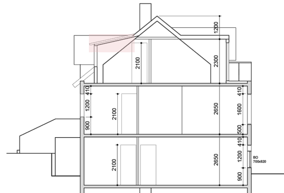
Skurðmynd
