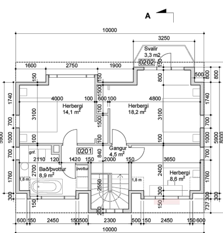
Grunnmynd rishæðar
