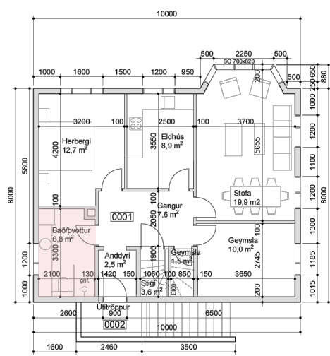
Grunnmynd kjallara
