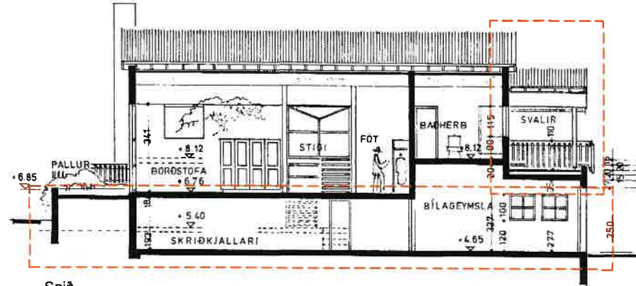
Snið
