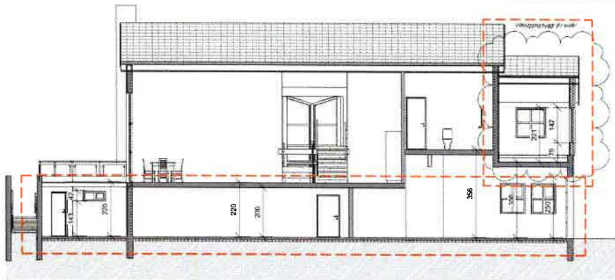
Snið
