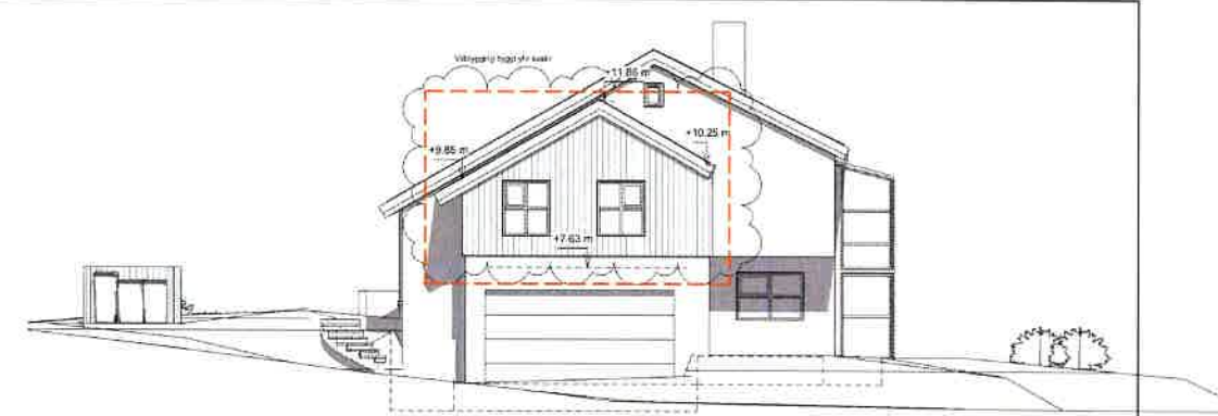
Útlit austur
