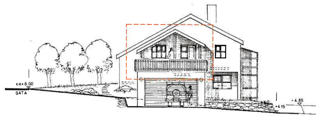
Útlit austur
