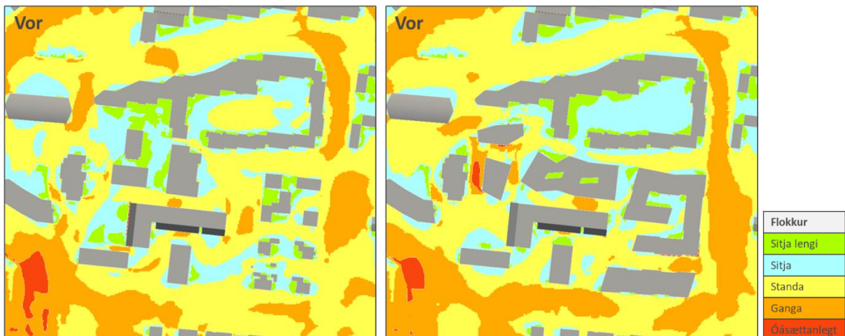
MYND 30 Tíðni vindhraða 2,5, 4, 6, og 8 m/s minni en 5% fyrir allar vindáttir yfir vor. Gildi fyrir vindhraðann eru samkvæmt City Lawson vindþæginda viðmiðinu. Viðmiðunargildið fyrir vindhraðann tilheyrir mismunandi athafnarflokkum. Kortið er unnið út frá hrágögnum um 10-mínútna vindhraða frá Veðurstofureitnum - 1475.
