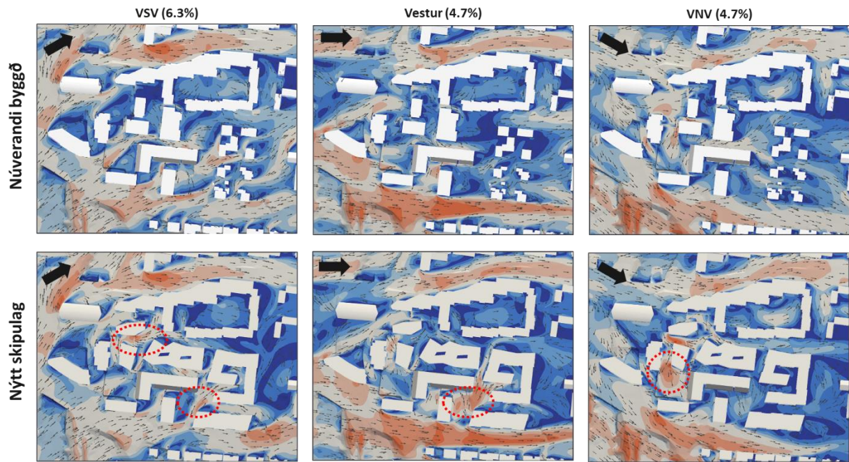
MYND 25 Meðalvindhraði sýndur á plani í 1,5m hæð yfir jörðu fyrir austanáttirnar. Prósenturnar við myndirnar sýna árlega tíðni vindáttanna byggð á gögnum frá veðurstöð á Veðurstofureitnum við Veðurstofu Íslands.
