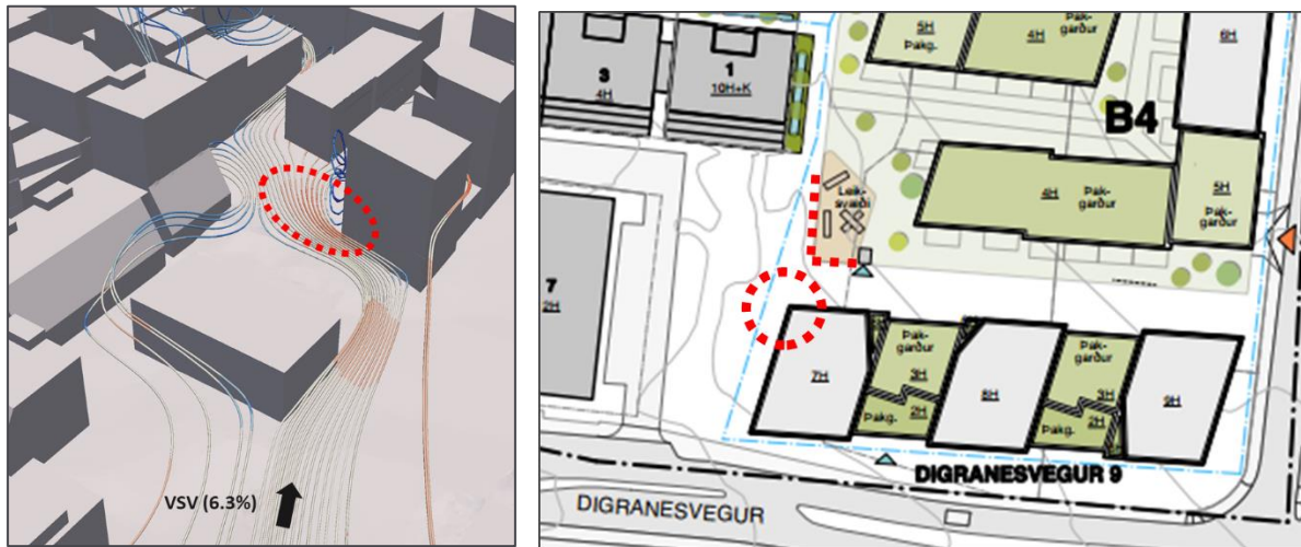
MYND 47 Vinstri; straumlínur sem sýna vind frá VSV-áttinni sem streymir inn sundið milli Digranesvegar 9 og Fannborgar 1 og að leiksvæðinu. Hægri; skipulagsuppdráttur af svæðinu ásamt merkingum þar sem ráðlagt er að staðsetja skjólmyndandi aðgerðir.
