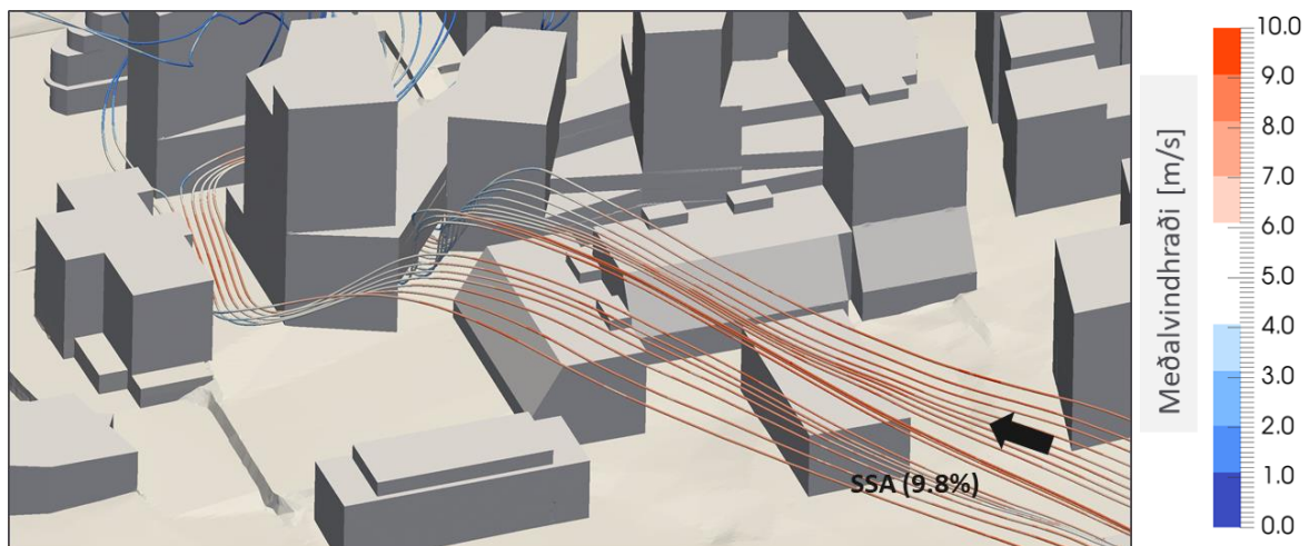
MYND 23 Straumlínur sem sýna flæði vinds úr SSA-áttinni sem streyma að Fannborg 2. Straumlínurnar eru litaðar með meðalvindhraða.
