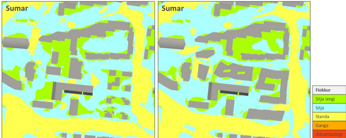
MYND 29 Tíðni vindhraða 2,5, 4, 6, og 8 m/s minni en 5% fyrir allar vindáttir yfir sumartímann. Gildi fyrir vindhraðann eru samkvæmt City Lawson vindþæginda viðmiðinu. Viðmiðunargildið fyrir vindhraðann tilheyrir mismunandi athafnarflokkum. Kortið er unnið út frá hrágögnum um 10-mínútna vindhraða frá Veðurstofureitnum - 1475.
