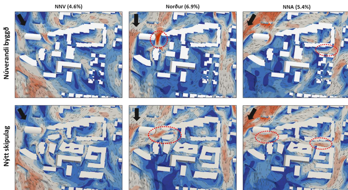
MYND 15 Meðalvindhraði sýndur á plani í 1,5m hæð yfir jörðu fyrir norðanáttirnar. Prósenturnar við myndirnar sýna árlega tíðni vindáttanna byggð á gögnum frá veðurstöð á Veðurstofureitnum við Veðurstofu Íslands.
