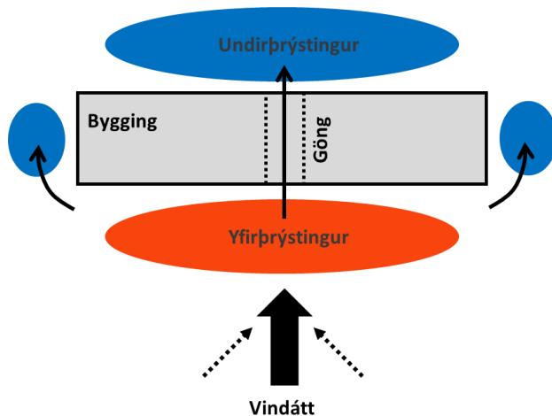
MYND 37 Skissa af þrýstingssvæðum í kringum byggingu þegar vindur lendir á langhlið hennar. Horft er á bygginguna að ofan.
