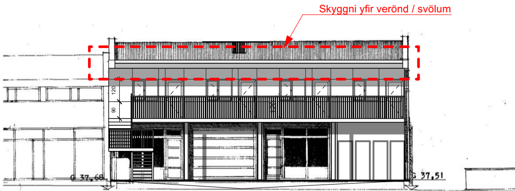
SUÐURHLIÐ EFTIR BREYTINGU
