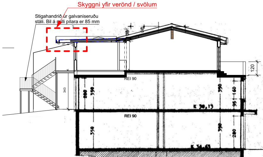
SNEIÐING EFTIR BREYTINGU
