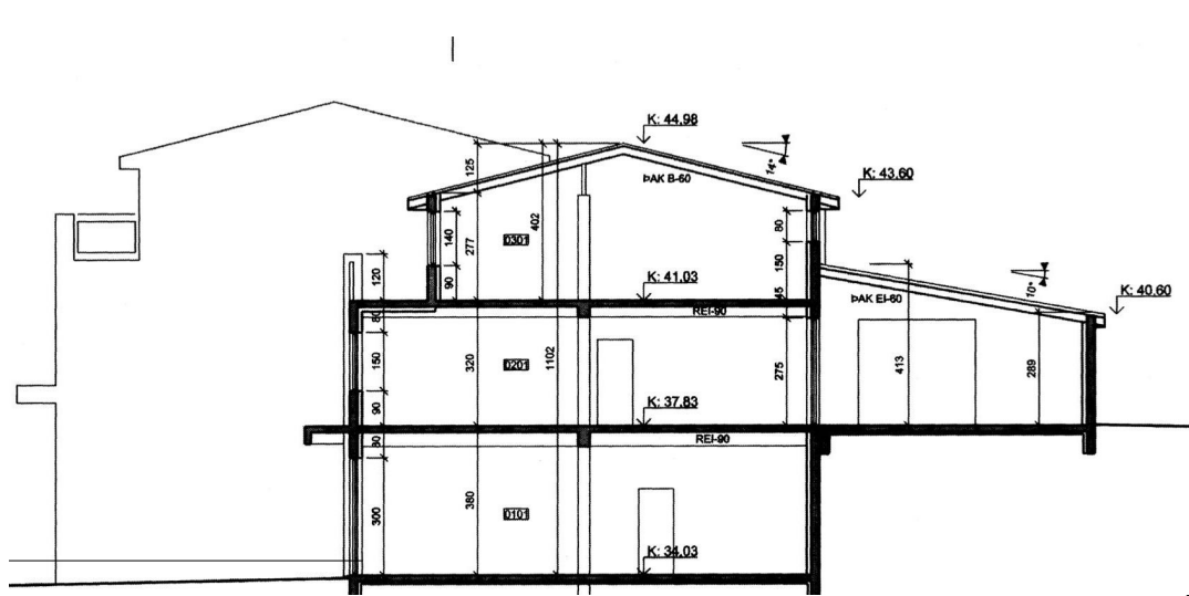
VESTURHLIÐ FYRIR BREYTINGU
