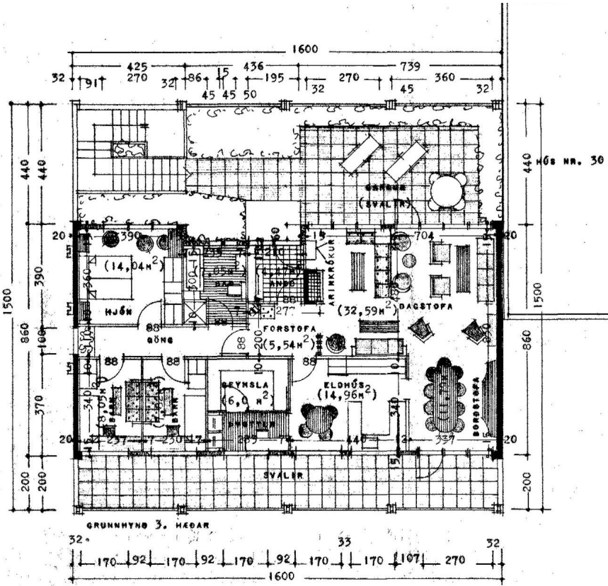
GRUNNMYND 3.HÆÐAR FYRIR BREYTINGU
