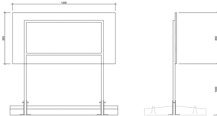
Mynd 7-1 Tillaga að undirstöðu fyrir upplýsingaskilti
