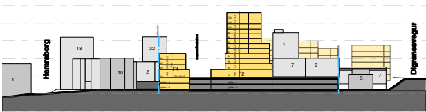
SKILMÁLARSNEIÐING D-D FANNBORG
