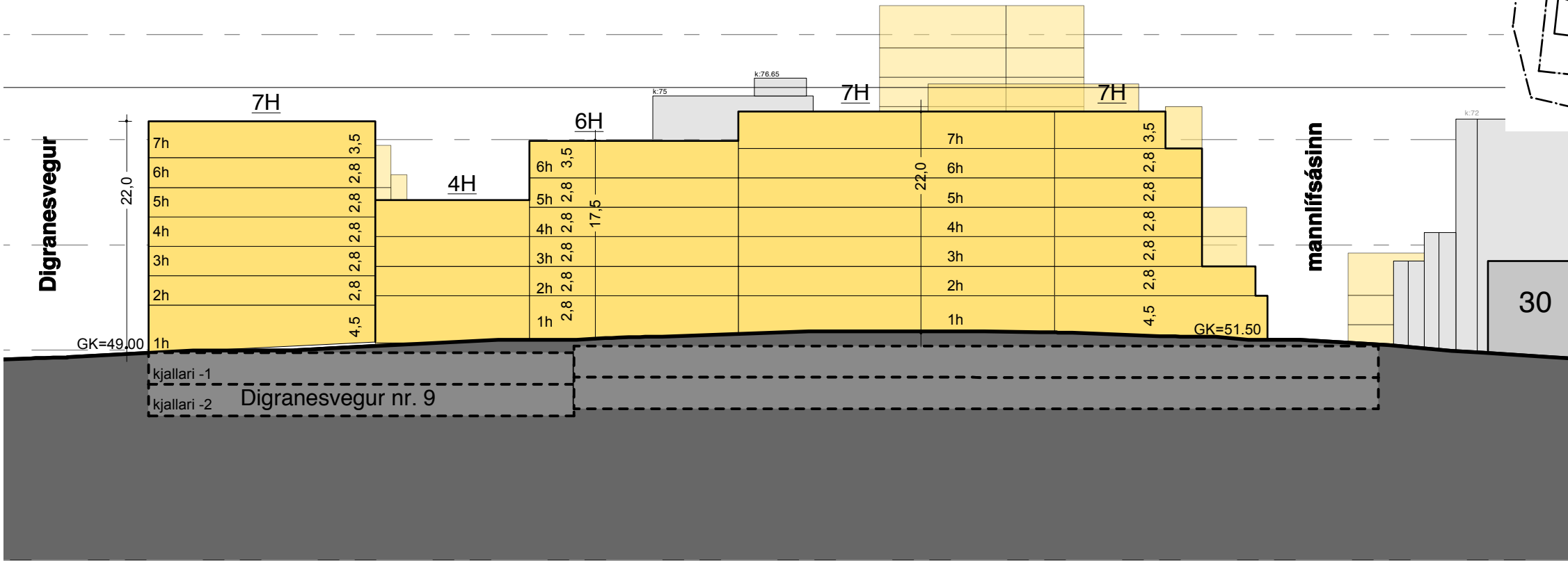
TRAÐARREITUR VESTARI Vallartröð
