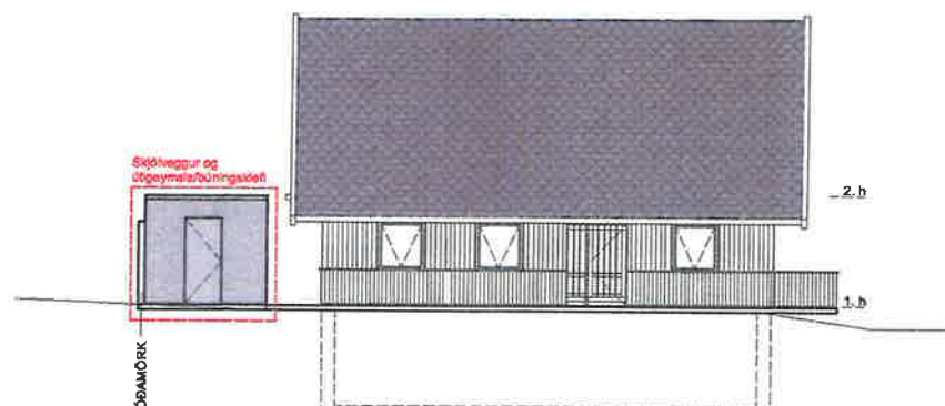
ÚTLIT SÚÐUR
