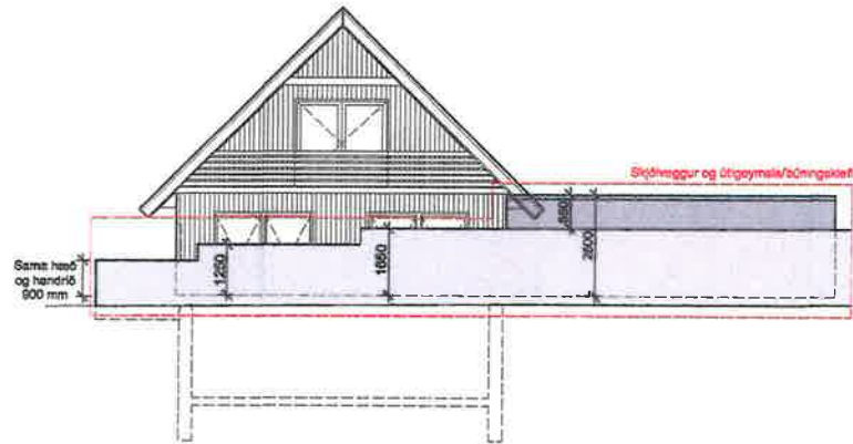
ÚTLIT VESTUR
