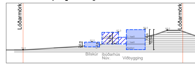
Tillaga - breytt deiliskipulag: Sneiðing A-A - Fornahvarf 10. Mkv. 1:1000
