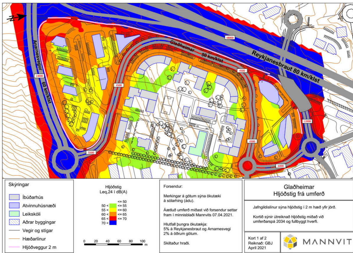
Mynd 5: Útreiknað hljóðstig í 2 m hæð á skipulagssvæðinu. Leikskóli og útivistarsvæði eru í húsagarði á miðju svæðinu.
