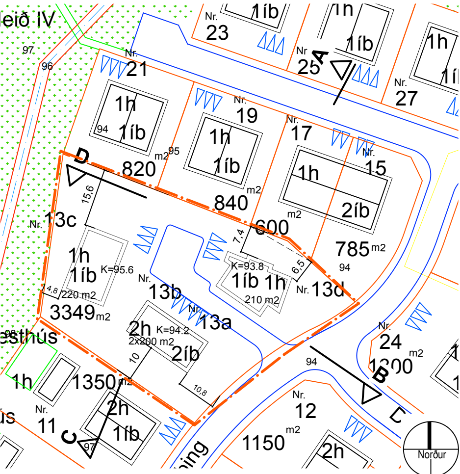
Tillaga að breyttu deiliskipulagi Dalaping 13a og b, c og d Mkv. 1:1000
