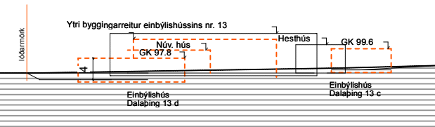
Skýringarmynd. Gildandi deili Sneiðmynd D-D í mkv. 1:500
