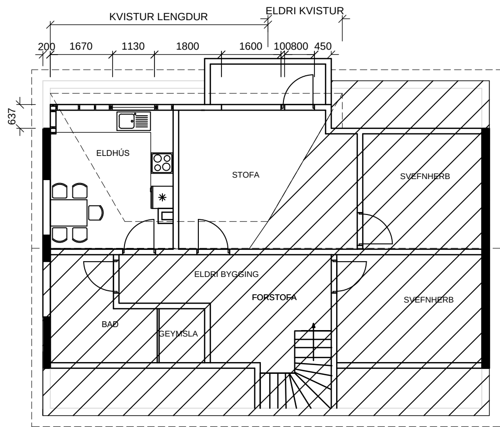
GRUNNMYND ÞAKHÆÐ, mkv.1:100
