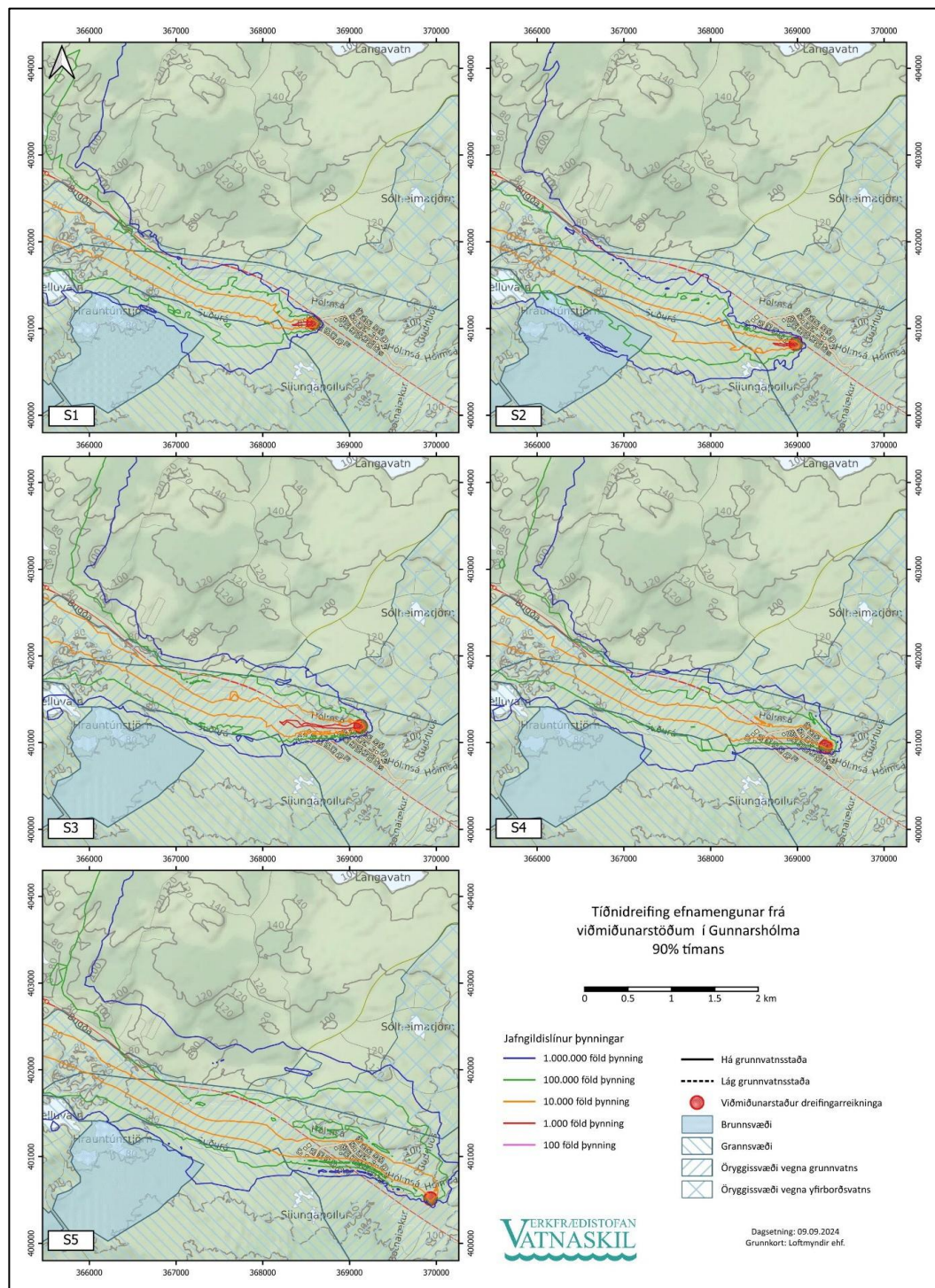
Mynd 6-4 Þýnningargeta grunnvatnsleiðara 90% tímans miðað við fastan styrk mengunar í írennsli á viðmiðunarstöðum S1 til S5 (Verkfræðistofan Vatnaskil, 2024a).
