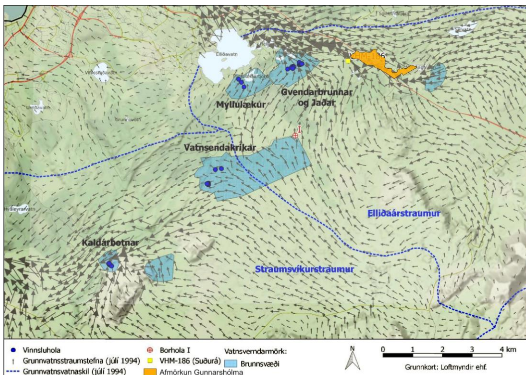
Mynd 3-5 Reiknað grunnvatnsrennsli í nágrenni helstu vatnsbóla á höfuðborgarsvæðinu (Verkfræðistofan Vatnaskil, 2018). Afmörkun Gunnarshólma er sýnd með appelsínugulur lit.
