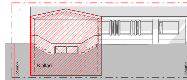
Skýringarmynd: Útlit vestur tillaga að breytingu 1:250
