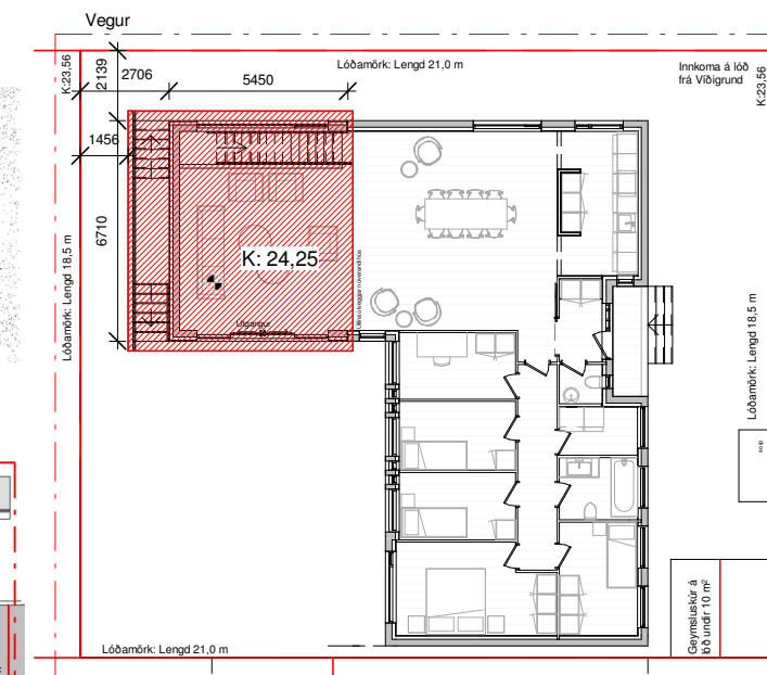
Skýringarmynd: Grunnmynd kjallari tillaga að breytingu 1:250
