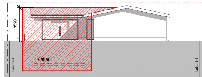
Skýringarmynd: Útlit suður tillaga að breytingu 1:250 Ekki til teikning af núverandi útlit suður.
