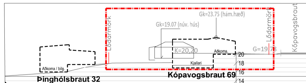
Skýringarmynd deiliskipulags sneiðing AA fyrir breytingu í mkv. 1:500
