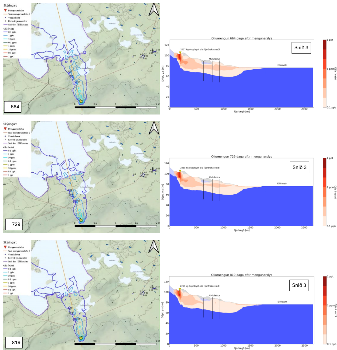
Mynd 55. Dreifing olíumengunar frá upptakastað 2, 664, 729 og 819 dögum eftir 5000 L mengunarslys.
