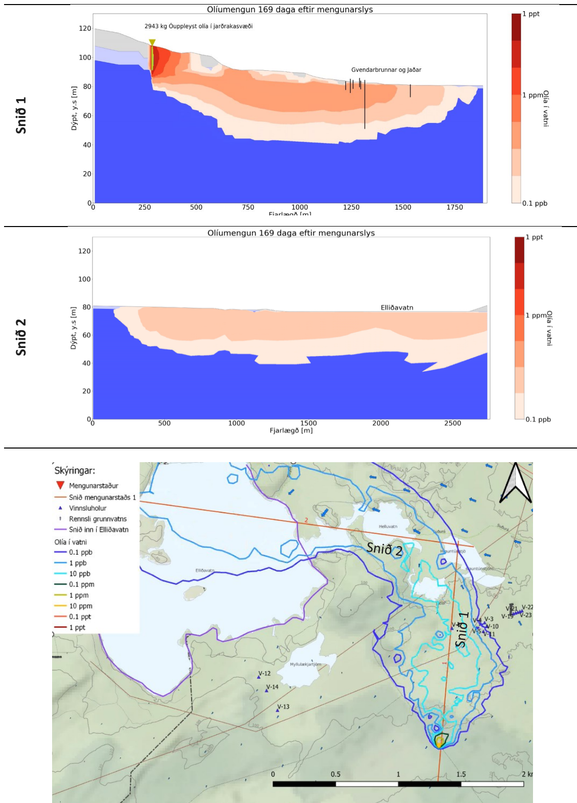
Mynd 32. Dreifing olíumengunar frá upptakastað 1, 169 dögum eftir mengunarslys þar sem 5000 L af olíu fara niður. Efst langsnið (Snið 1) eftir mengunarskýi frá upptakastað að vatnstökusvæðum í Heiðmörk. Fyrir miðju langsnið (Snið 2) frá Hrauntúnstjörn í Leitarhrauni að Elliðavatni. Neðst yfirlitsmynd yfir dreifingu mengunar frá upptakastað.
