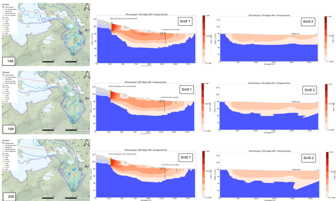
Mynd 37. Dreifing olíumengunar frá upptakastað 1, 149, 169 og 209 dögum eftir 5000 L mengunarslys.
