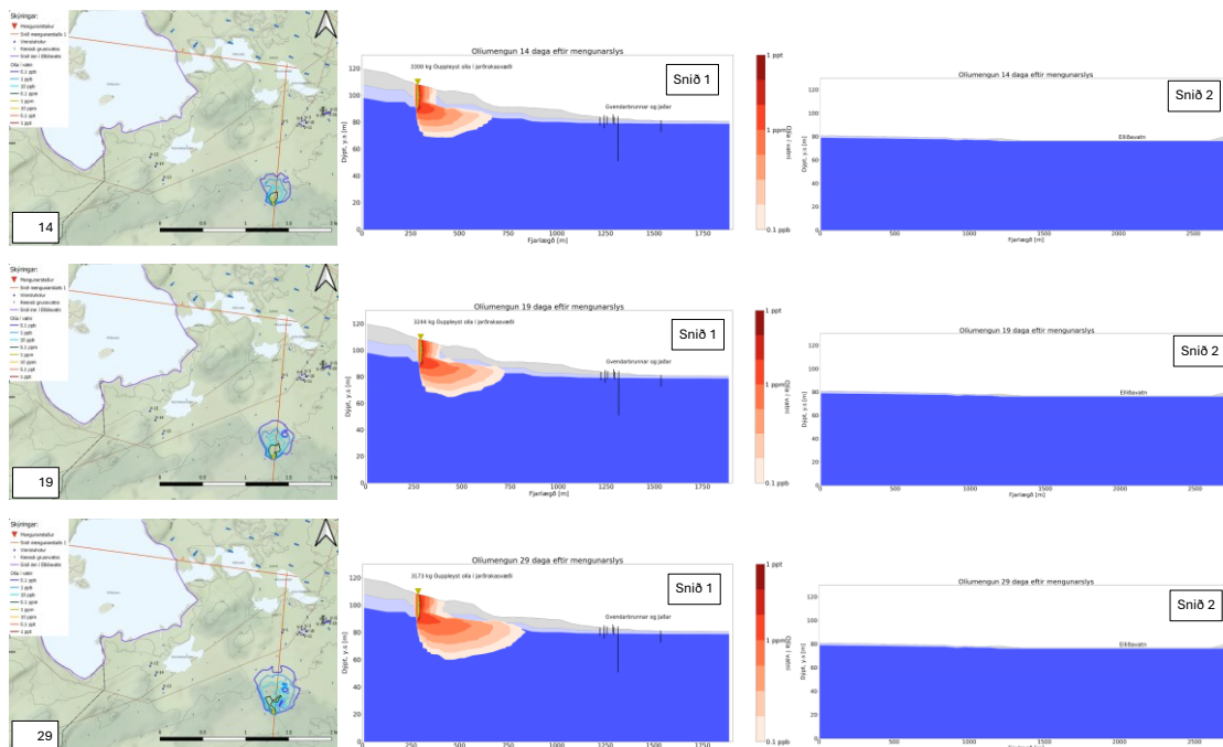
Mynd 35. Dreifing olíumengunar frá upptakastað 1, 14, 19 og 29 dögum eftir 5000 L mengunarslys.
