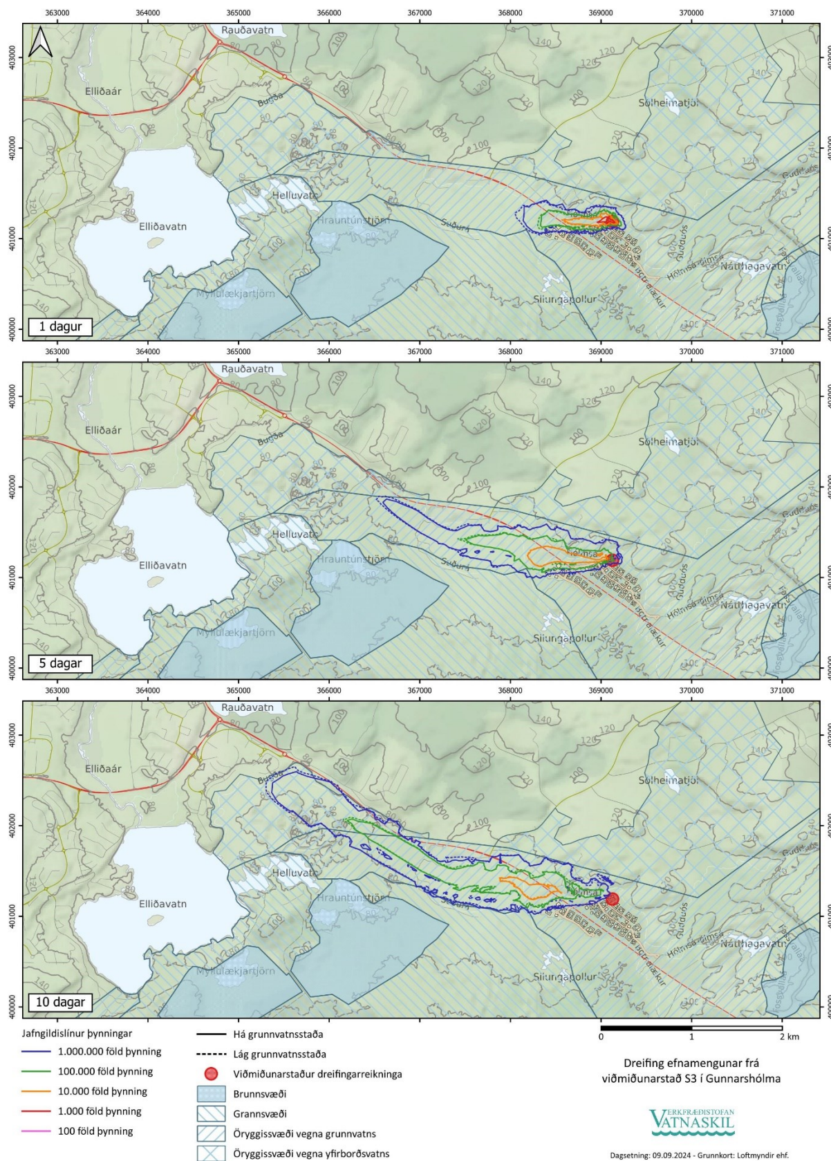
Mynd 15. Dreifing efnamengunar frá viðmiðunarstað S3 í Gunnarshólma eftir 1 dag, 5 og 10 daga eftir að mengunarefni berst til grunnvatnsborðs.
