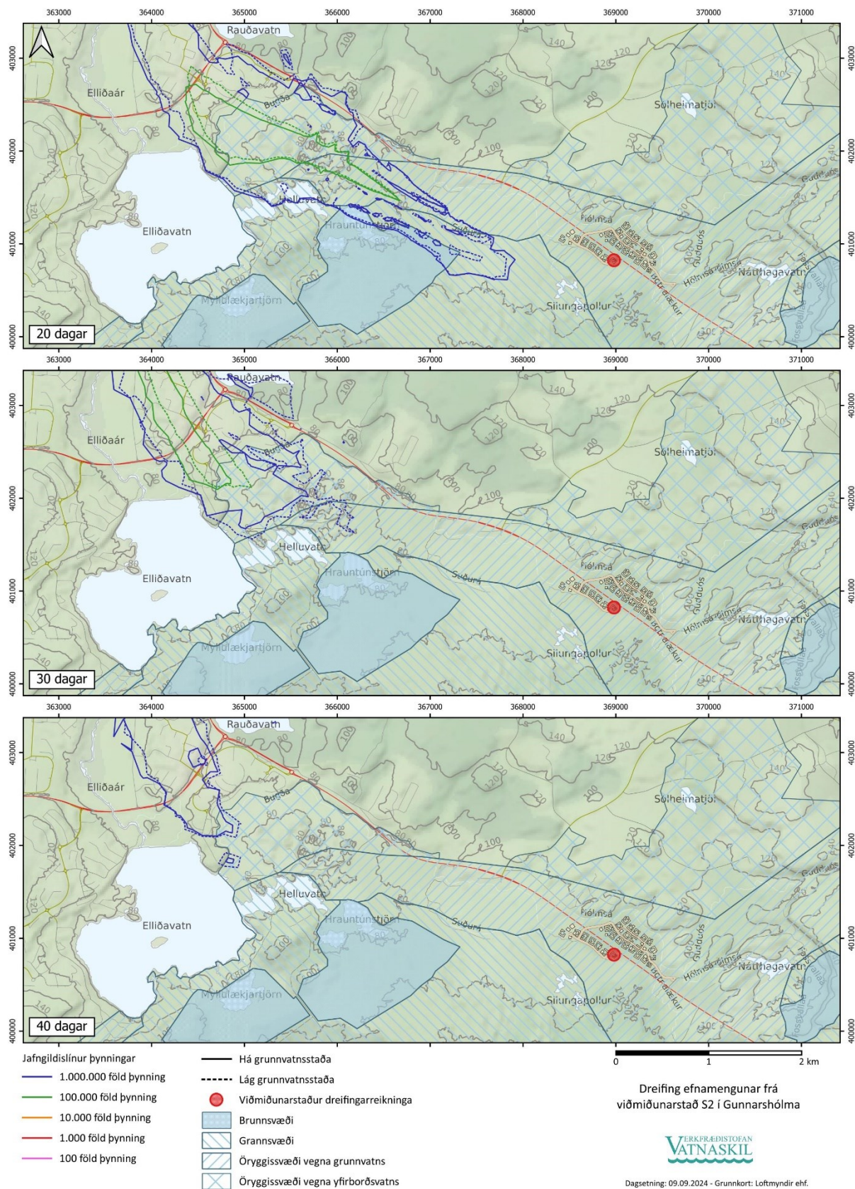
Mynd 14. Dreifing efnamengunar frá viðmiðunarstað S2 í Gunnarshólma eftir 20, 30 og 40 eftir að mengunarefni berst til grunnvatnsborðs.
