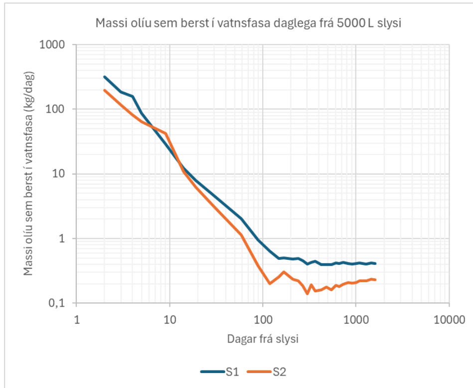
Mynd 29. Massi olíu sem berst í vatnsfasa daglega frá 5000 L olíuslysi á upptakastað 1 (S1) og upptakastað 2 (S2) í Heiðmörk.
