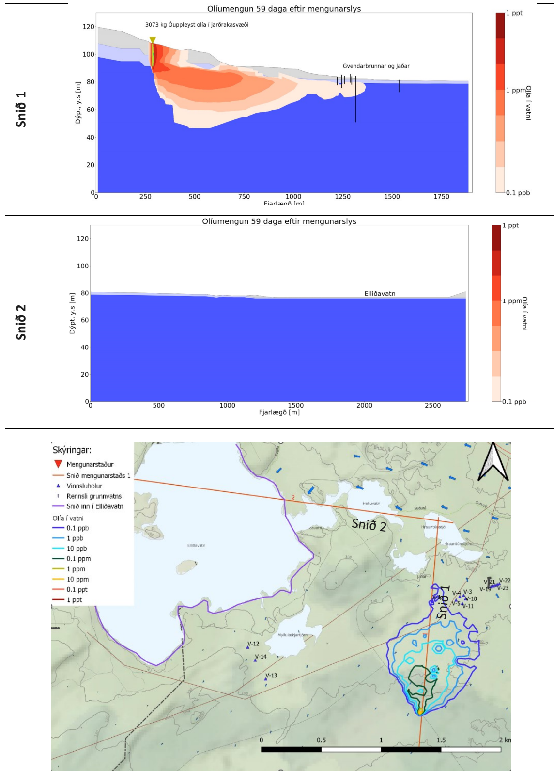
Mynd 31. Dreifing olíumengunar frá upptakastað 1, 59 dögum eftir slys þar sem 5000 L af olíu fara niður. Efst langsnið (Snið 1) eftir mengunarskýi frá upptakastað að vatnstökusvæðum í Heiðmörk. Fyrir miðju langsnið (Snið 2) frá Hrauntúnstjörn í Leitarhrauni að Elliðavatni. Neðst yfirlitsmynd yfir dreifingu mengunar frá upptakastað.
