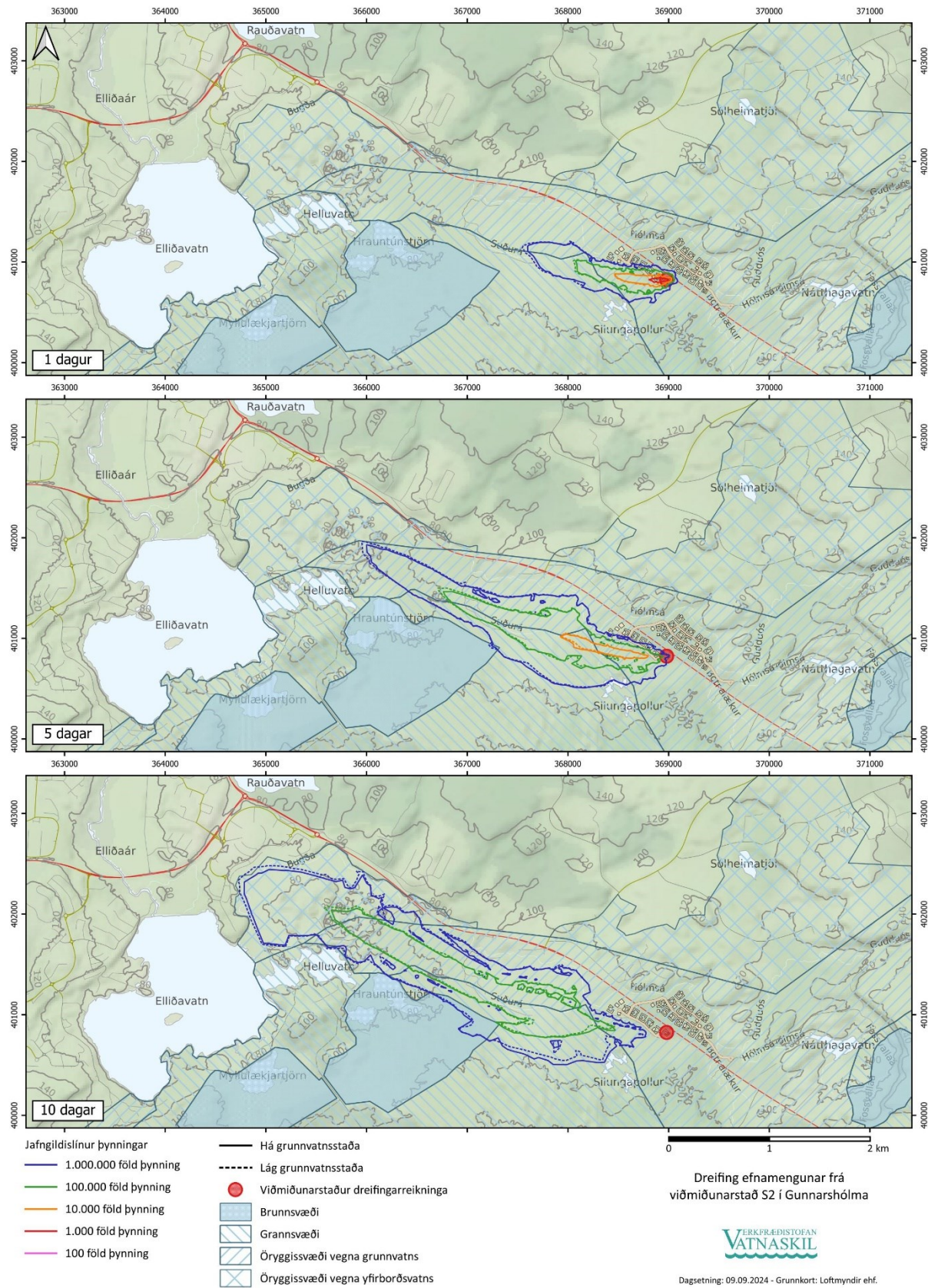
Mynd 13. Dreifing efnamengunar frá viðmiðunarstað S2 í Gunnarshólma eftir 1 dag, 5 og 10 daga eftir að mengunarefni berst til grunnvatnsborðs.
