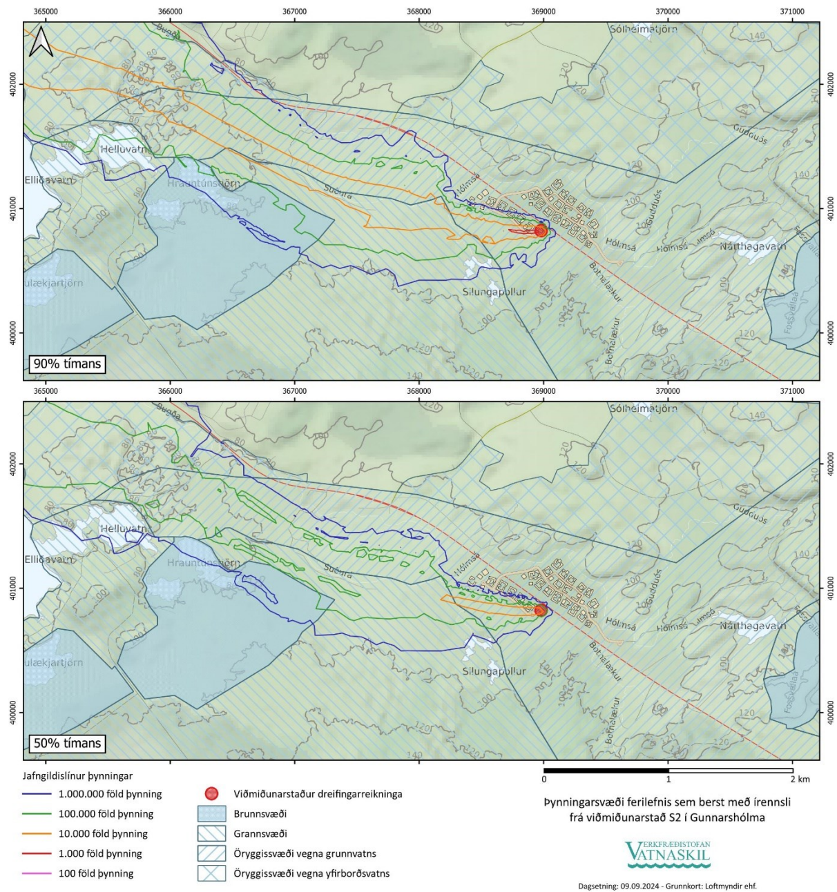
Mynd 22. Þýnningargeta grunnvatnsleiðara 90% tímans (efri mynd) og 50% tímans (neðri mynd) miðað við fastan styrk mengunar í írennsli á viðmiðunarstað S2.
