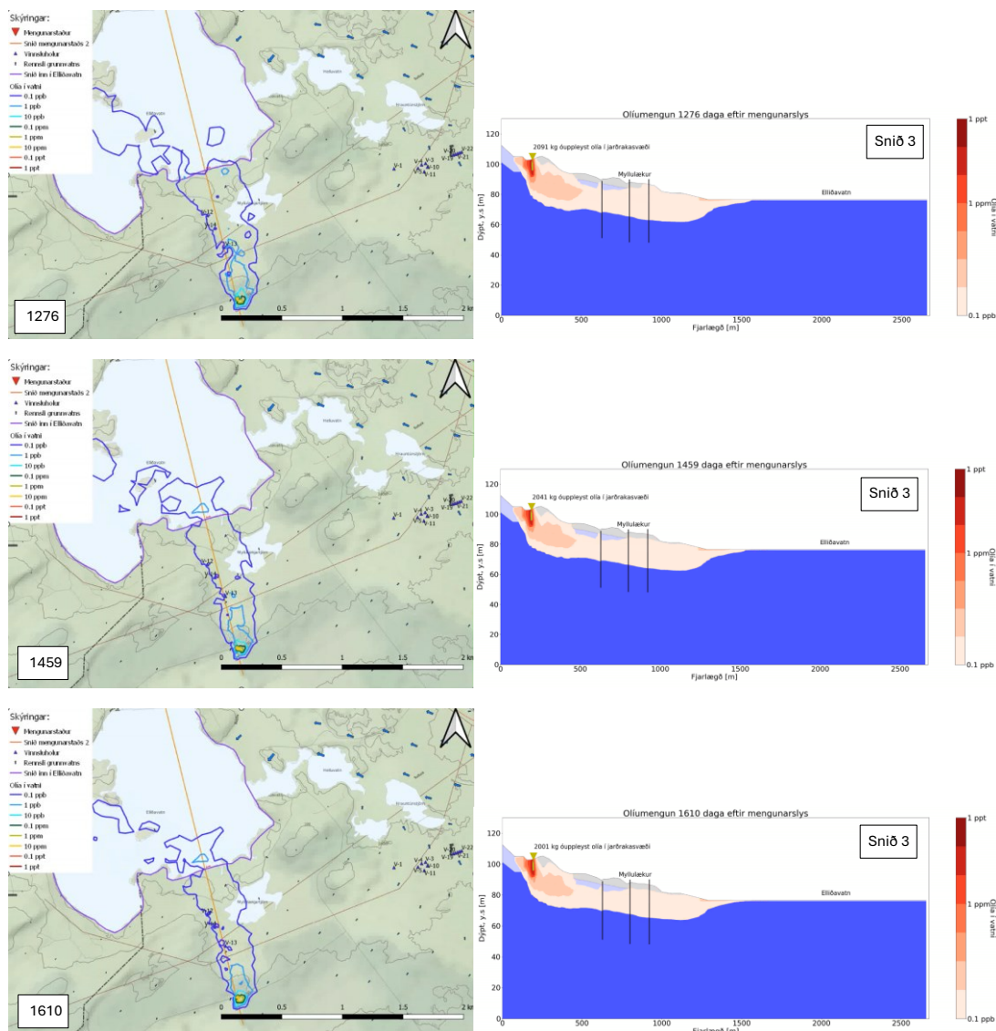
Mynd 57. Dreifing olíumengunar frá upptakastað 2, 1276, 1459 og 1610 dögum eftir 5000 L mengunarslys.
