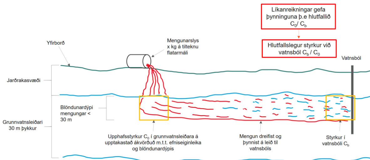
Mynd 9. Skematísk mynd til útskýringar á tulkun dreifingarreikninga m.t.t. mengunarslyss.
