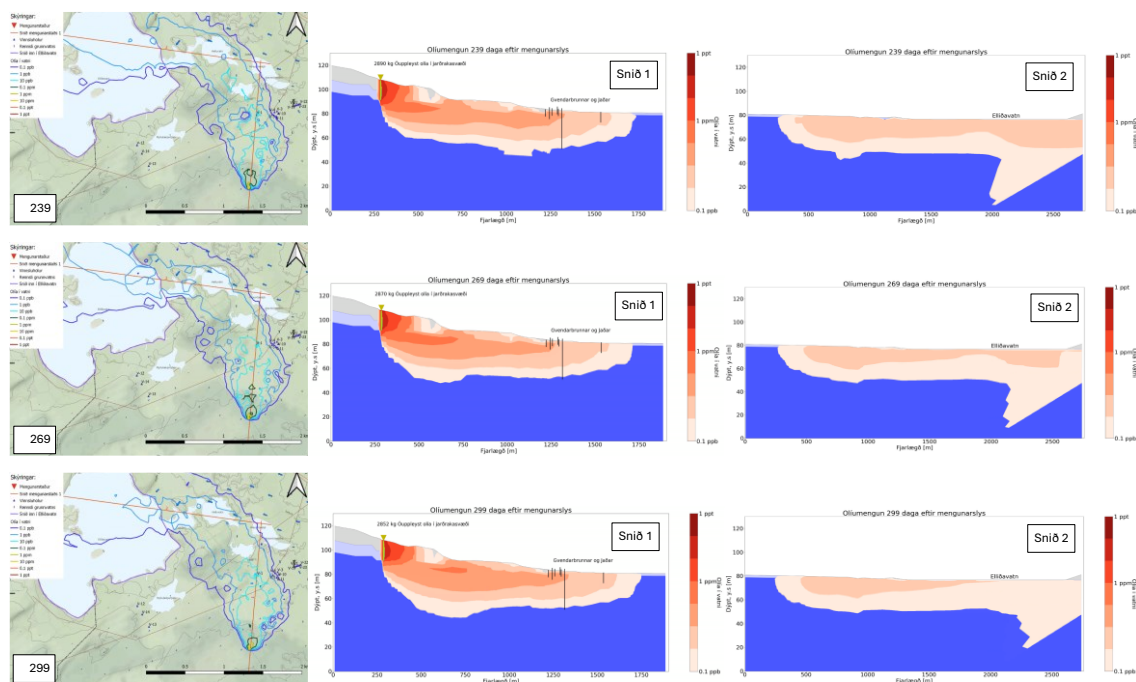
Mynd 38. Dreifing olíumengunar frá upptakstað 1, 239, 269 og 299 dögum eftir 5000 L mengunarslyss.
