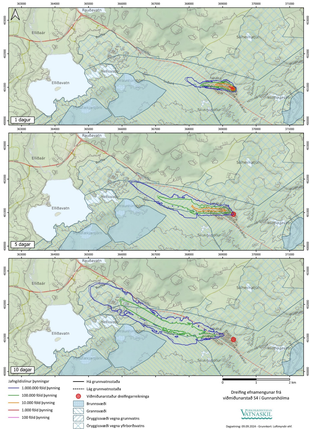
Mynd 17. Dreifing efnamengunar frá viðmiðunarstað S4 í Gunnarshólma eftir 1 dag, 5 og 10 daga eftir að mengunarefni berst til grunnvatnsborðs.
