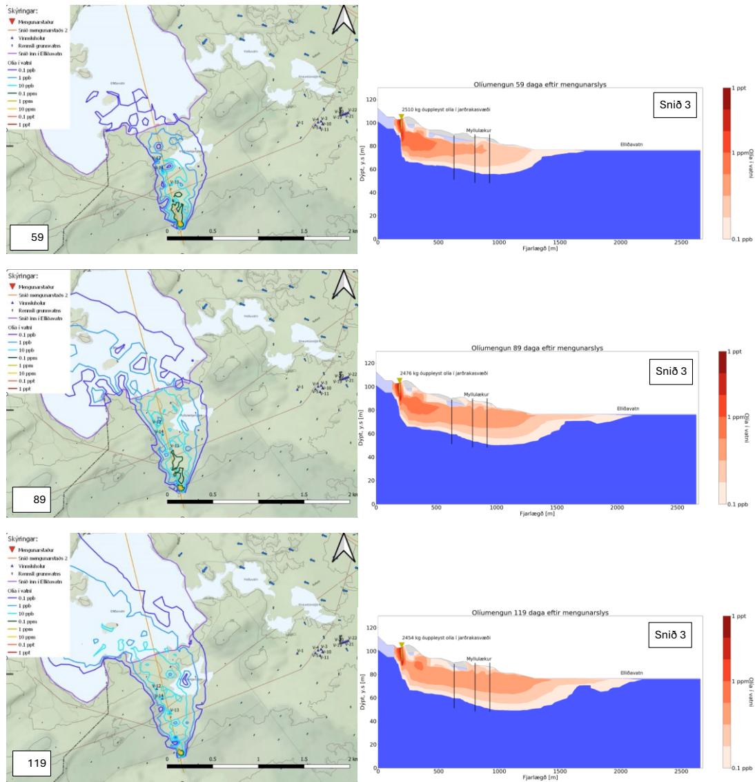
Mynd 50. Dreifing olíumengunar frá upptakastað 2, 59, 89 og 119 dögum eftir 5000 L mengunarslys.
