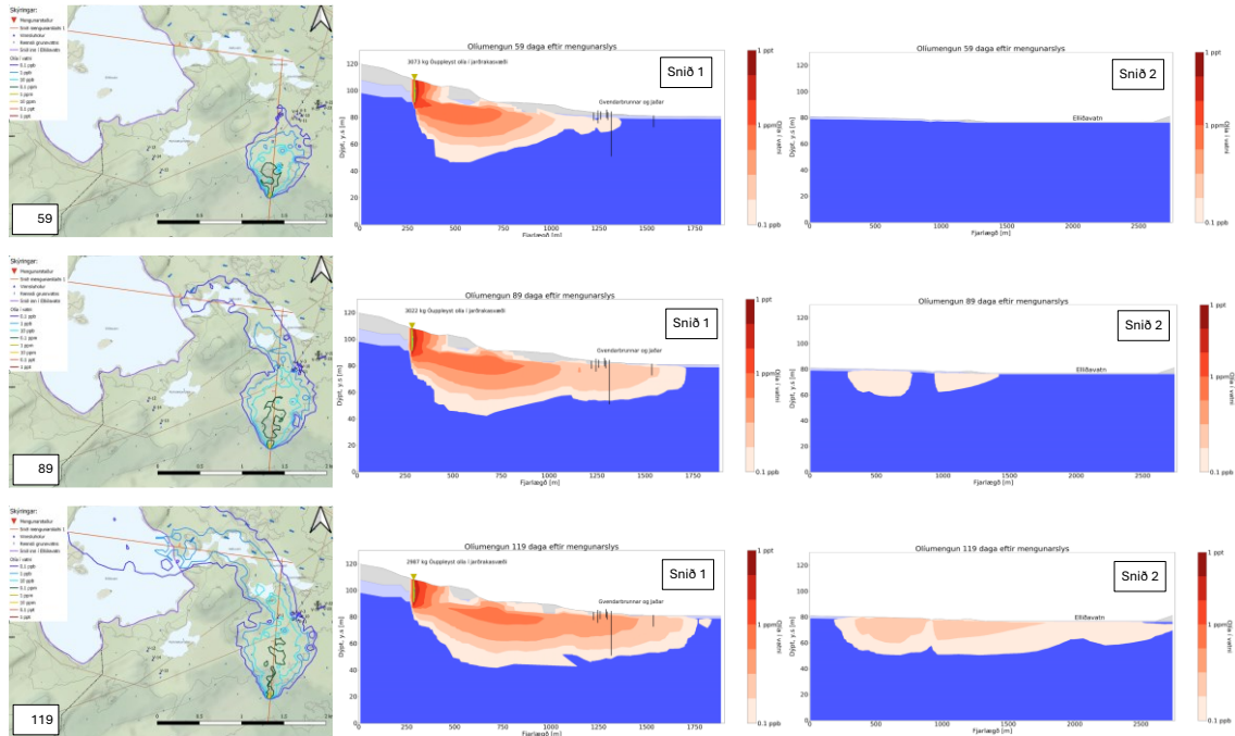
Mynd 36. Dreifing olíumengunar frá upptakastað 1, 59, 89 og 119 dögum eftir 5000 L mengunarslys.
