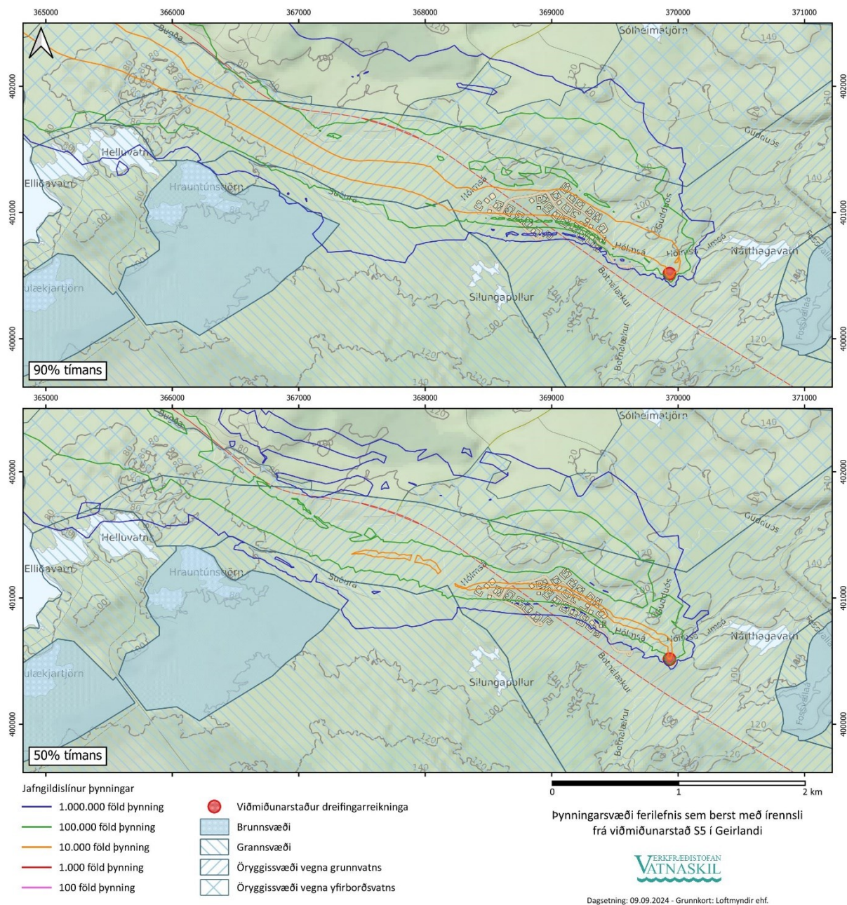
Mynd 25. Þýnningargeta grunnvatnsleiðara 90% tímans (efri mynd) og 50% tímans (neðri mynd) miðað við fastan styrk mengunar í írennsli á viðmiðunarstað S5.
