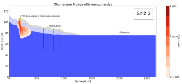
Mynd 48. Dreifing olíumengunar frá upptakastað 2, 1, 4 og 9 dögum eftir 5000 L mengunarslys.
