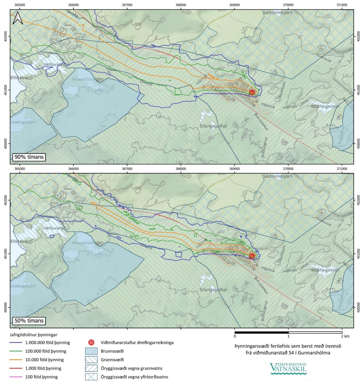
Mynd 24. Þýnningargeta grunnvatnsleiðara 90% tímans (efri mynd) og 50% tímans (neðri mynd) miðað við fastan styrk mengunar í írennsli á viðmiðunarstað S4.
