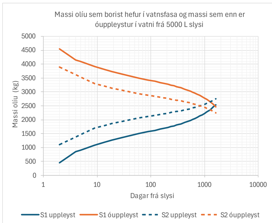
Mynd 30. Massi olíu sem borist hefur í grunnvatn og massi sem enn er óuppleystur í vatni frá 5000 L olíuslysi á upptakastað 1 (S1) og upptakastað 2 (S2) í Heiðmörk.
