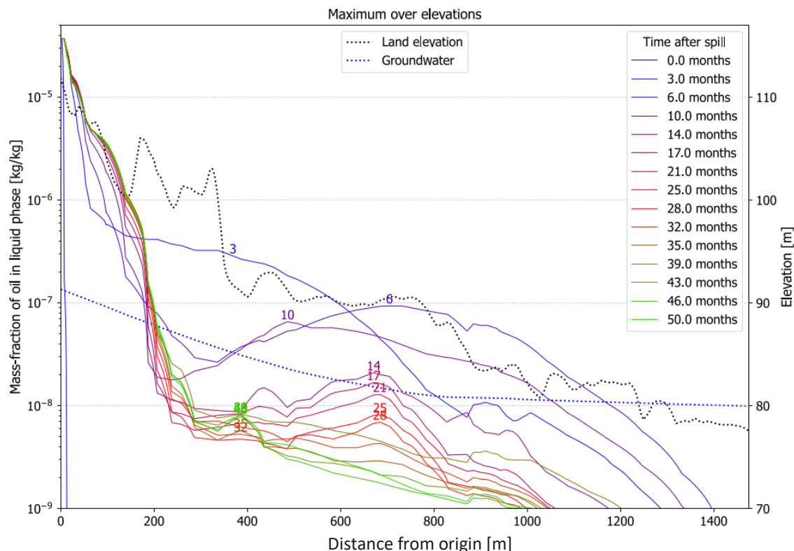
Mynd 44. Þróun á reiknuðum mesta styrk olíu í grunnvatni eftir sniði 1 milli upptakastaðar 1 (0 m fjarlægð) og vatnsbólsvæðis (930 m fjarlægð) fyrir 5000 L mengunarslys og valda mánuði liðna frá slysi.
