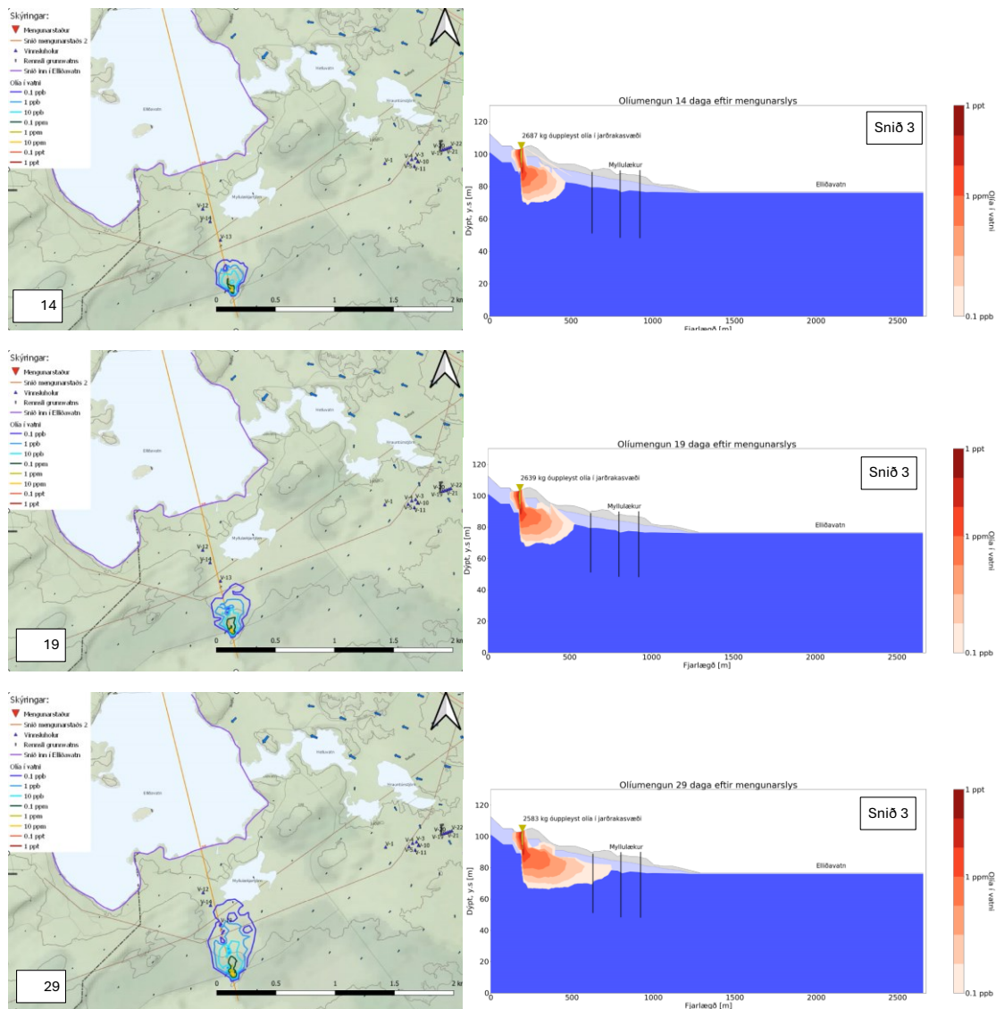
Mynd 49. Dreifing olíumengunar frá upptakastað 2, 14, 19 og 29 dögum eftir 5000 L mengunarslys.
