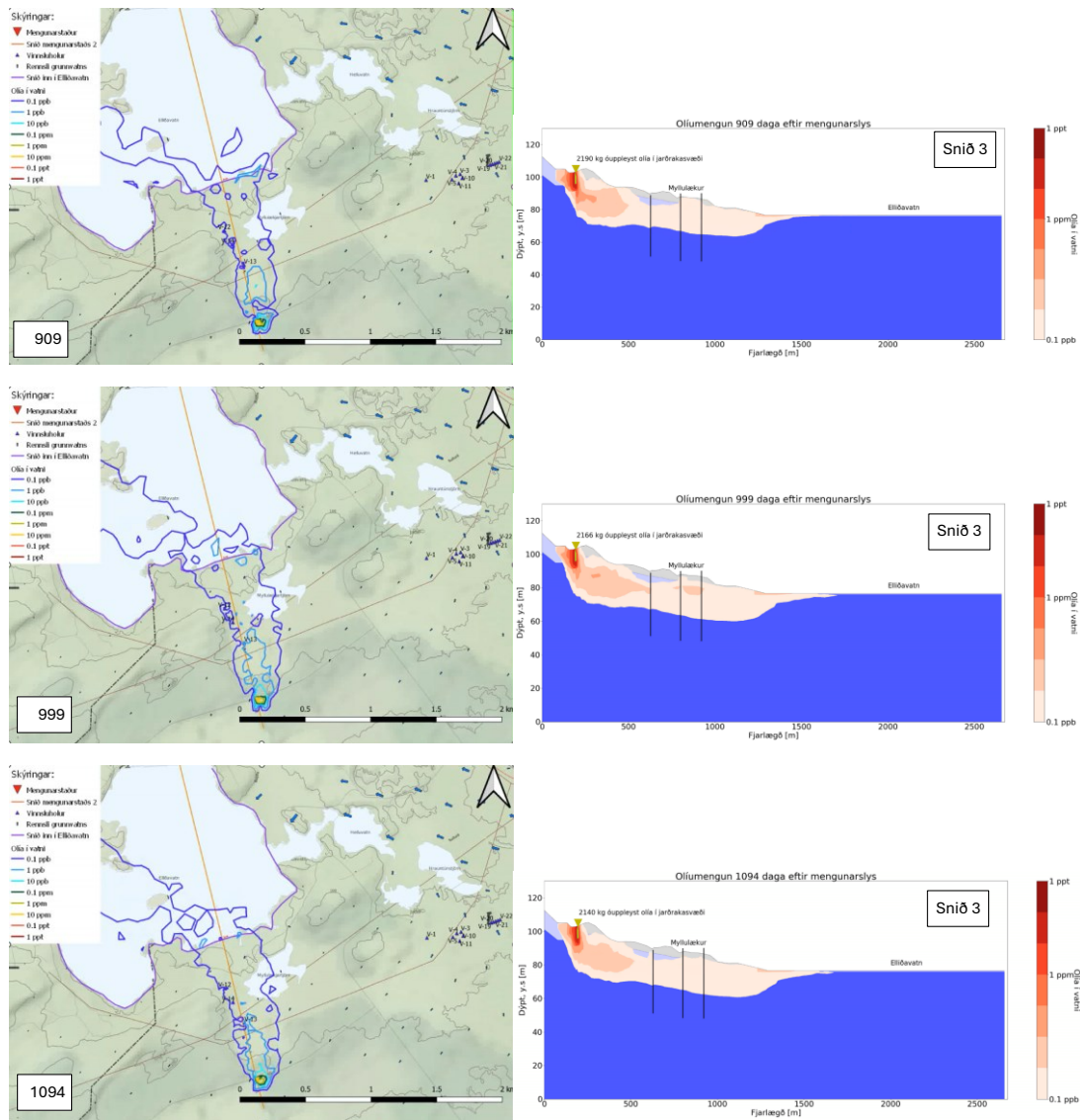
Mynd 56. Dreifing olíumengunar frá stað upptakastað setningu 2, 909, 999 og 1094 dögum eftir 5000 L mengunarslys.
