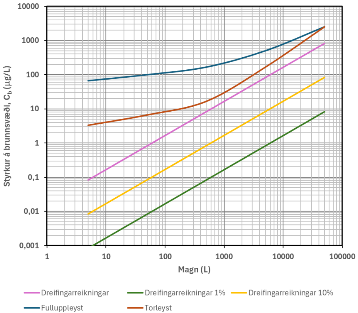
Mynd 67. Metinn mesti styrkur á brunnsvæði fyrir mismunandi stærði mengunarslysa út frá dreifingarreikningum (atvikareikningum) og varfærunum viðmiðum um styrk fulluppleystra og torleystra efna.
