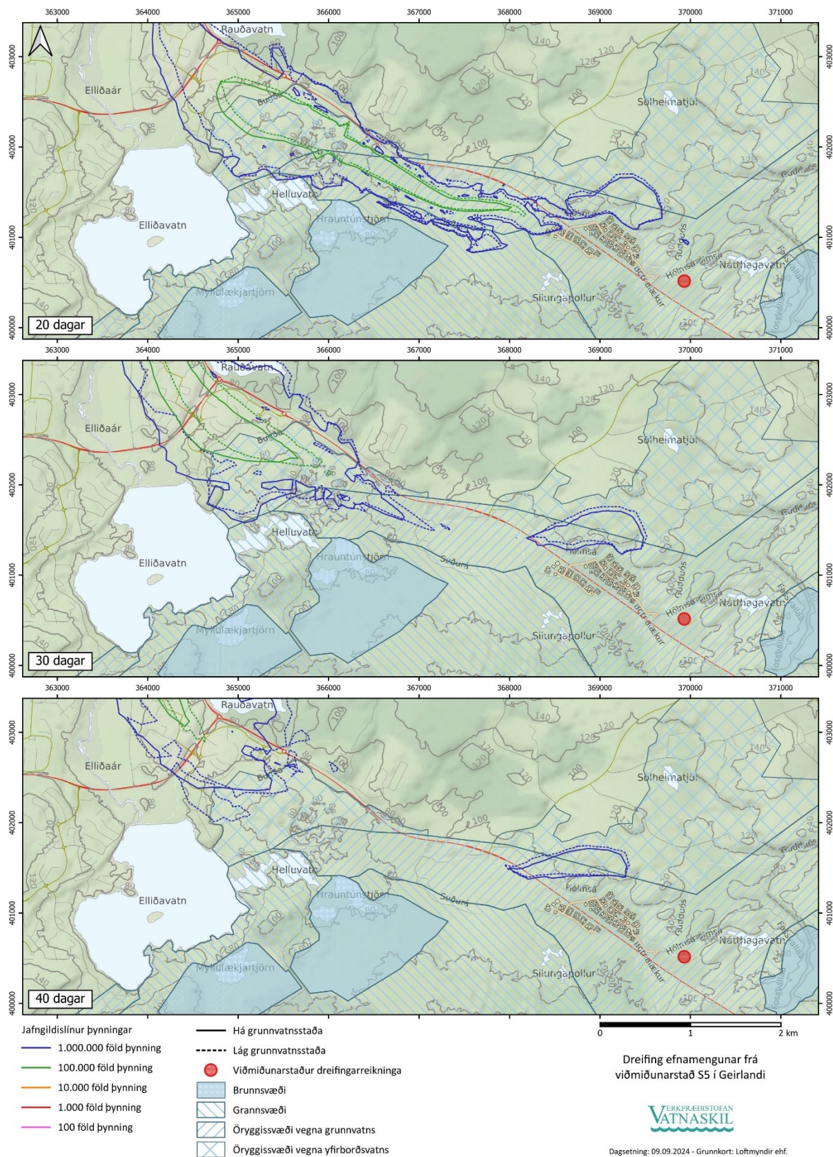
Mynd 20. Dreifing efnamengunar frá viðmiðunarstað S5 í Geirlandi eftir 20, 30 og 40 daga eftir að mengunarefni berst til grunnvatnsborðs.
