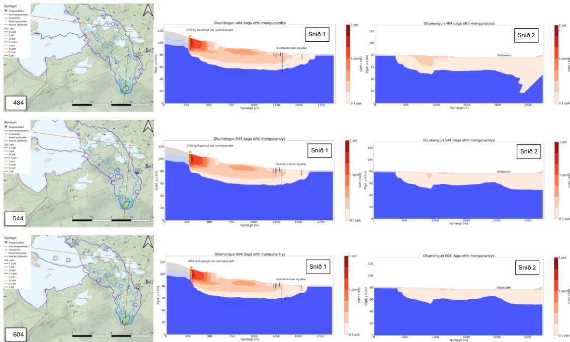
Mynd 40. Dreifing olíumengunar frá upptakastað 1, 484, 544 og 604 dögum eftir 5000 L mengunarslys.
