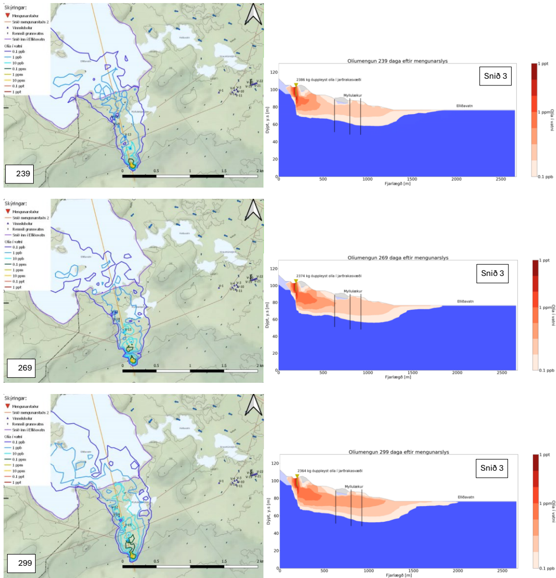
Mynd 52. Dreifing olíumengunar frá upptakastað 2, 239, 269 og 299 dögum eftir 5000 L mengunarslys.
