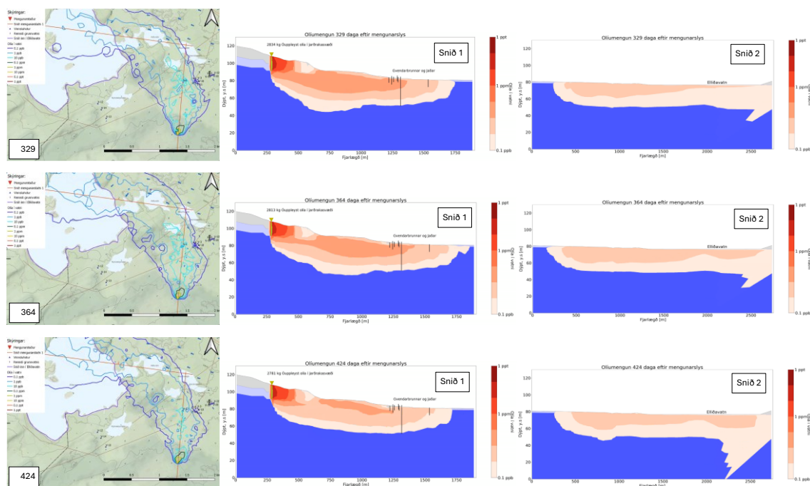
Mynd 39. Dreifing olíumengunar frá upptakstað 1, 329, 364 og 424 dögum eftir 5000 L mengunarslyss.
