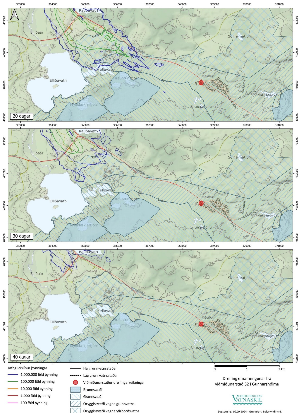
Mynd 12. Dreifing efnamengunar frá viðmiðunarstað S1 í Gunnarshólma eftir 20, 30 og 40 daga eftir að mengunarefni berst til grunnvatnsborðs.
