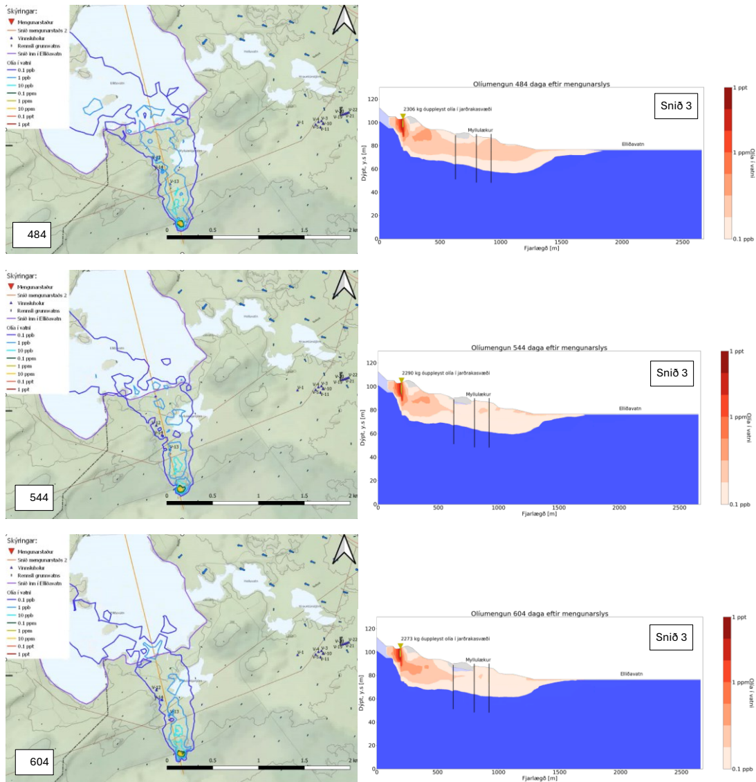
Mynd 54. Dreifing olíumengunar frá upptakastað 2, 484, 544 og 604 dögum eftir 5000 L mengunarslys.
