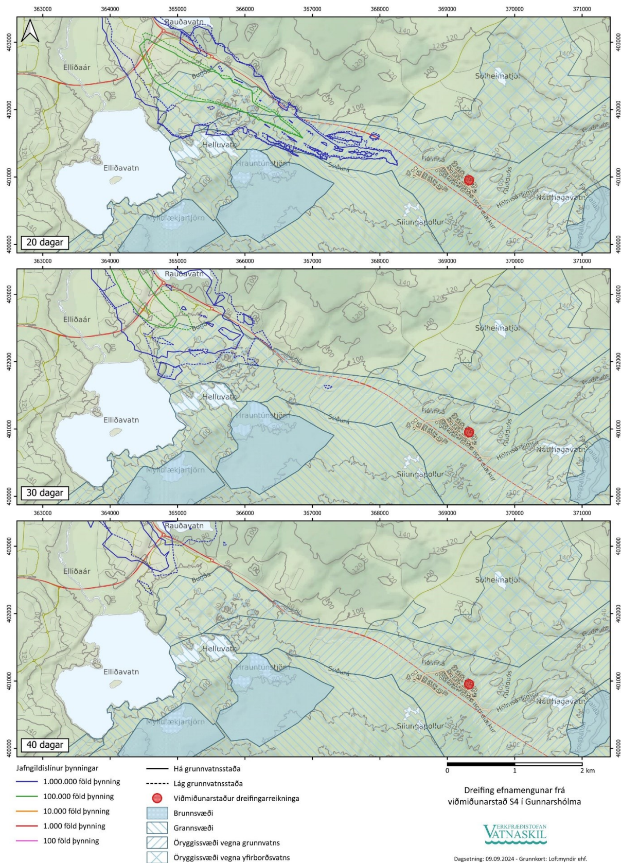
Mynd 18. Dreifing efnamengunar frá viðmiðunarstað S4 í Gunnarshólma eftir 20, 30 og 40 daga eftir að mengunarefni berst til grunnvatnsborðs.
