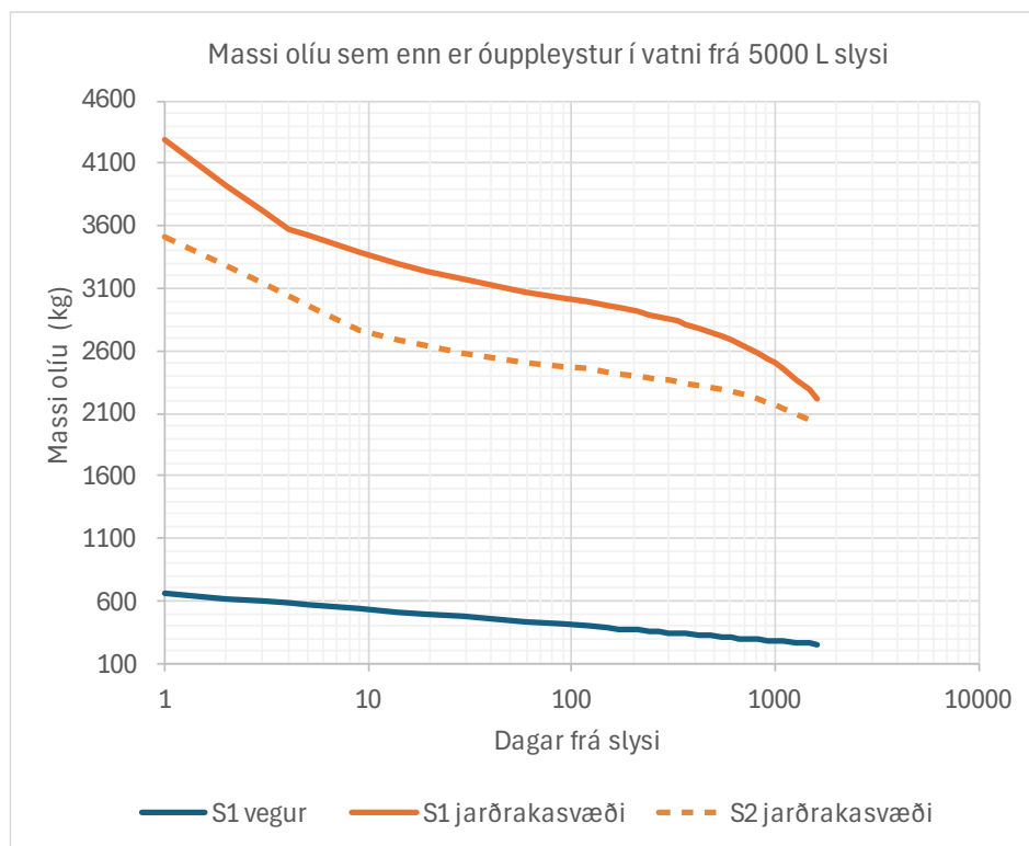
Mynd 28. Massi olíu sem enn er óuppleystur í vatnsfasa á hverjum tímapunkti frá 5000 L olíuslysi, fyrir vegstæði og jarðrakasvæði á upptakastað 1 (S1) og jarðrakasvæði á upptakastað 2 (S2) í Heiðmörk.
