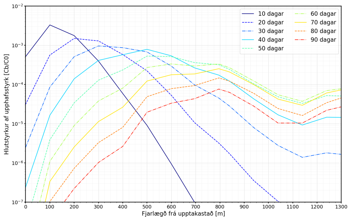
Mynd 64. Þróun hlutstyrks ferilefnis í atvikareikningum óhvarfgjarns ferilefnis frá upptakastað 1 í Heiðmörk ofan Gvendarbrunna og Jaðars eftir sniði 4. Sýndar er niðurstöður á völdum dögum eftir að ferilefni berst til grunnvatnsborðs og blandast strax í upphafsruðmmáli á upptakastað.
