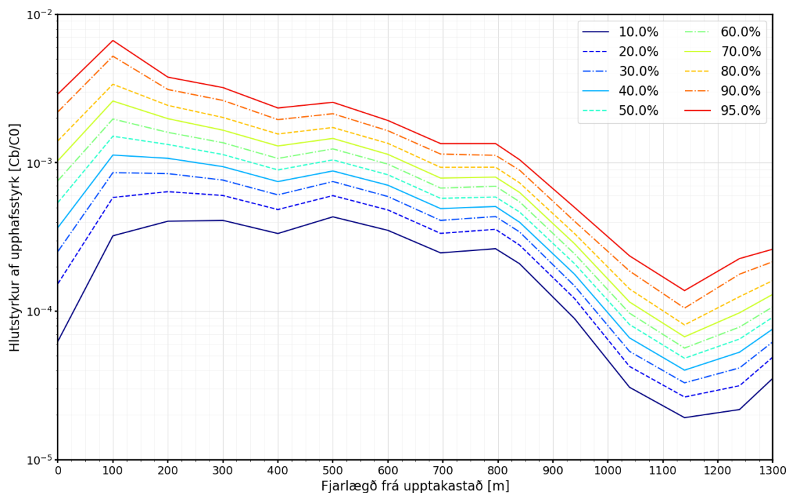
Mynd 65. Tíðnigreining á hlutstyrk ferilefnis í tíðnireikningum óhvarfgjarns ferilefnis frá upptakastað 1 í Heiðmörk ofan Gvendarbrunna og Jaðars eftir sniði 4. Sýndar er niðurstöður fyrir valið hlutfall keyrslutímans (60 ár), milli 10 og 95% tímans. Reikningarnir miða við fastan styrk ferilefnis í írennsli á upptakastað.
