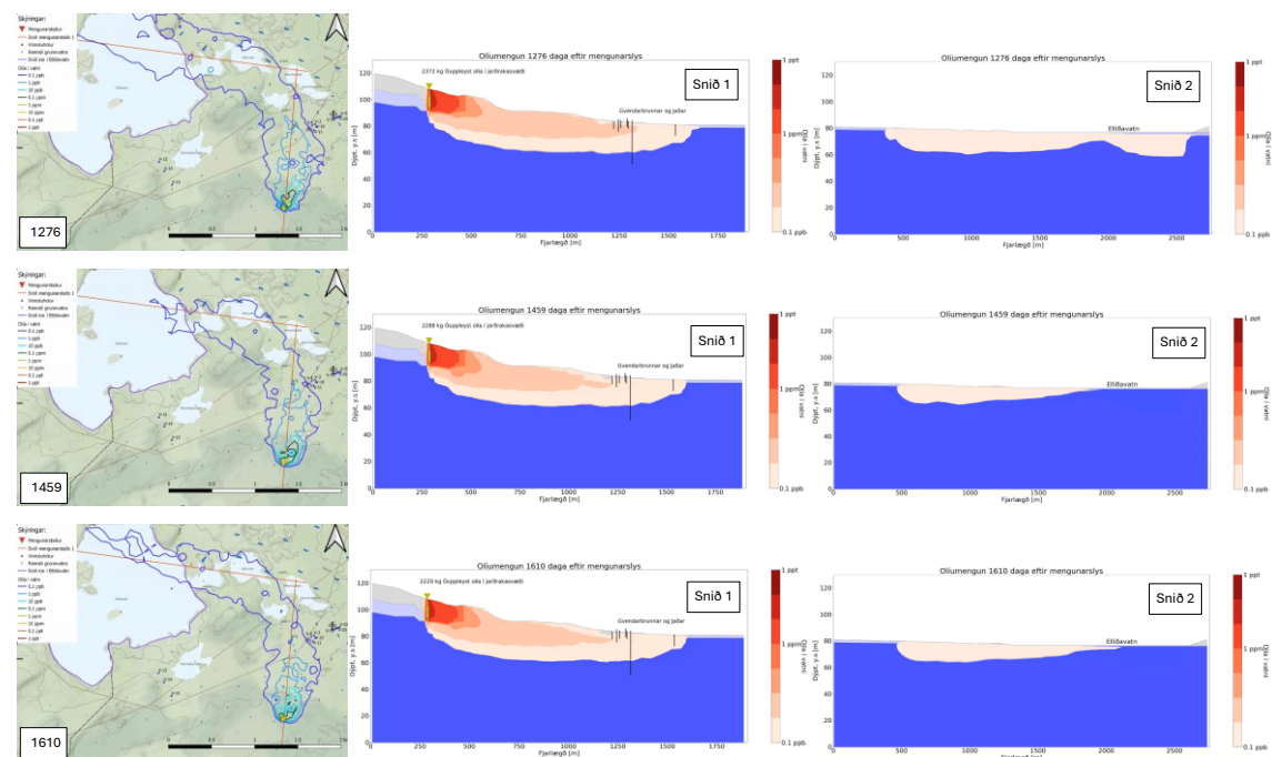
Mynd 43. Dreifing olíumengunar frá upptakastað 1, 1276, 1459 og 1610 dögum eftir 5000 L mengunarslys.
