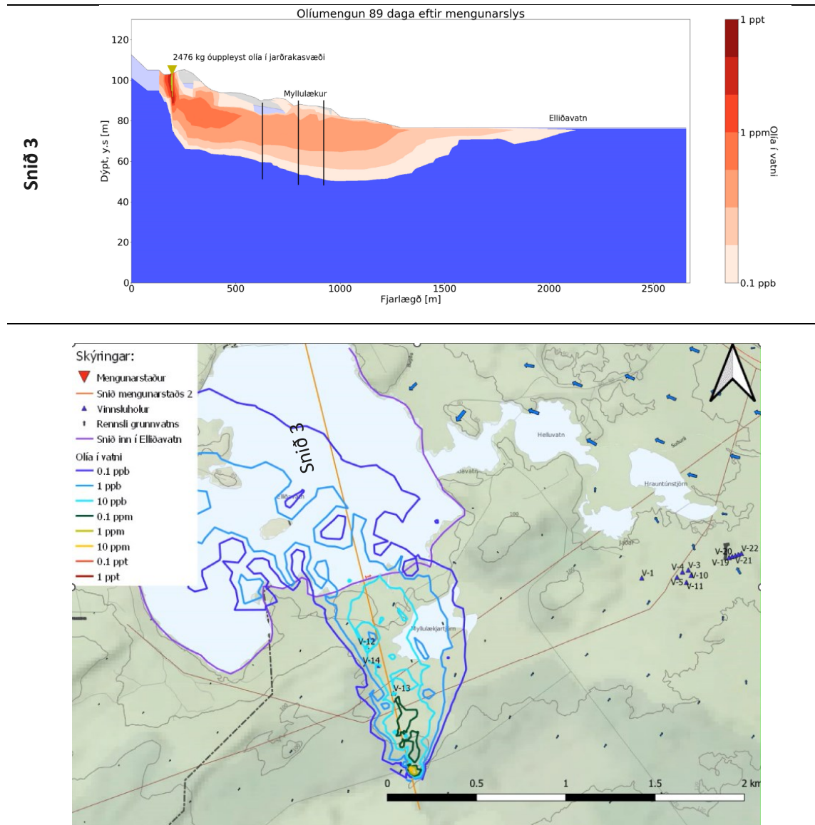
Mynd 46. Dreifing olíumengunar frá upptakastað 2, 89 dögum eftir mengunarslys þar sem 5000 L af olíu fara niður. Efst langsnið (Snið 3) eftir mengunarskíi frá upptakastað að vatnstökusvæðinu í Myllulæk. Neðst yfirlitsmynd yfir dreifingu mengunar frá upptakastað.
