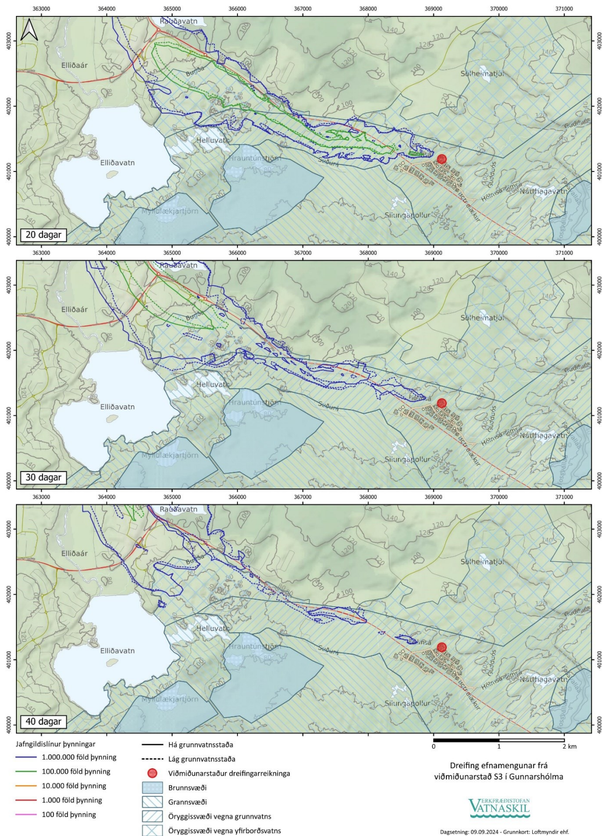
Mynd 16. Dreifing efnamengunar frá viðmiðunarstað S3 í Gunnarshólma eftir 20, 30 og 40 daga eftir að mengunarefni berst til grunnvatnsborðs.
