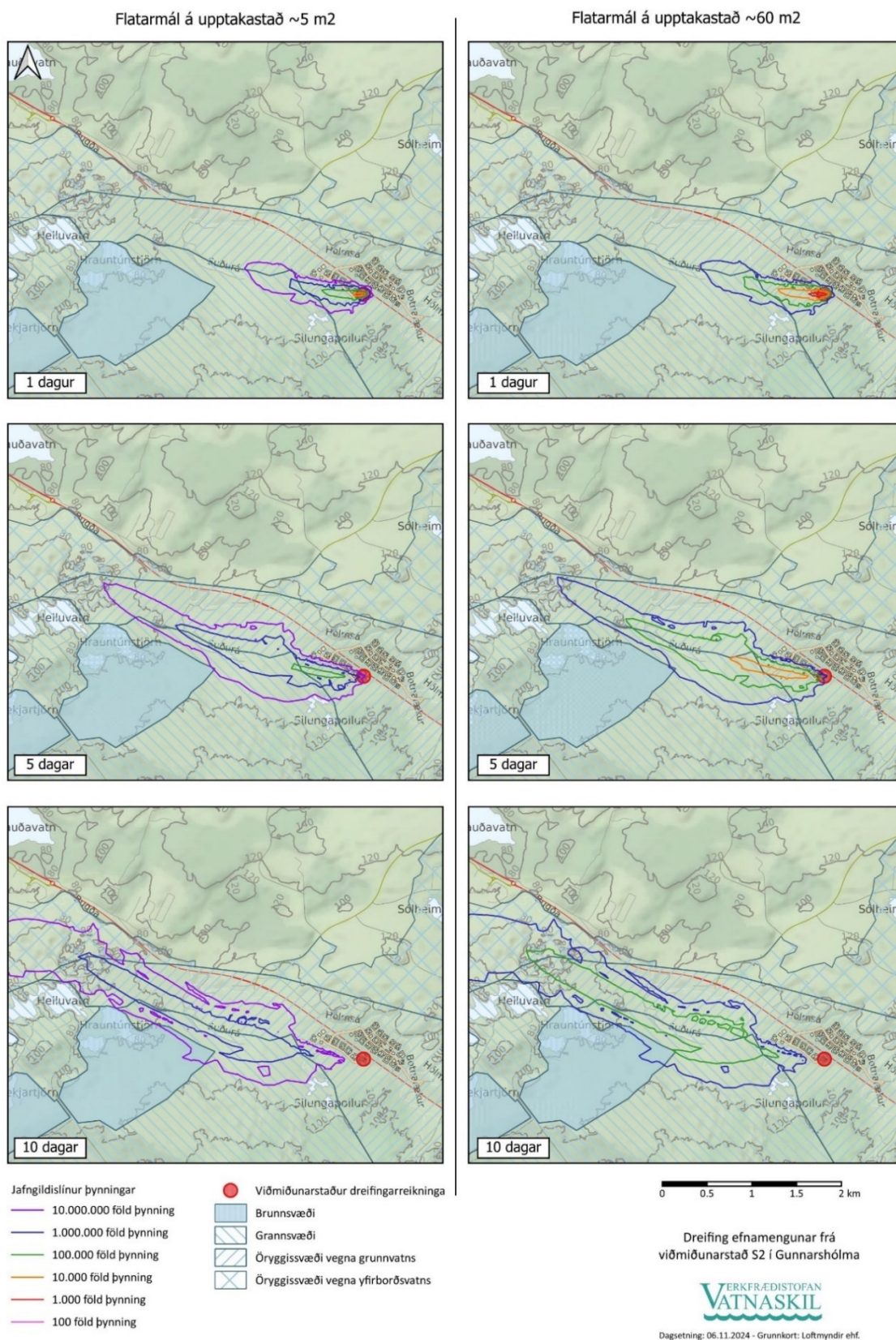
Mynd 26. Þróun dreifingar mengunar frá viðmiðunarstað S2 í Gunnarshólma, 1 til 10 daga eftir að mengunarefni berst til grunnvatns. Samanburður á niðurstöðum fyrir mismunandi stærð reiknins á upptakastað.
