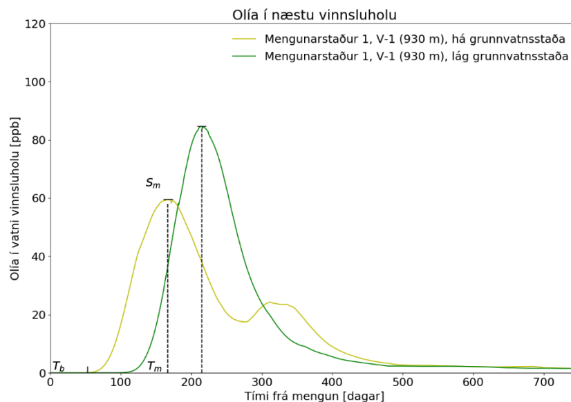
Mynd 59. Áhrif grunnvatnsstöðu á hæsta styrk olíu í vatni í V-1 eftir 5000 L mengunarslys við upptakastað 1.
