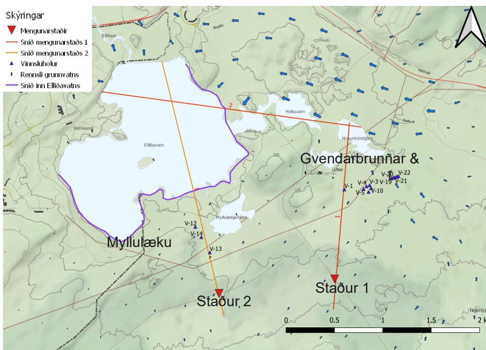
Mynd 27. Staðsetningar mengunarstaða, upptakastaðar 1 og upptakastaðar 2, lega sniða, vinnsluhola og grunnvatnsstraumar.
