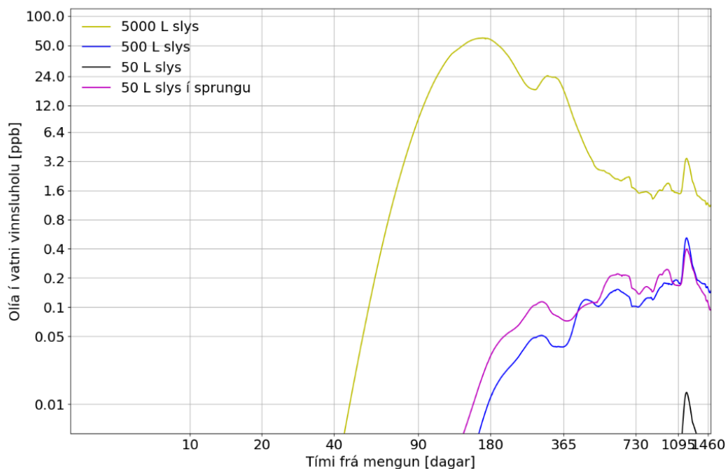
Mynd 60. Áhrif stærðar mengunarslyss á flutningstíma og styrk olíu í vinnsluholu V-1.
