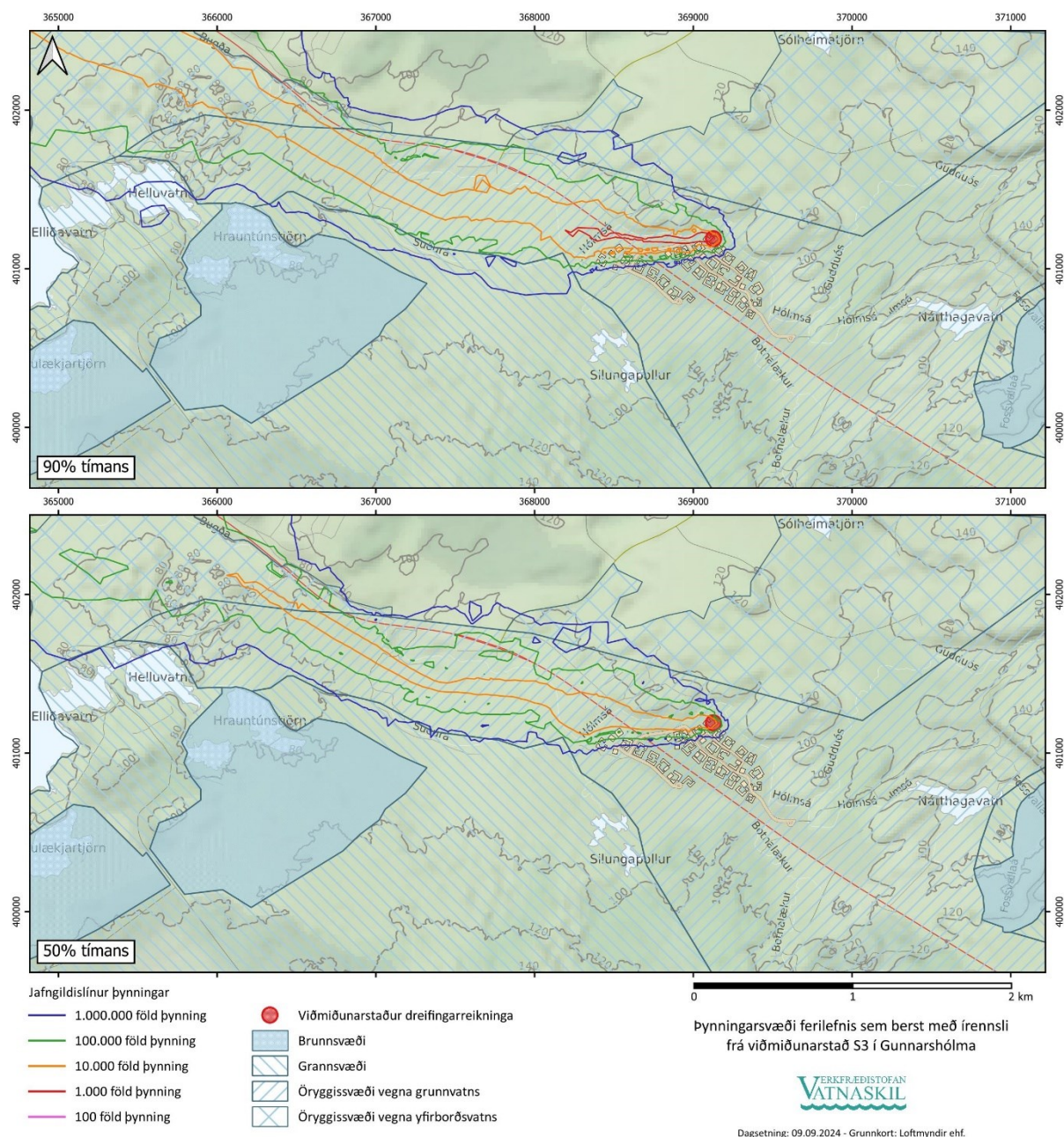
Mynd 23. Þynningargeta grunnvatnsleiðara 90% tímans (efri mynd) og 50% tímans (neðri mynd) miðað við fastan styrk mengunar í írennsli á viðmiðunarstað S3.
