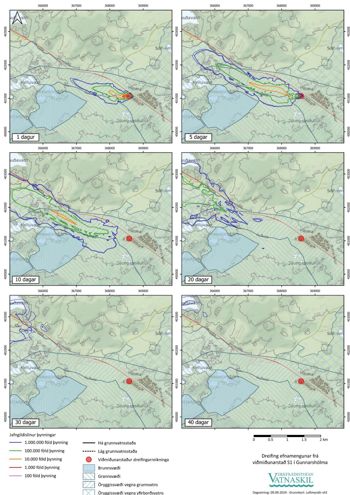
Mynd 5. Þróun dreifingu mengunar frá viðmiðunarstað S1 í Gunnarshólma, 1 til 40 daga eftir að mengunarefni berst til grunnvatns.
