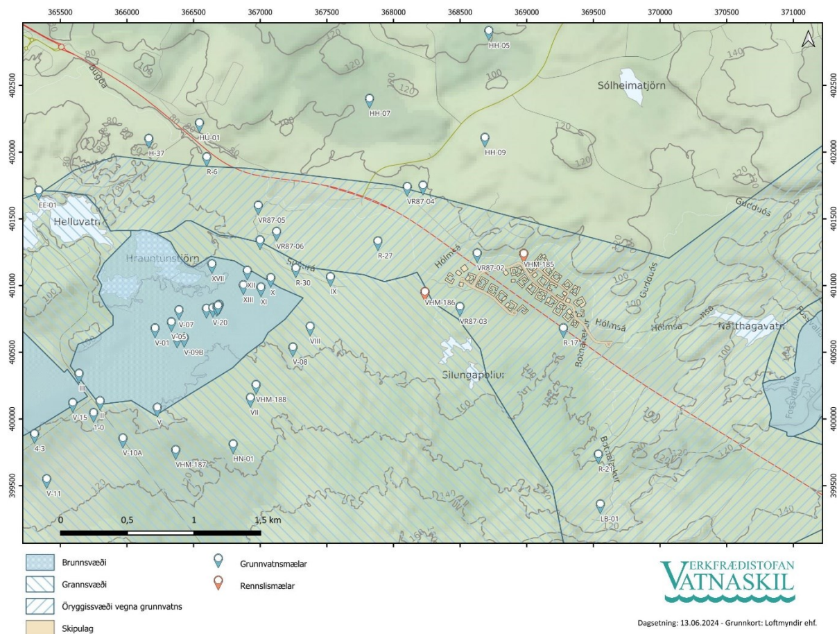
Mynd 1. Yfirlitskort af skipulagssvæði og nærliggjandi svæði ásamt staðsetningum grunnvatns- og rennslismæla.
