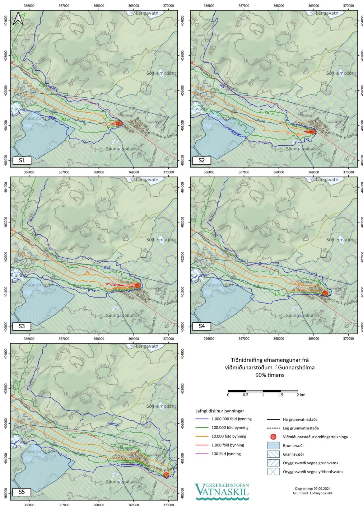
Mynd 8. Þynningargeta grunnvatnsleiðara 90% tímans miðað við fastan styrk mengunar í rennsli á viðmiðunarstöðum S1 til S5.
