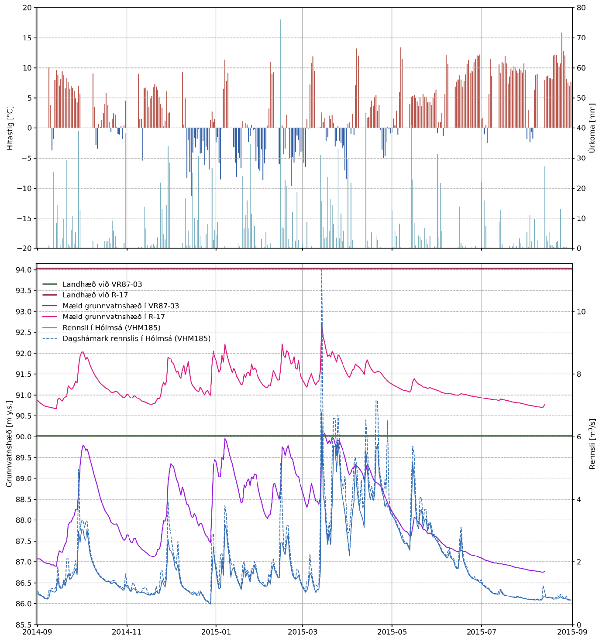
Mynd 3. Efri mynd; reiknuð dagsúrkoma (ljósblá lína) og hitastig (rauð og blá lína). Neðri mynd; mæld grunnvatnshæð í holu VR87-03 og R-17 ásamt mældu meðal- og hámarksdagsrennsli í Hólmsá fyrir vatnsárið 2014. Landhæð við VR87-03 er rétt rúmir 90 m y.s. en landhæð við R-17 er rétt rúmir 94 m y.s.
