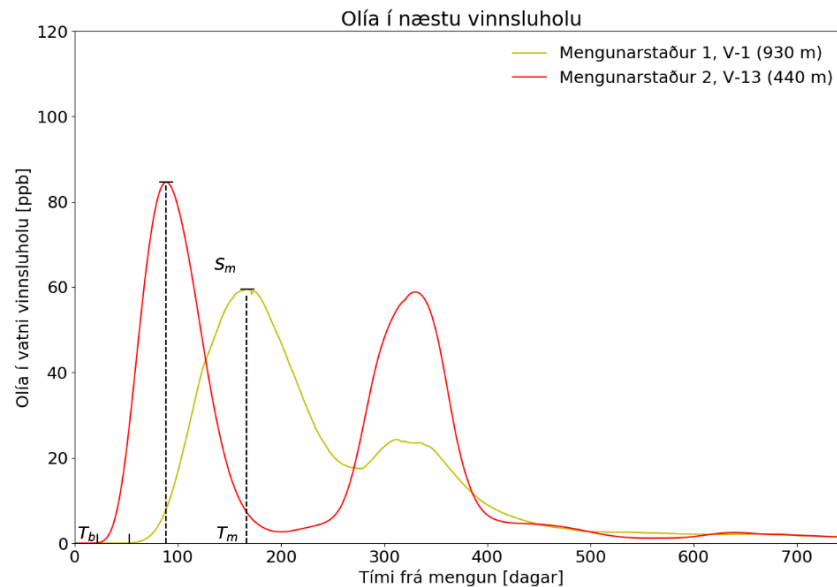
Mynd 58. Samanburður á styrk olíu í næstu vinnsluholu frá upptakastað mengunar og þróun með tíma frá mengunarslysi. T_m er tíminn sem hæsti styrkur olíu S_m reiknast í næstu vinnsluholu.
