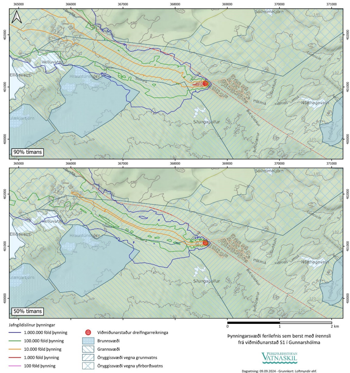
Mynd 21. Þýnningargeta grunnvatnsleiðara 90% tímans (efri mynd) og 50% tímans (neðri mynd) miðað við fastan styrk mengunar í írennsli á viðmiðunarstað S1.
