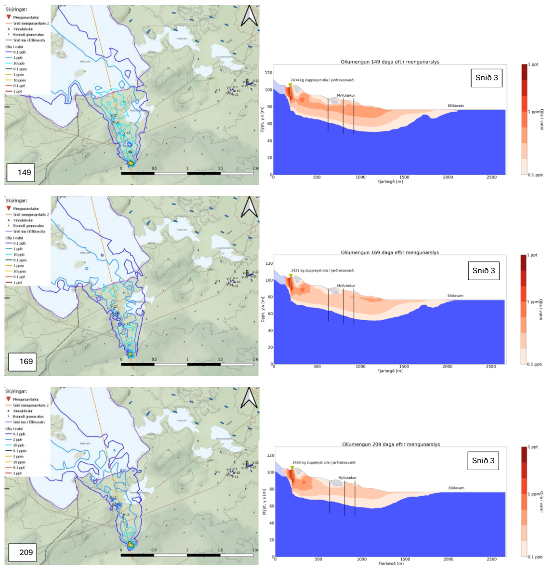
Mynd 51. Dreifing olíumengunar frá upptakastað 2, 149, 169 og 209 dögum eftir 5000 L mengunarslys.
