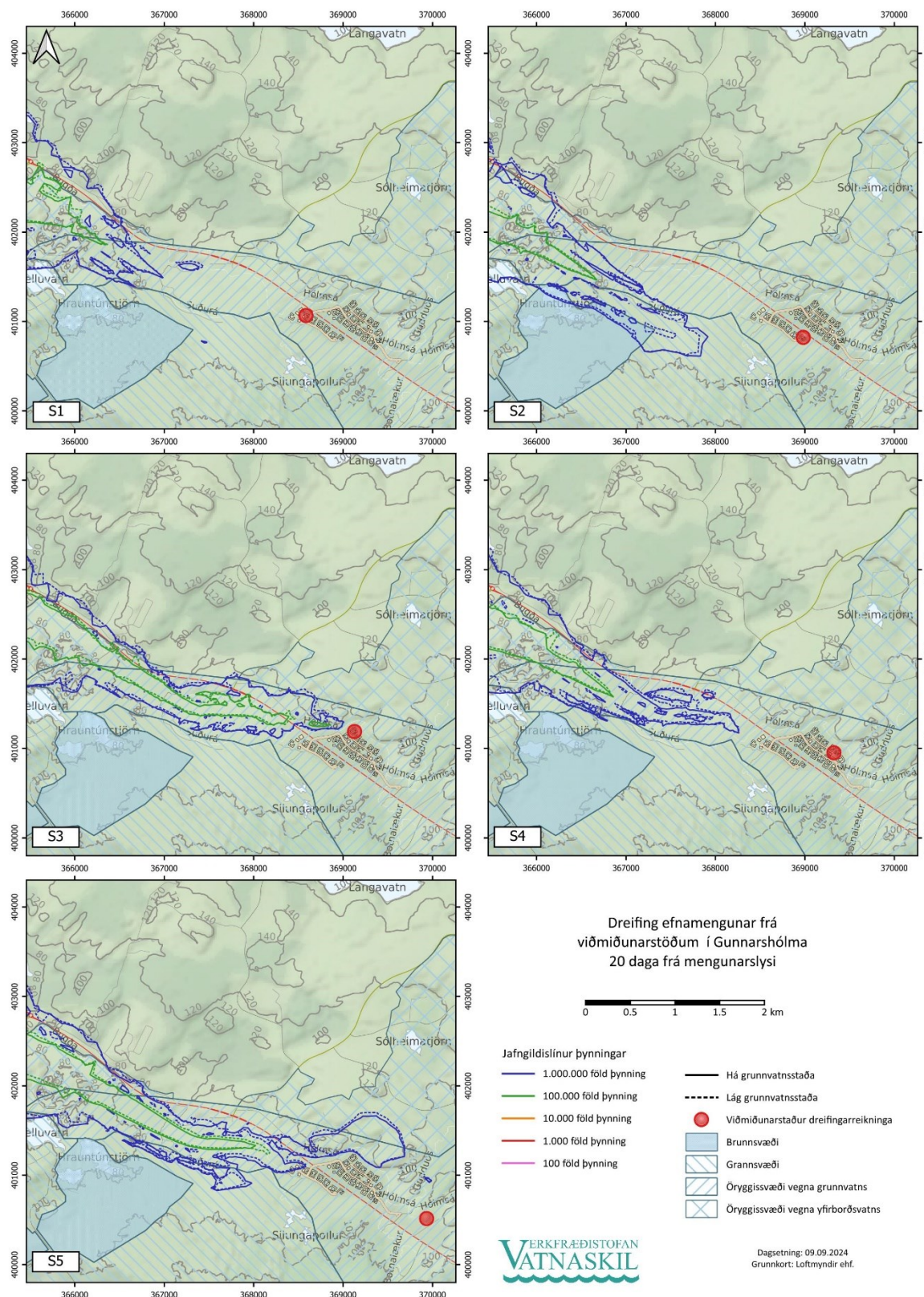
Mynd 7. Samanburður dreifingu mengunar frá viðmiðunarstöðum S1 til S5 í Gunnarshólma, 20 dögum eftir að mengunarefni berst til grunnvatns.
