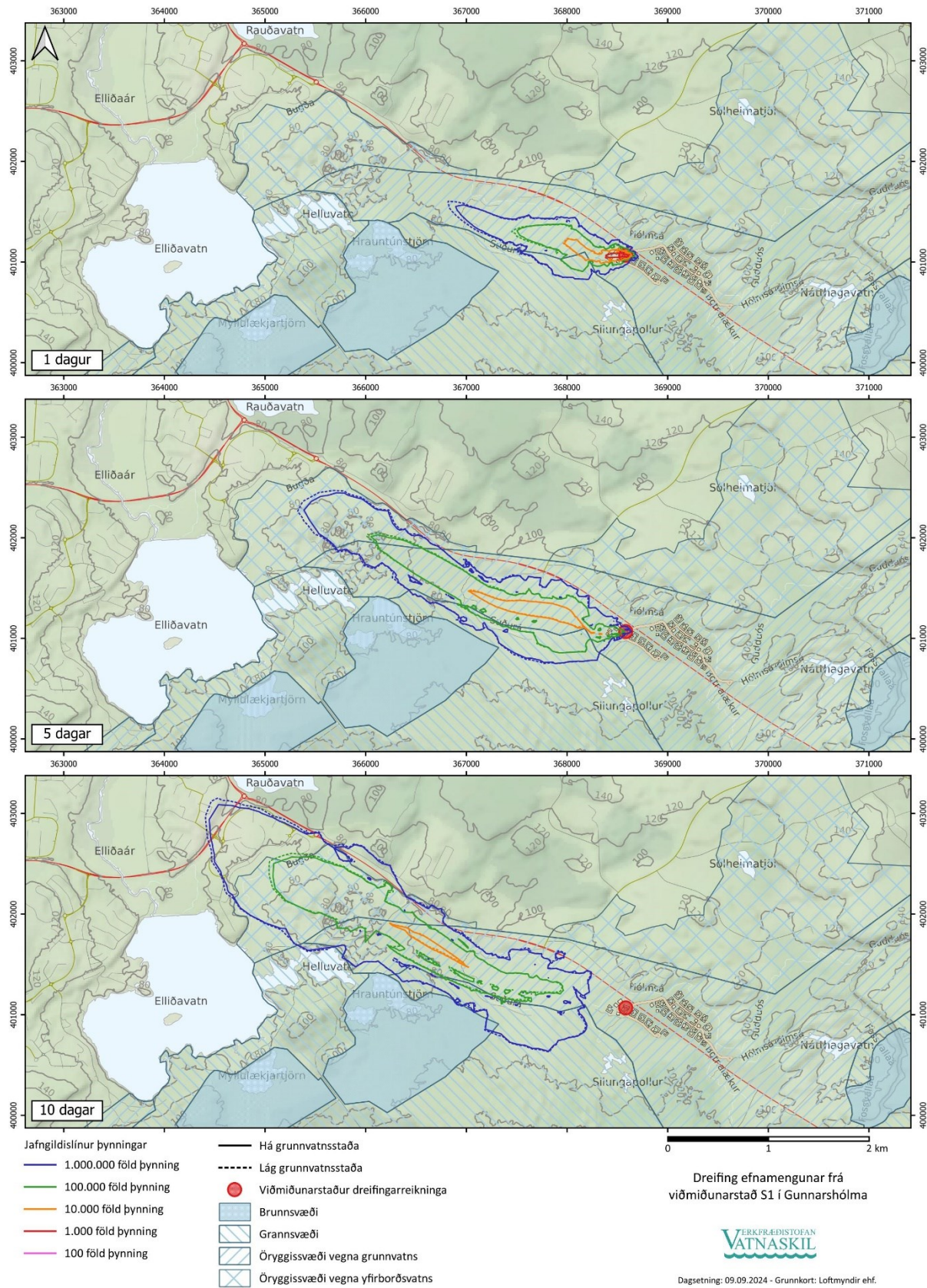
Mynd 11. Dreifing efnamengunar frá viðmiðunarstað S1 í Gunnarshólma eftir 1 dag, 5 og 10 daga eftir að mengunarefni berst til grunnvatnsborðs.
