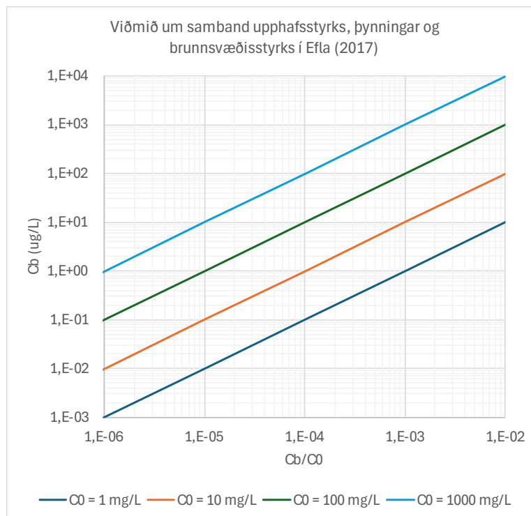
Mynd 66. Viðmið notað í Efla (2017) varðandi samband upphafsstyrks á slyssað, þynningar mengunarefnis í grunnvatnsleiðara og styrks mengunarefnis á brunnsvæði.
