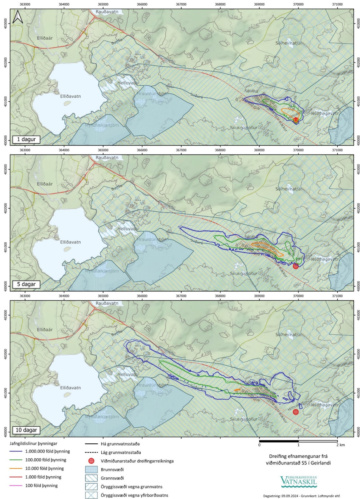
Mynd 19. Dreifing efnamengunar frá viðmiðunarstað S5 í Geirlandi eftir 1 dag, 5 og 10 daga eftir að mengunarefni berst til grunnvatnsborðs.
