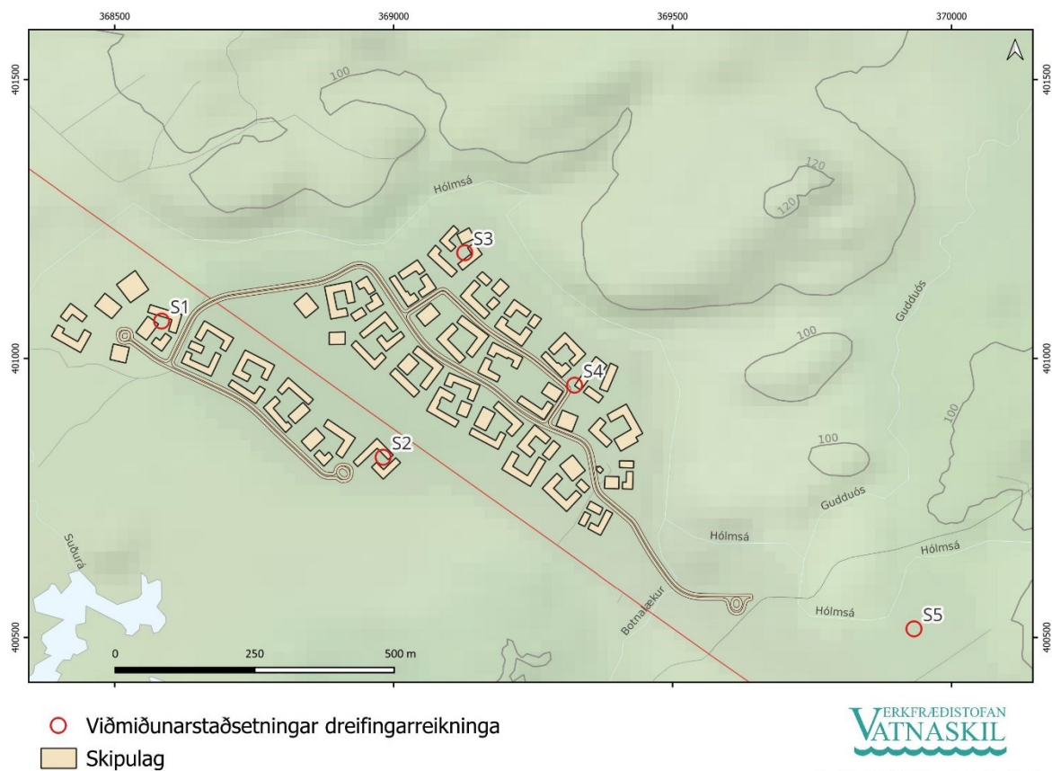
Mynd 4. Yfirlitsmynd skipulagssvæðis og viðmiðunarstaðsetninga dreifingarreikninga.
