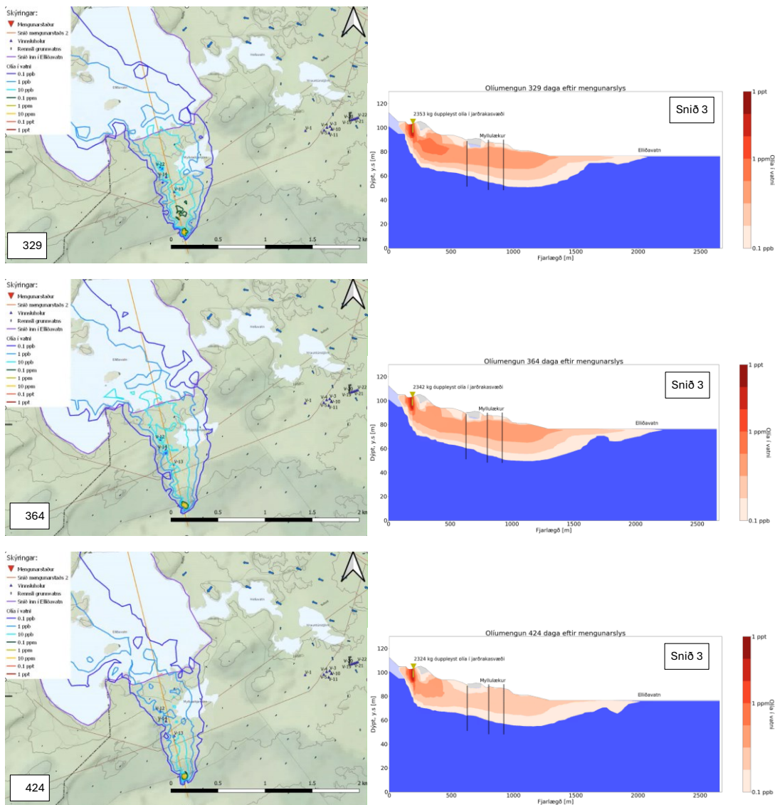
Mynd 53. Dreifing olíumengunar frá upptakastað 2, 329, 364 og 424 dögum eftir 5000 L mengunarslys.
