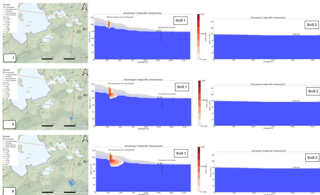
Mynd 34. Dreifing olíumengunar frá upptakastað 1, 1, 4 og 9 dögum eftir 5000 L mengunarslys.
