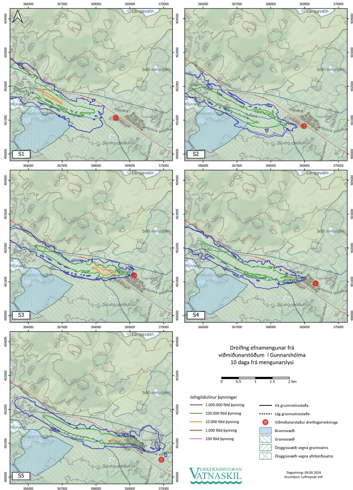
Mynd 6. Samanburður dreifingu mengunar frá viðmiðunarstöðum S1 til S5 í Gunnarshólma, 10 dögum eftir að mengunarefni berst til grunnvatns.
