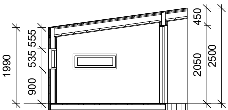
A-A 1 : 100
