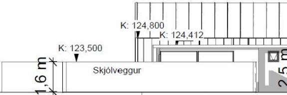
Skýringarmynd: Götumynd suðurhlíð eftir breytingar í mkv. 1:200
