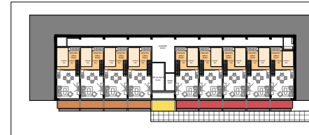
Grunnmynd millipalls 1:1000
