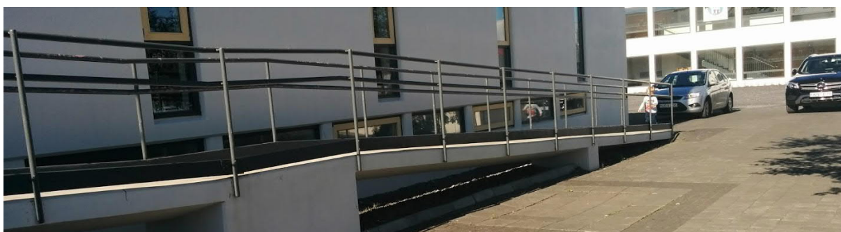
Mynd 4-48 Skábraut við Álfaneslaug. Kantur er við hlið skábrautarinnar, hvíldarpallar og handlistar í 0,7 og 0,9 m hæð eru við brautina (Mynd: Berglind Hallgrímsdóttir).
