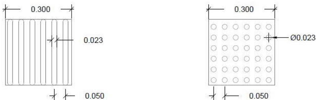
Mynd 4-13 Hellur ætlaðar til að mynda sértækar leiðarlínur, vinstra megin er stefnueining og áherslu- og varúðareining hægra megin (Mynd: Áslaug Katrín Aðalsteinsdóttir).
