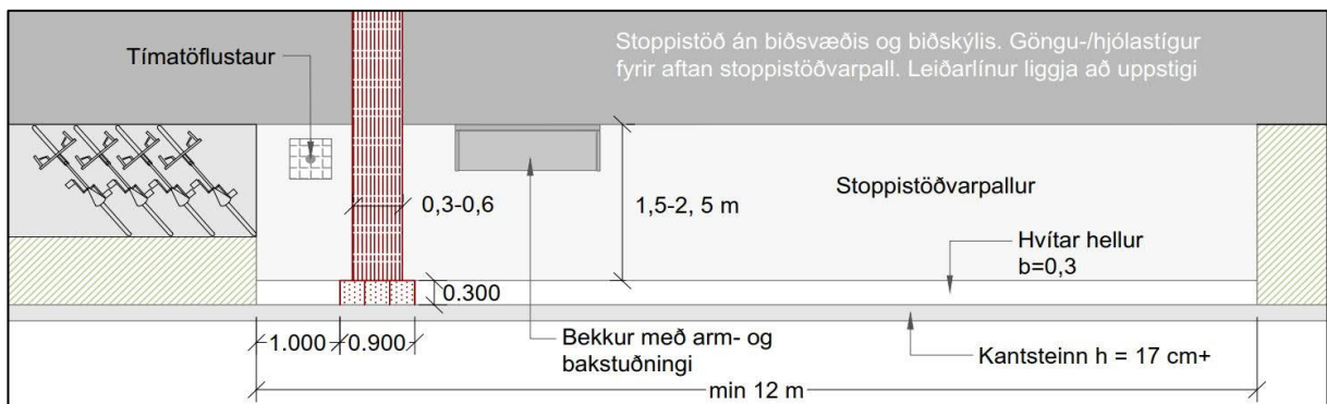
Mynd 5-5 Mynd sýnir notkun á leiðarlínunum við stoppistöð án biðskýlis og sérstaks biðsvæðis. Göngu- og hjólastígur liggur utan við stoppistöðvarpall. Leiðarlínur fanga væntanlega farþega frá göngustíg og leiða þá að uppstigi í vagn. Hjólagrindur eru staðsettar utan við stoppistöðvarpall, fjær akstursstefnu (Mynd: Áslaug Katrín Aðalsteinsdóttir).
