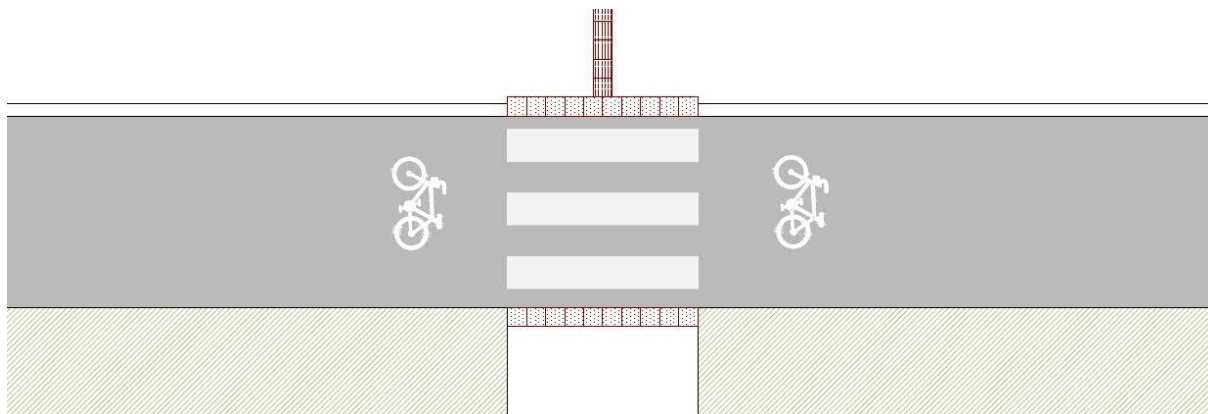
Mynd 4-26 Útfærsla á sértækum leiðarlínum þar sem göngustígur þverar hjólastíg. Mikilvægt er að vara hjólandi vegfarendur við þverun gangandi vegfarenda í tíma, til dæmis með skiltum eða yfirborðsmerkingum (Mynd: Áslaug Katrín Aðalsteinsdóttir).
