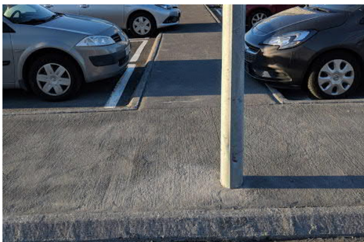
Mynd 4-34 Gönguleið frá bílastæði að inngangi verslunar. Gönguleiðin er nægilega breið en niðurtekt vantar við enda hennar. Ljósastaur er í gangvegnum, staurinn hefði þurft að færa úr miðju gönguleiðar og setja annað yfirborðsefni umhverfis hann (Mynd: Berglind Hallgrímsdóttir).
