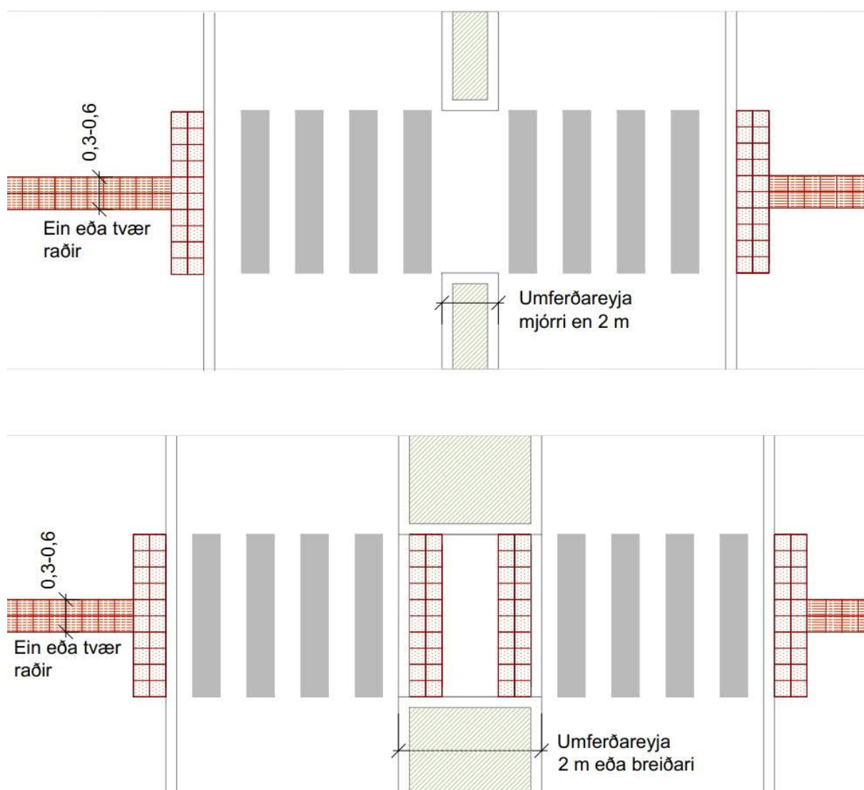
Mynd 4-28 Útfærsla á leiðarlínum á miðeyju við gangbrautir, án merkinga þegar miðeyja er mjórri en 2 m (efri mynd) og með merkingum á umferðareyju þegar miðeyjan er 2 m eða breiðari (neðri mynd) (Mynd: Áslaug Katrín Aðalsteinsdóttir).
