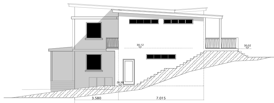
Útlit Vestur
