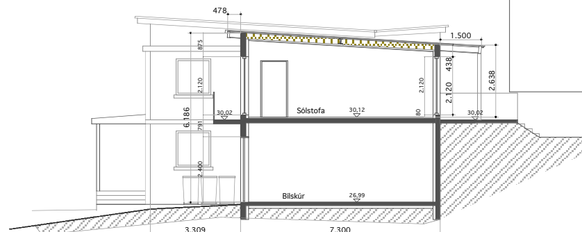
Sneiðing A - A
