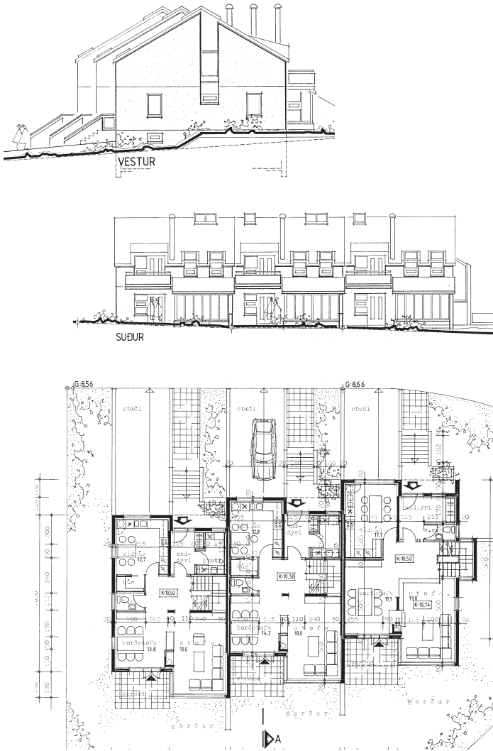
Mynd 154: Grunnmyndir og áskýndir
