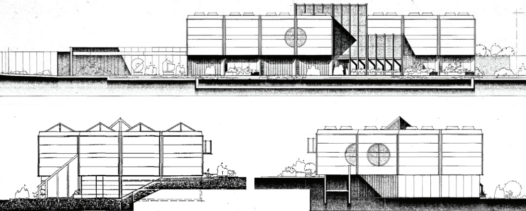
Mynd 151: Ásýndir. Aðaluppdráttur fyrir Gerðarsafn, 1986.
