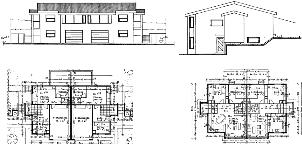
Mynd 155: Grunnmyndir og ásyndir
