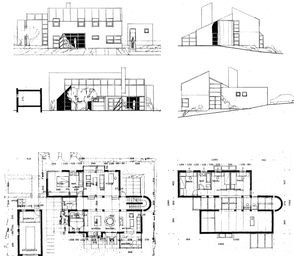
Mynd 157: Grunnmyndir og ásýndir
