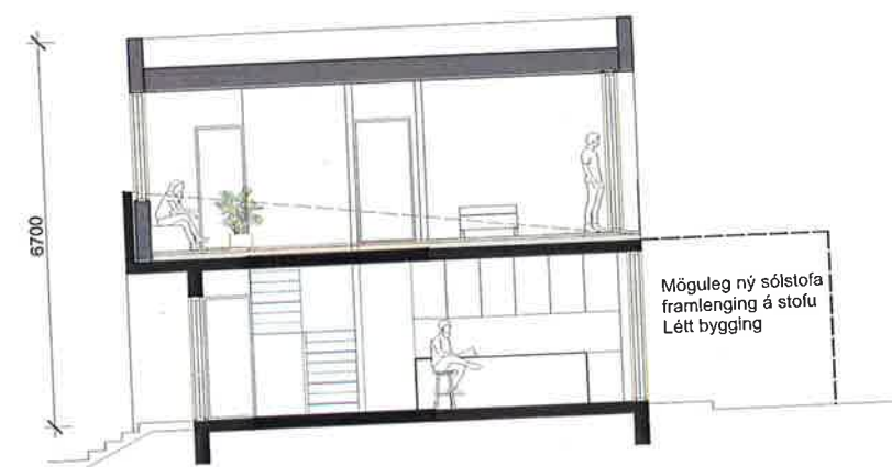
Sneiðing A mvk. 1:100 Sjá staðsetningu sniðpílu á afstöðumynd
