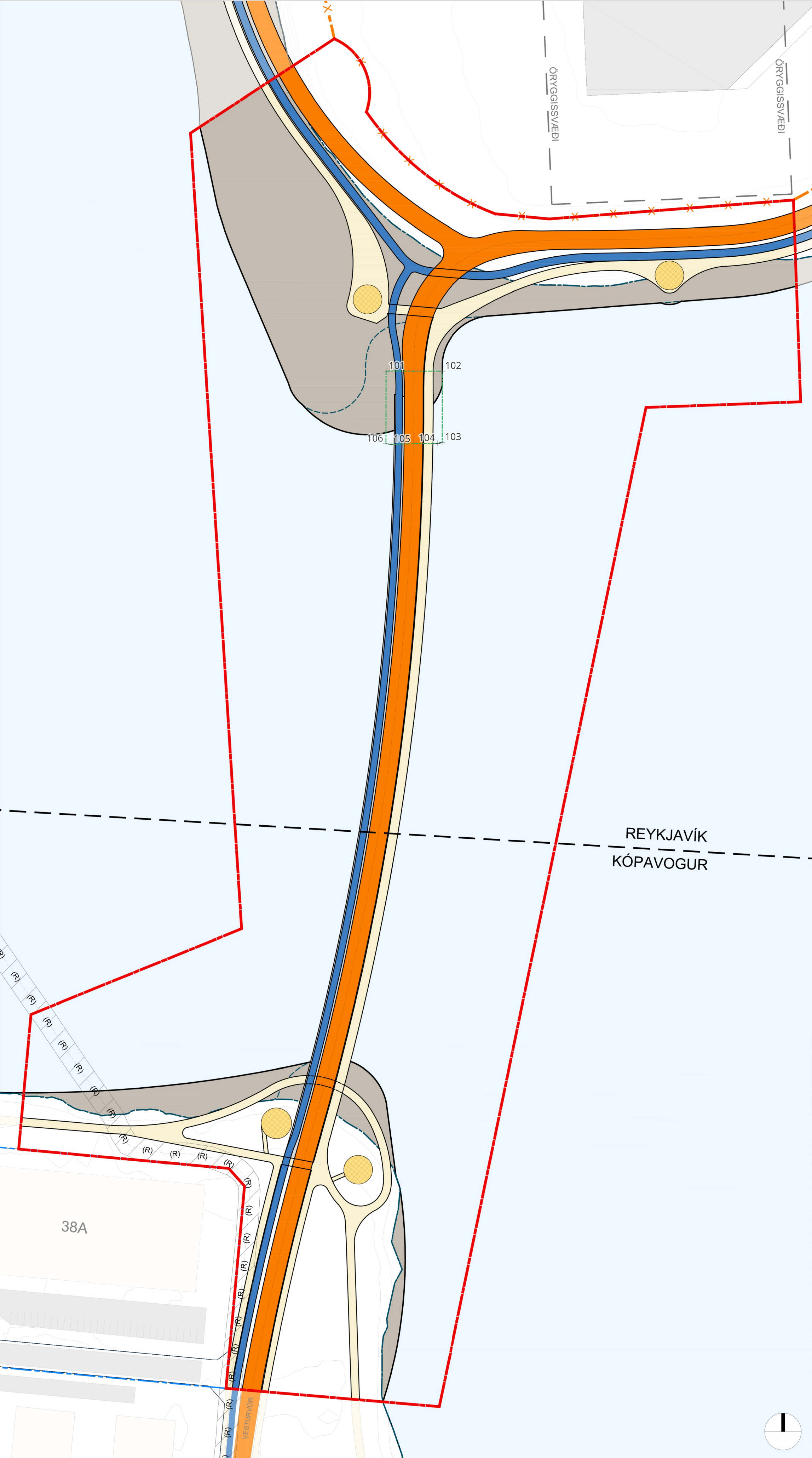
Gildandi deiliskipulag, samþykkt í umhverfis- og skipulagsráði Reykjavíkurborgar 20. mars 2024 og bæjarstjórn Kópavogsbæjar 13. febrúar 2024. Sínd er áorðin breyting vegna lóðar við brúarstöpul Reykjavíkurmegin. Mælikvarði 1:1.000
